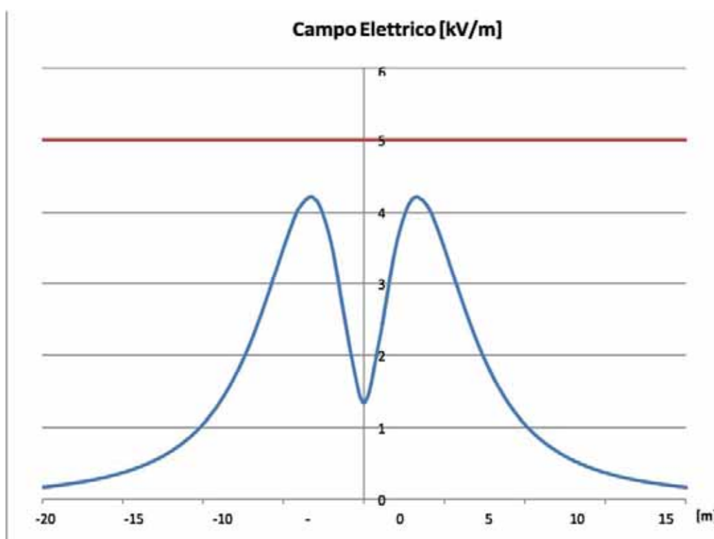
Figura 10: Campo elettrico al suolo generato dal sistemi sbarre a 150 kV
