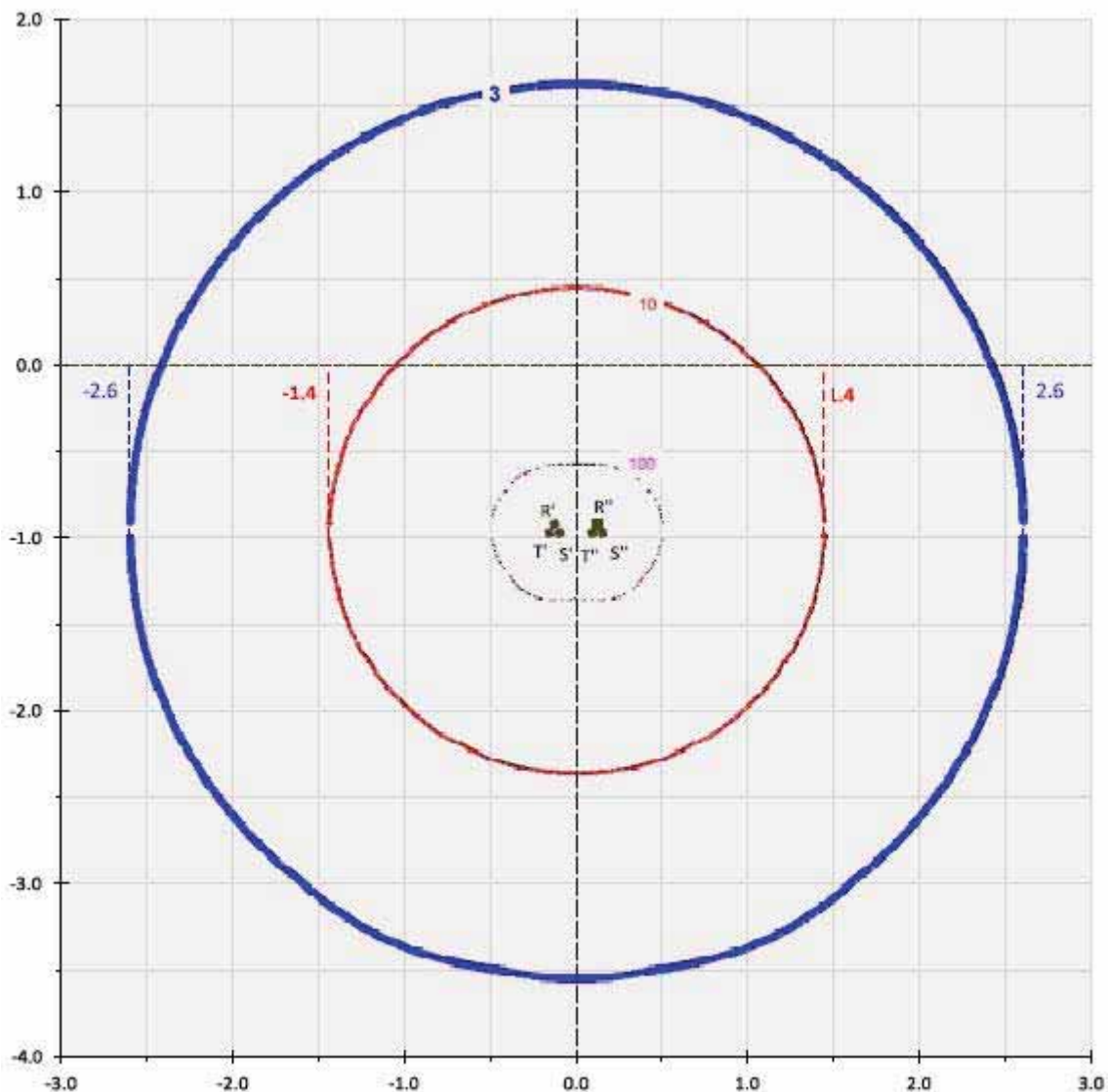
Figura 9: Curve di equilivello per il campo di induzione magnetica generato da una linea MT posata a trifoglio ( I_{max}=710^\circ ; formazione(3x1x240))
