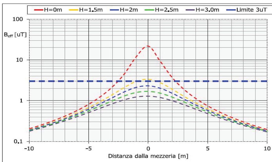
Figura 7: Andamento dell'induzione magnetica prodotta dalla linea in cavo per la massima corrente del cavo. Si può osservare come nel caso peggiore il valore di 3 \mu T è raggiunto a circa 2,6 m dall'asse del cavidotto.
