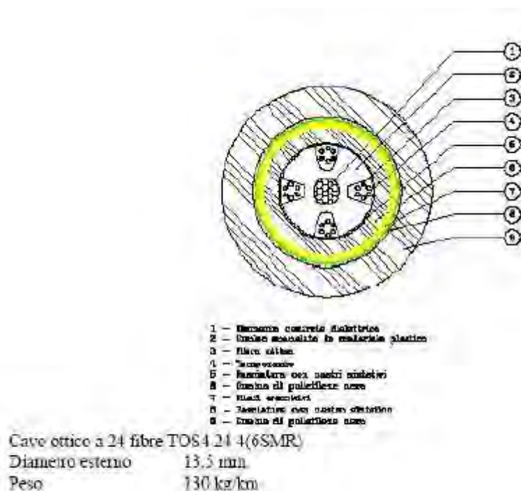
Schema cavo fibra ottica (F.O.)
