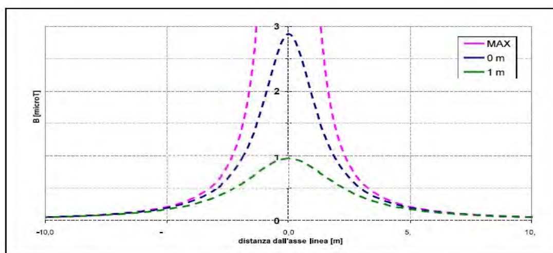
Andamento dell'induzione magnetica prodotta dalla linea in cavo
