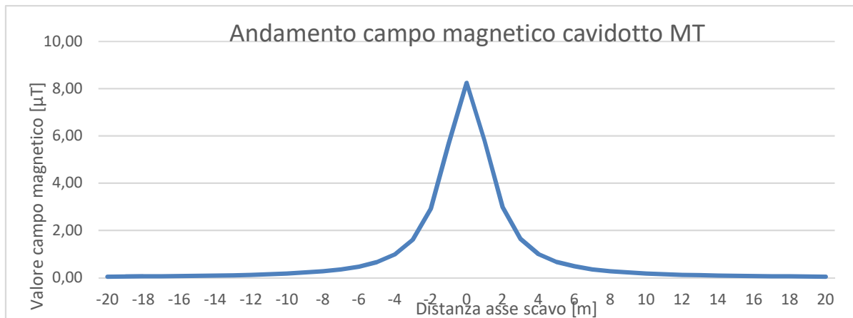
Figura: Induzione magnetica rispetto all'asse del cavidotto
