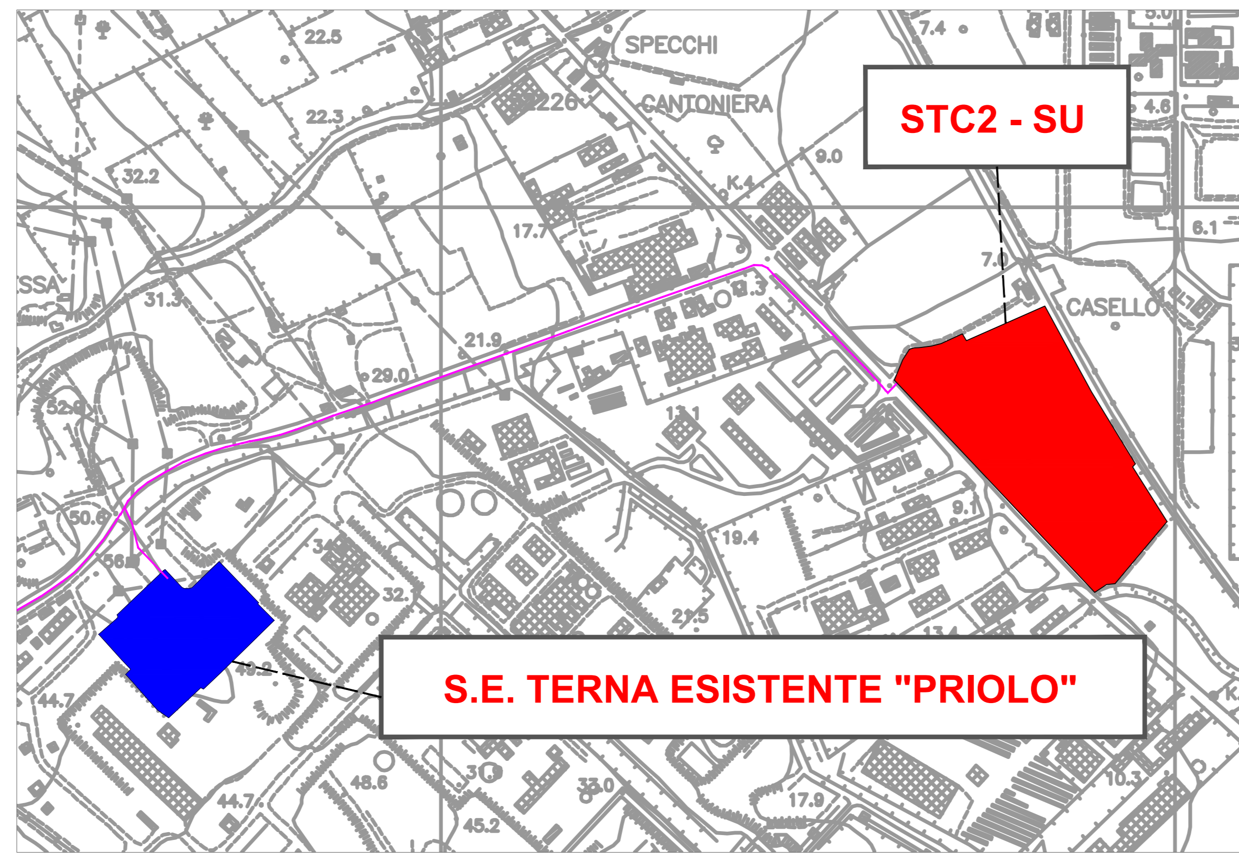
INQUADRAMENTO DI DETTAGLIO S.E. E S.U. SU CTR Scala 1:5.000
