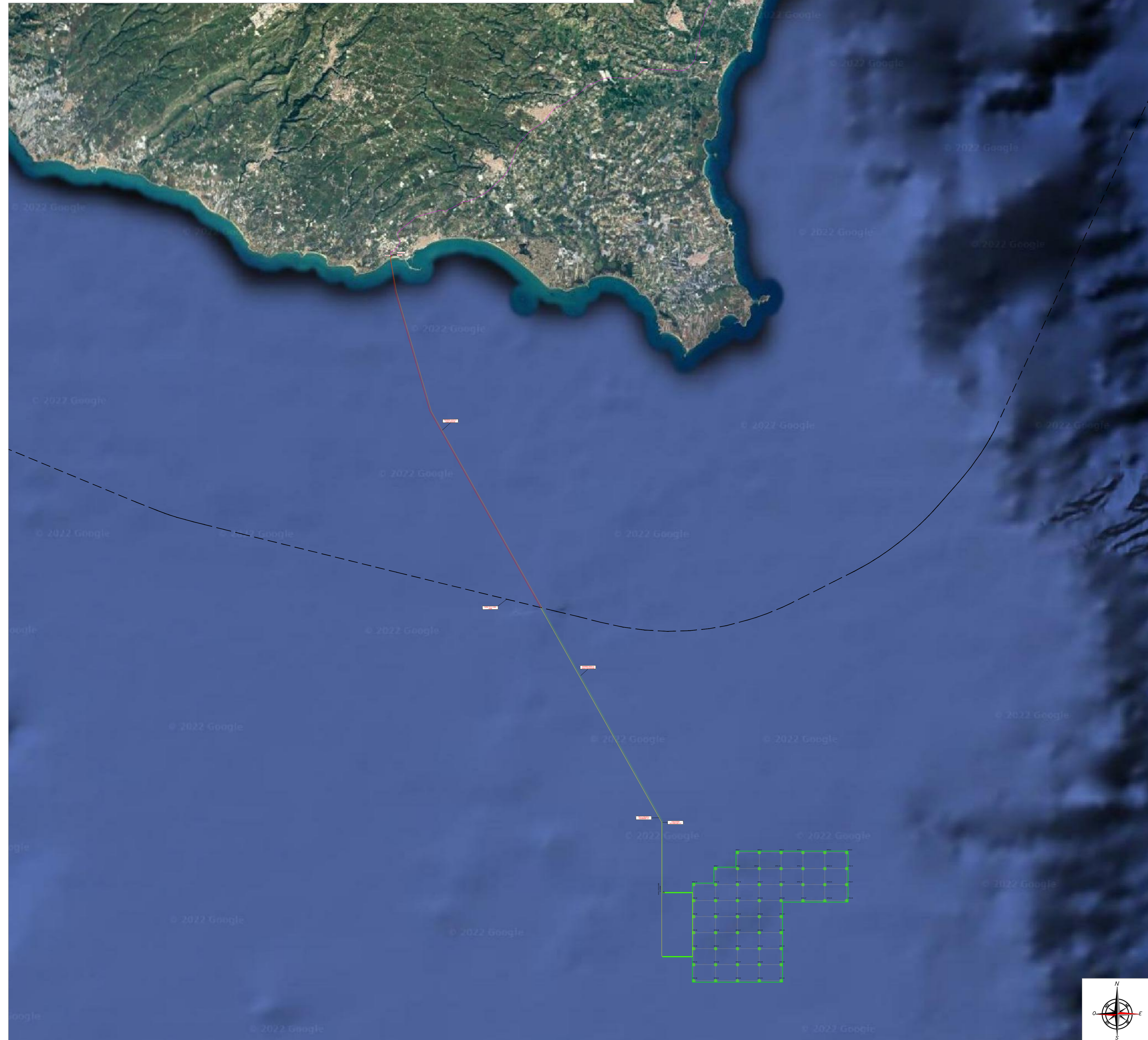
INQUADRAMENTO GENERALE PARCO EOLICO Scala 1:150.000
