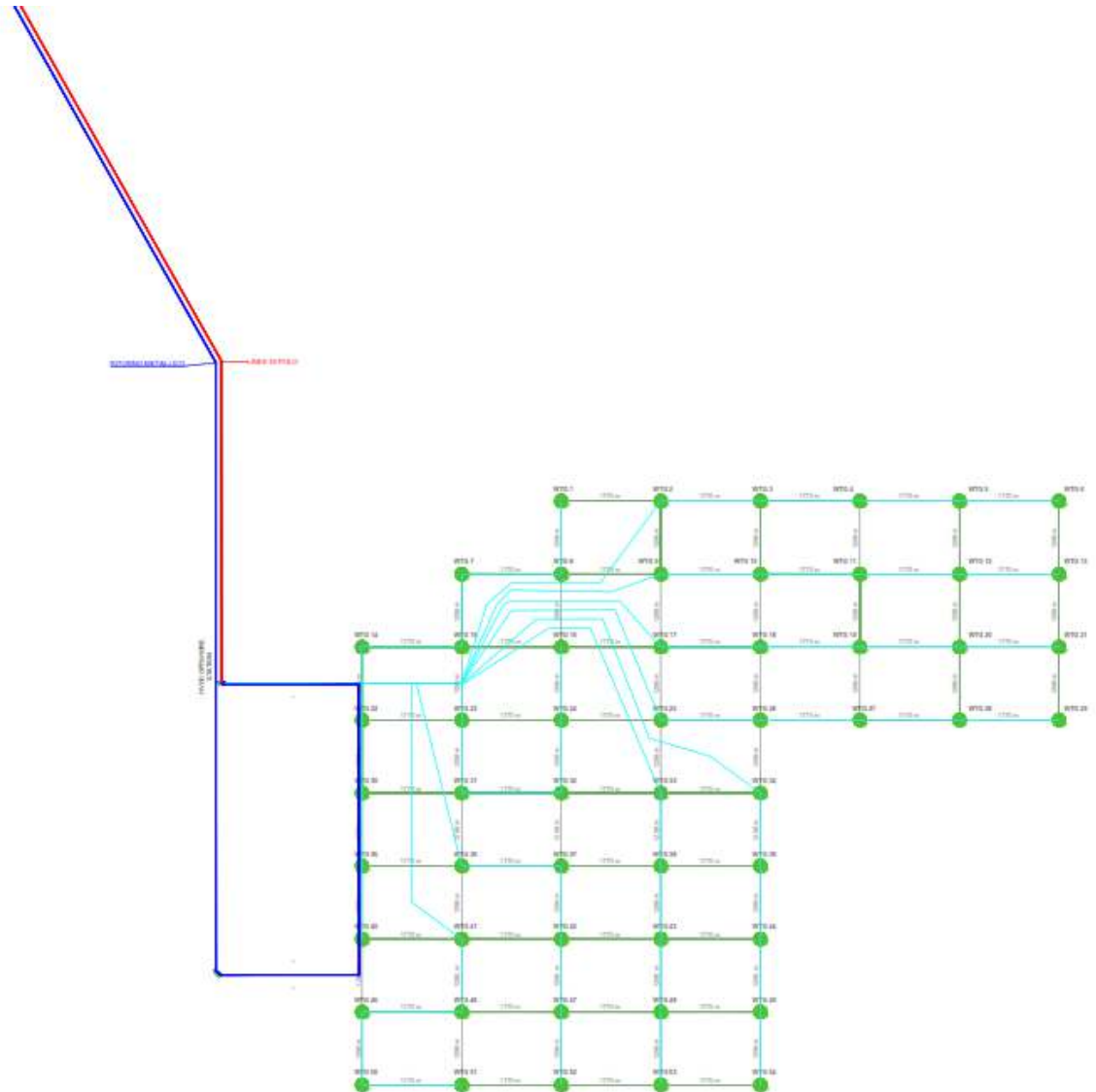
Figura 3 - Schema elettrico di collegamento del Parco Eolico: le WTG (cerchi verdi), le linee di stringa a 66 kV (linee ciano), le linee di polo (linea rosso) e la linea di ritorno metallico (blu)
