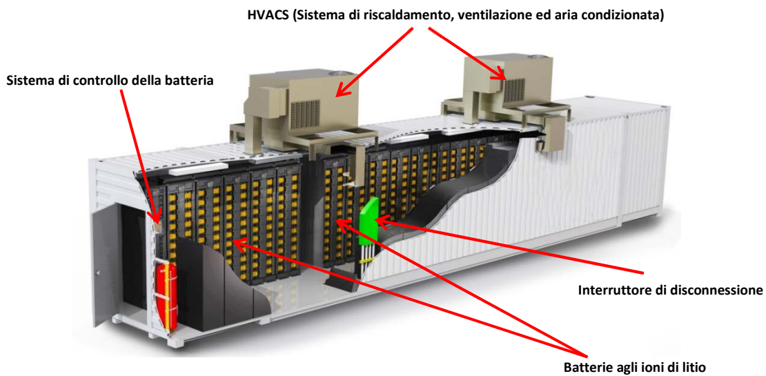
Figura 19 BESS - Container tipo
