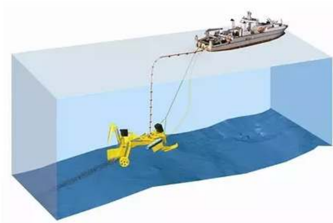
Figura 9 - Esempio di nave posa cavo
