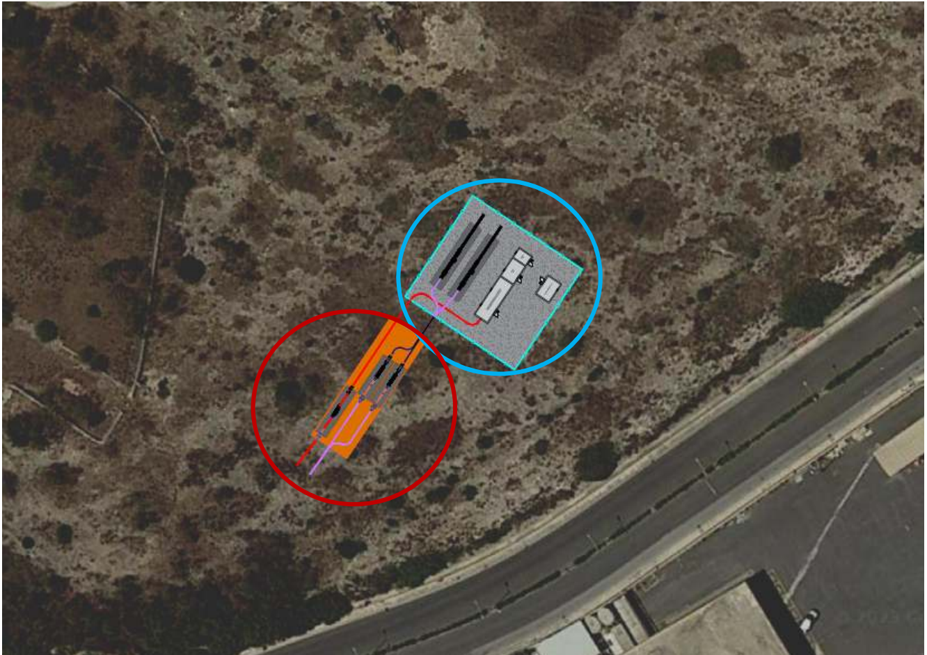
Figura 11 - Stazione di sezionamento (cerchio azzurro) e fossa giunti (cerchio rosso)
