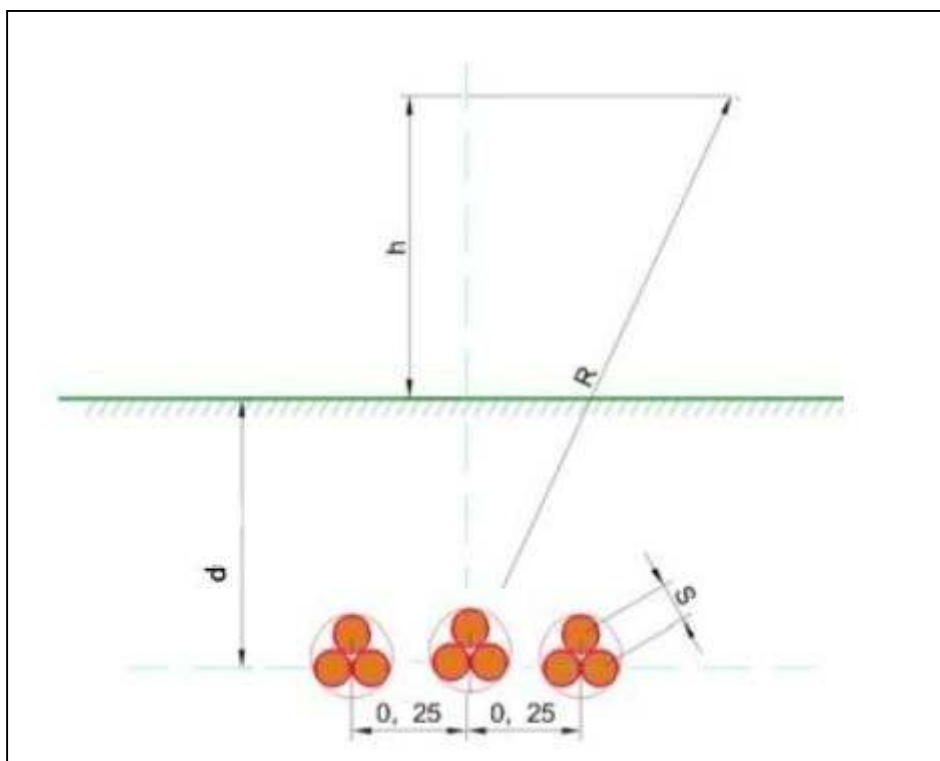
Figura 21 sistema di tre terne a trifoglio
