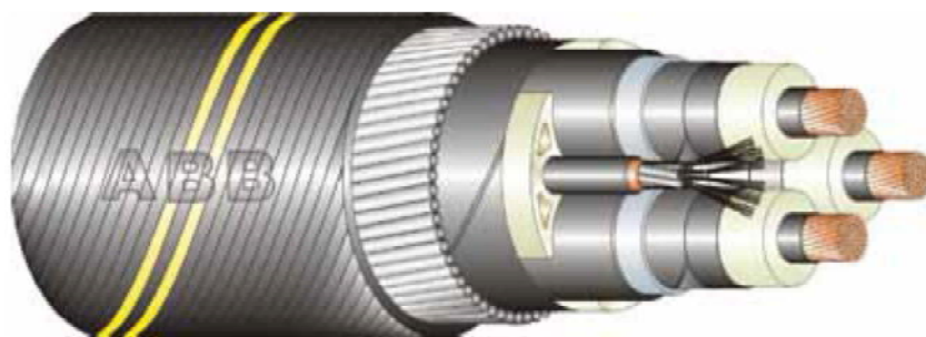
Figura 8 - Cavo sottomarino 66 kV con conduttori di rame
