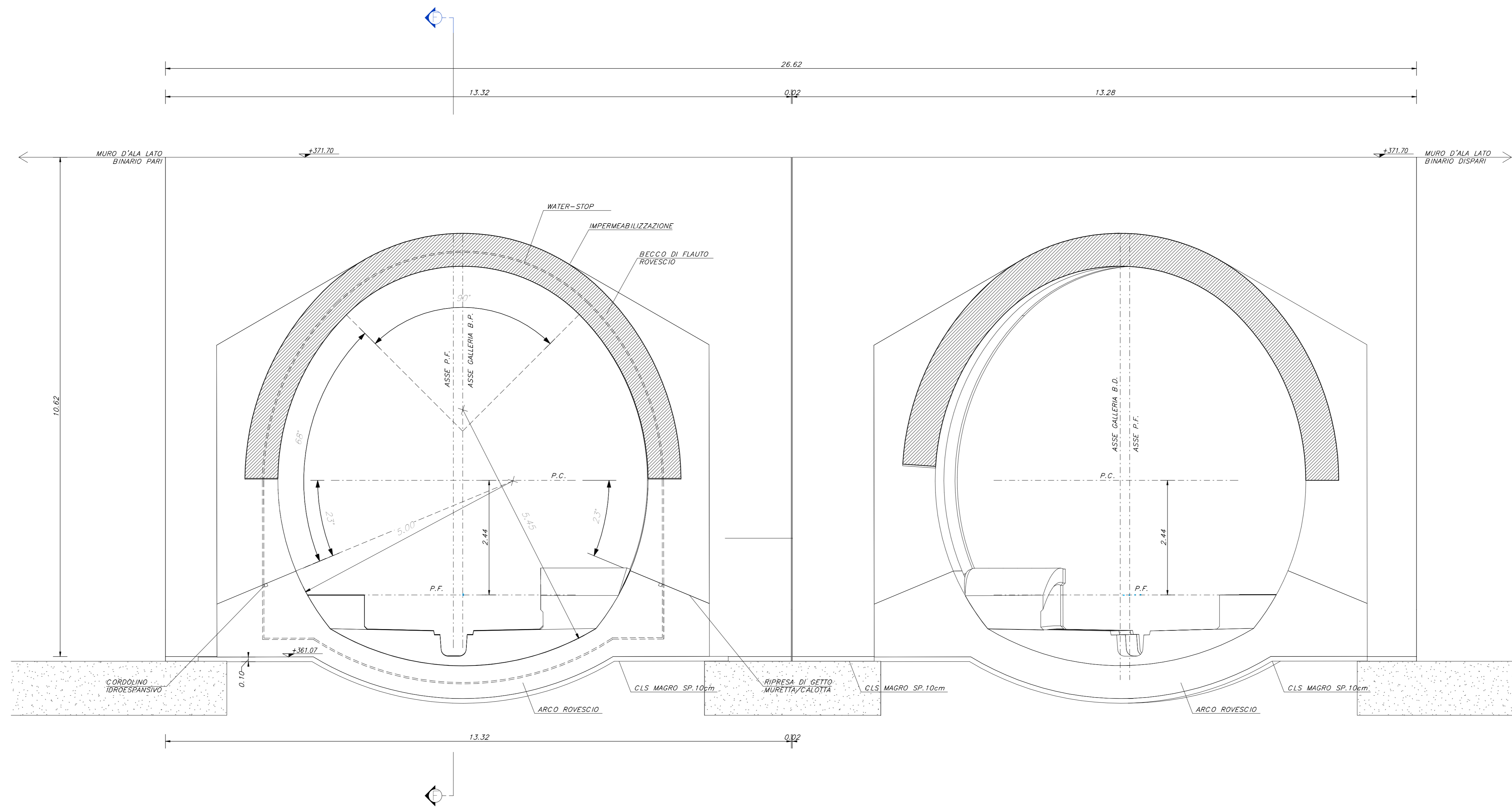
PROSPETTO GALLERIA ARTIFICIALE SCALA 1:50
