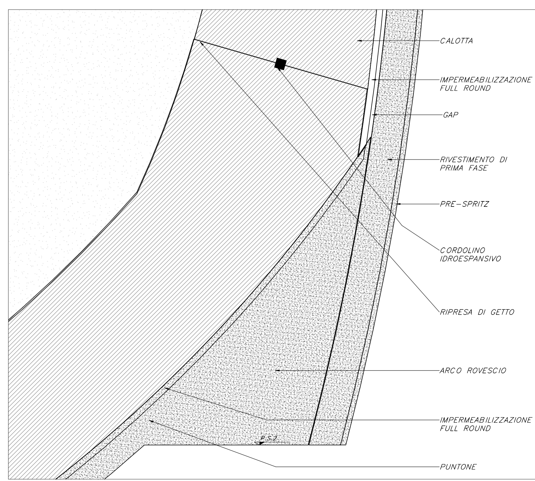
DETTAGLIO 1 SCALA 1:20
