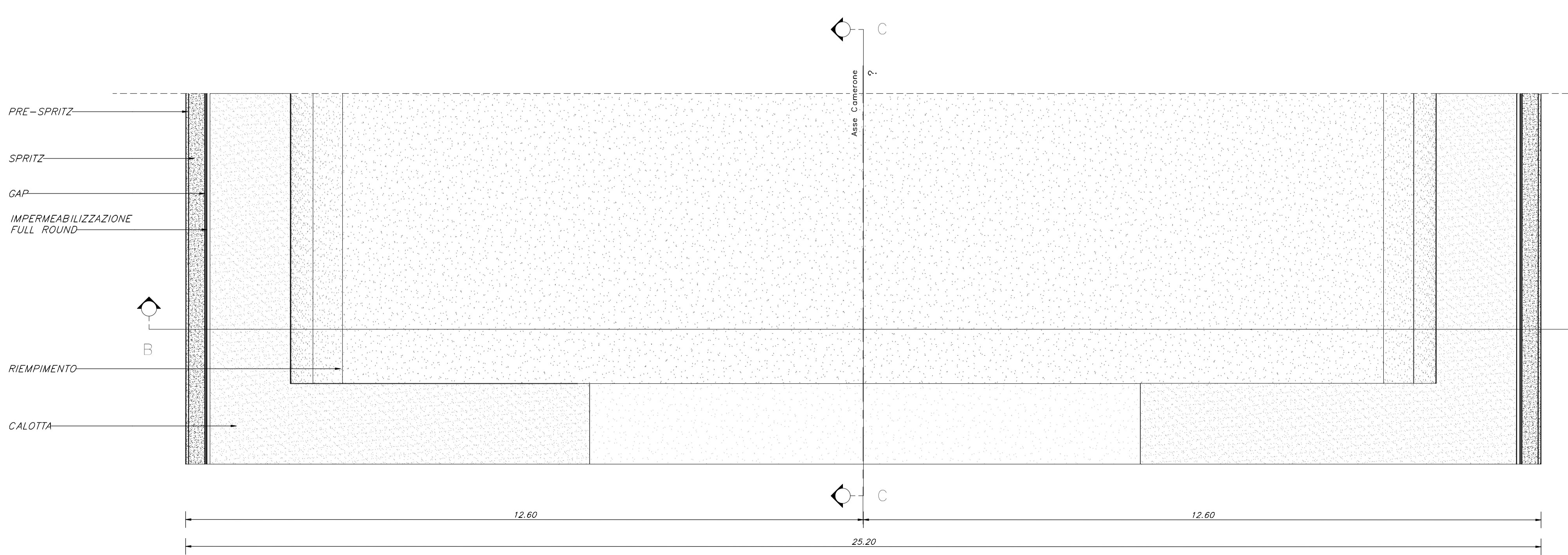
PIANTA P.C. SCALA 1:50
