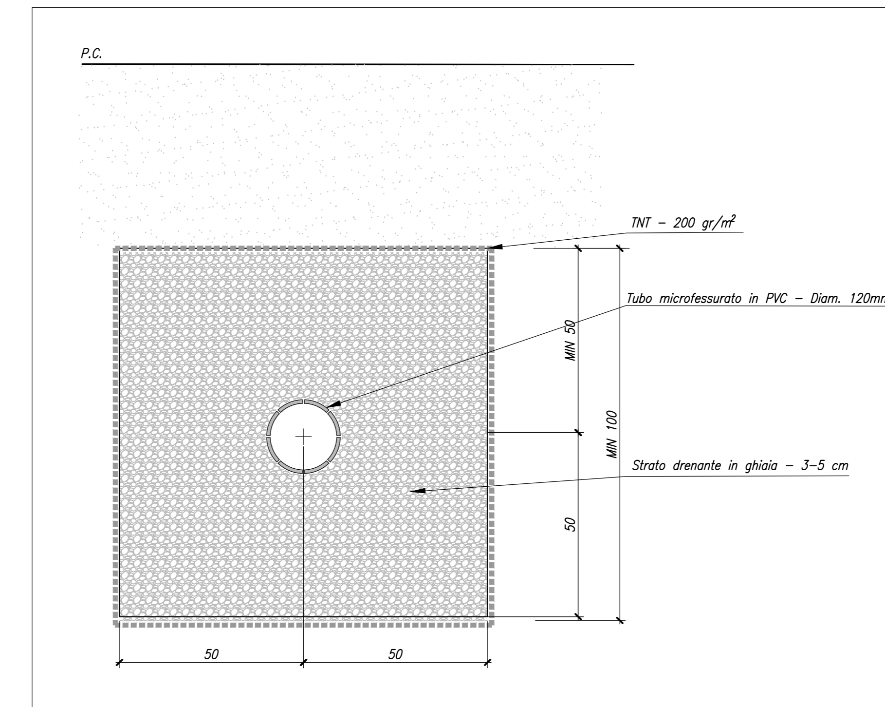
DETTAGLIO TRINCEA DISPERDENTE Scala 1:10
