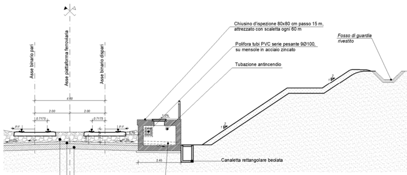
Sezione tipica per il drenaggio in trincea con marciapiede
