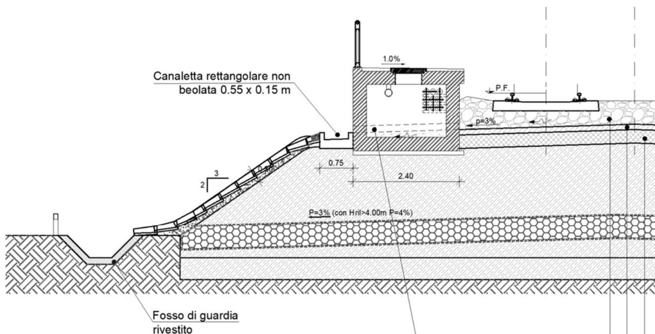
Sezione tipica per il drenaggio in rilevato con marciapiede
