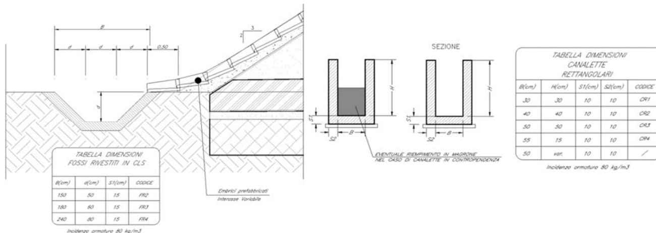
Particolare di fosso rivestito in calcestruzzo (FR) e di canaletta rettangolare (CR), con codifica e dimensioni
