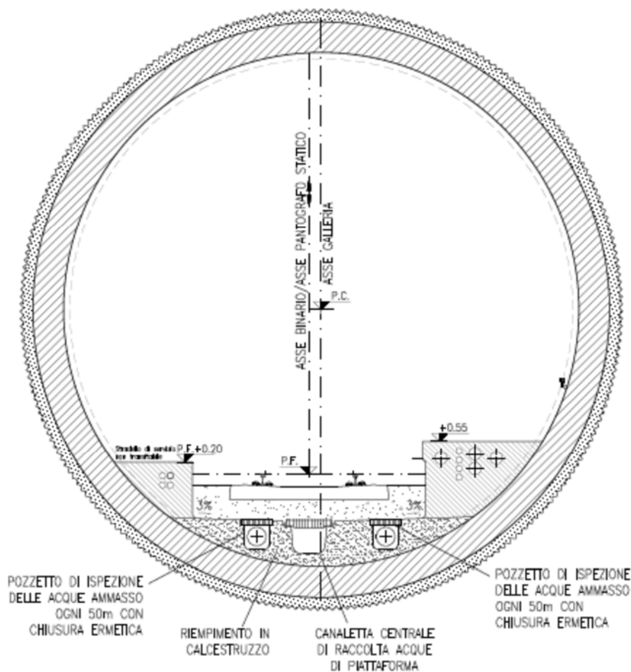
Sezione tipologica per il drenaggio in galleria
