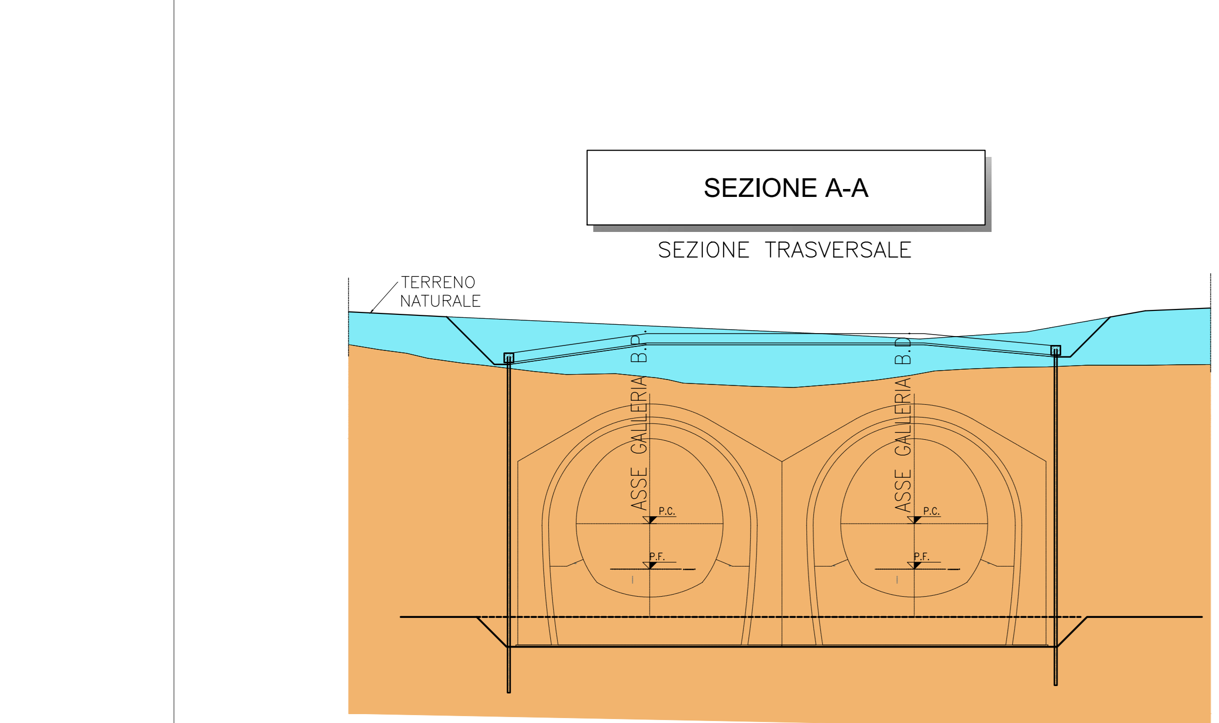
STRALCIO DELLA SEZIONE GEOLOGICA TRASVERSALE - Scala distanze 1:1000, quote 1:1000
