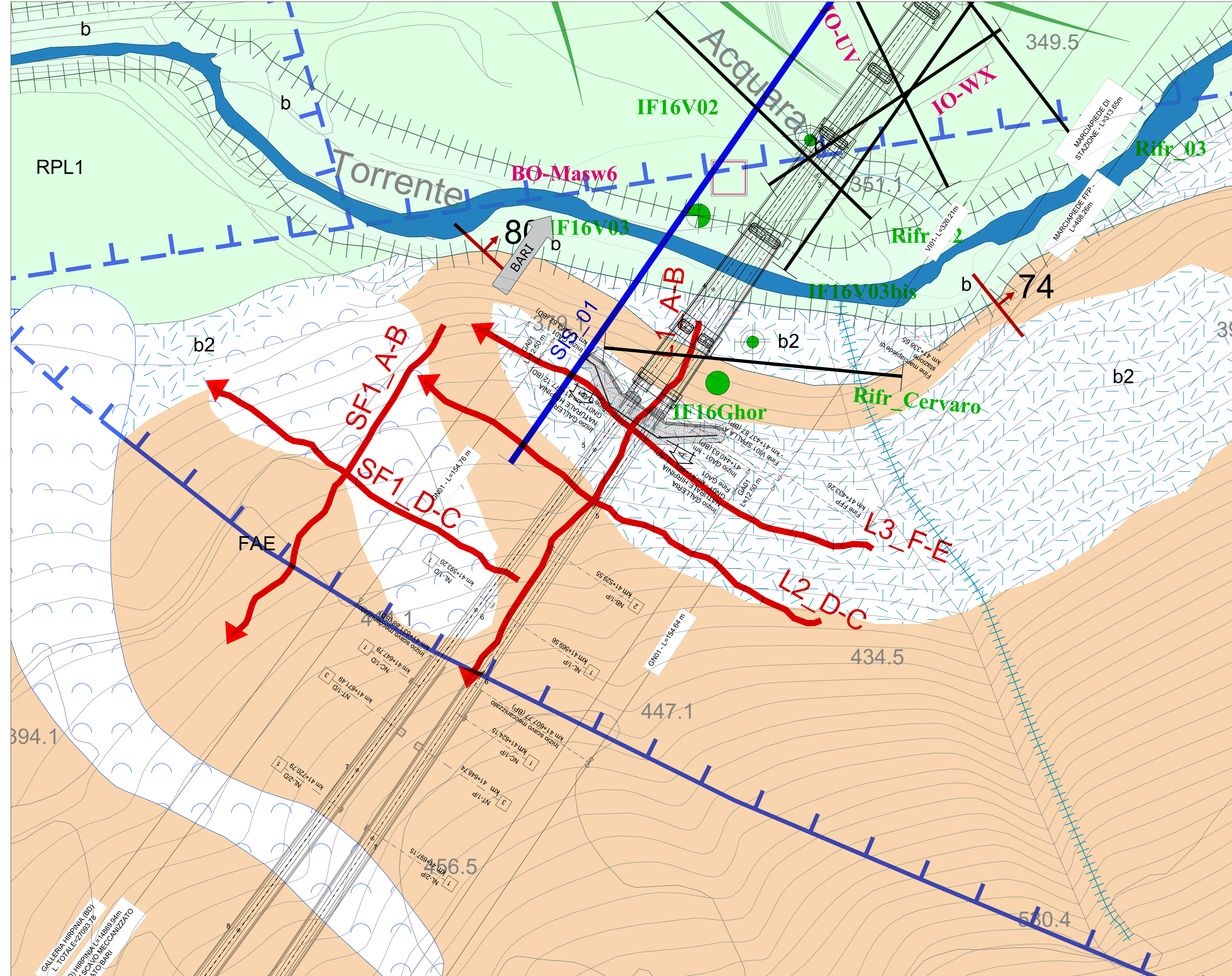
STRALCIO DELLA CARTA GEOLOGICA-GEOMORFOLOGICA - Scala 1:1000
