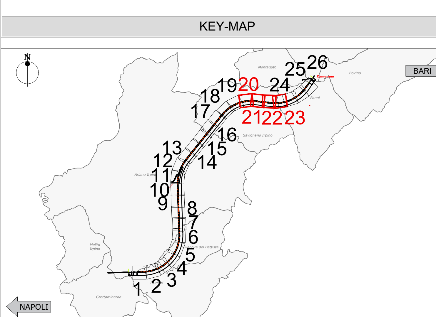
PLANIMETRIA UBICAZIONE NICCHIE SCALA 1:1000 GALLERIA HIRPINIA - 22 di 26
