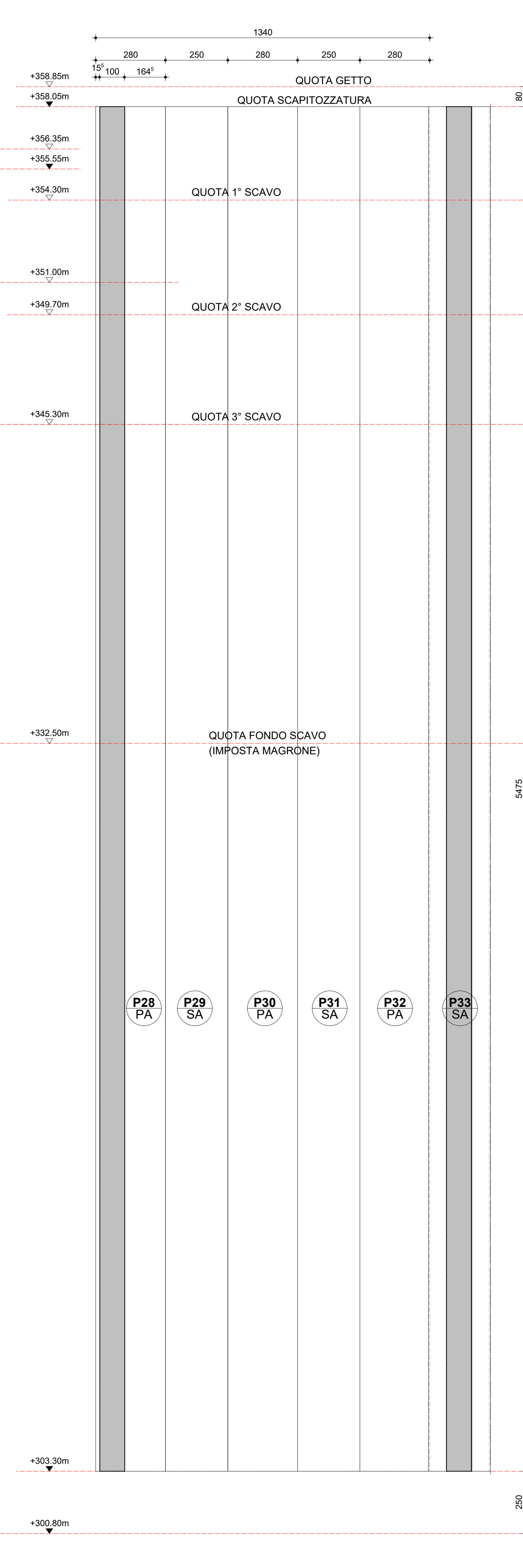
SVILUPPATA E1-E1 SCALA 1:100
