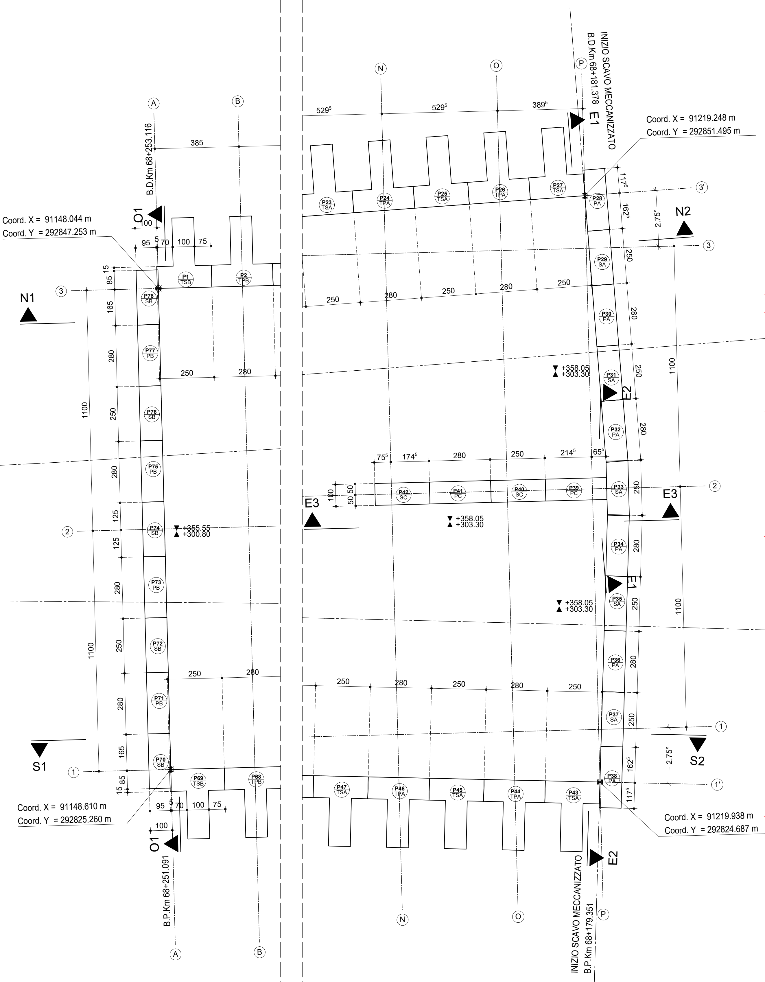
SVILUPPATA O1-O1 SCALA 1:100
