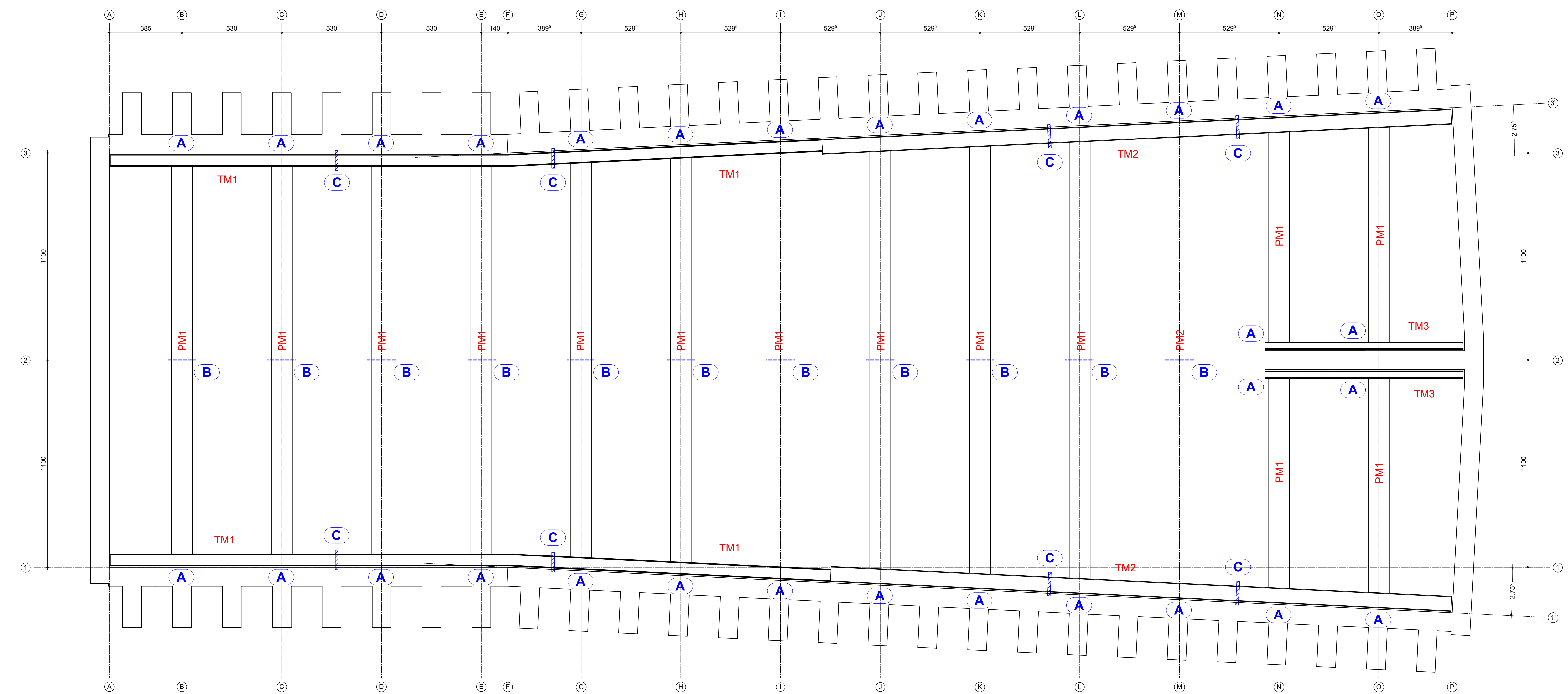
PIANTA CHIAVE COLLEGAMENTI E MONTAGGIO STRUTTURE METALLICHE SCALA 1:100
