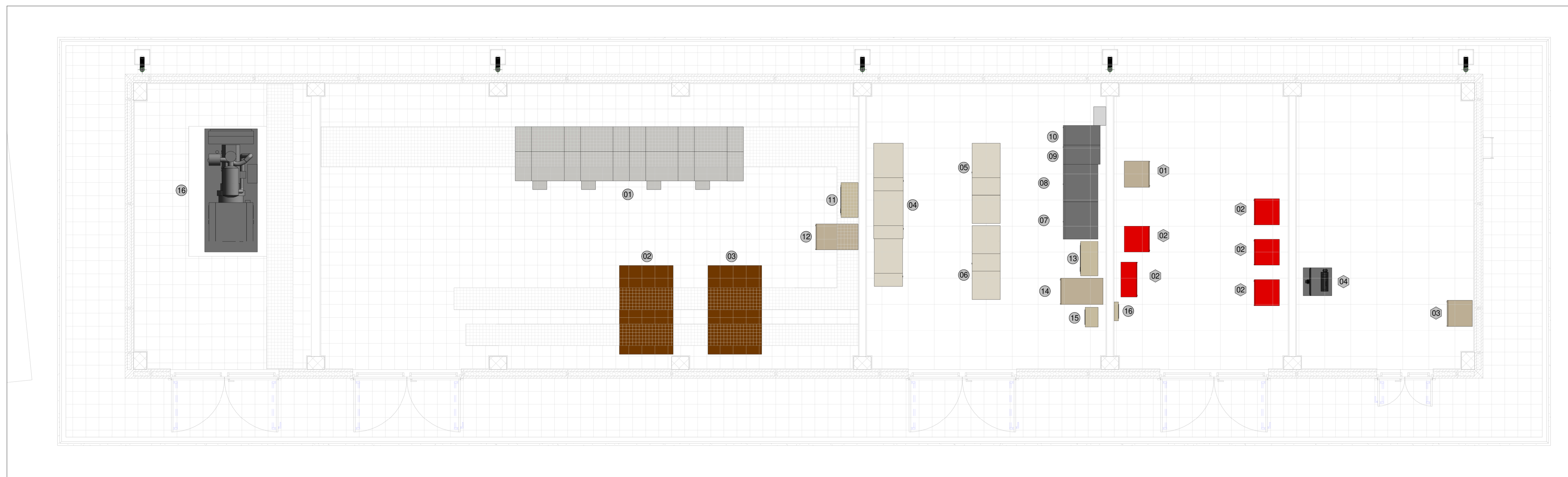
PIANTA DISPOSIZIONE APPARECCHIATURE TLC FA01A 1:50
