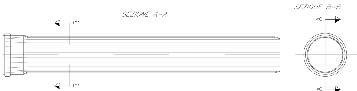
Figura 5 - Dettaglio tipologico collettore circolare – giunto a bicchiere
