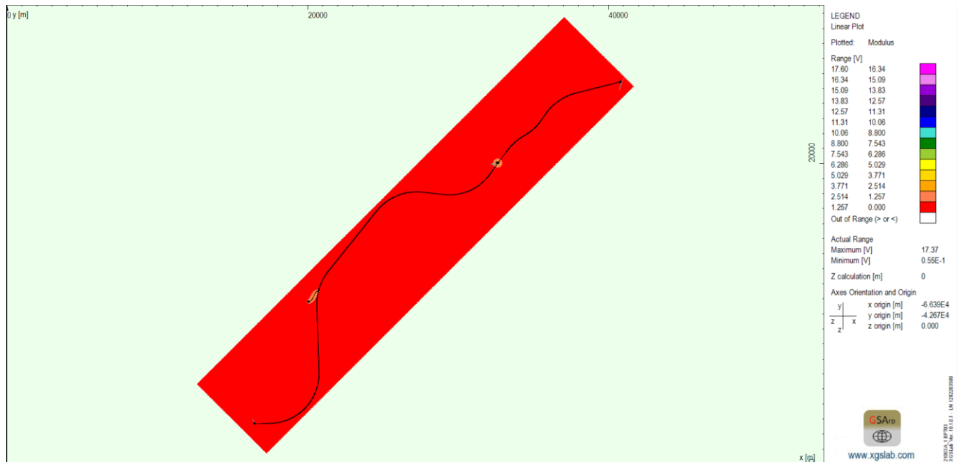
Figura A1-4 - Distribuzione 2D dei potenziali sulla superficie del terreno (impianto di terra complessivo)
