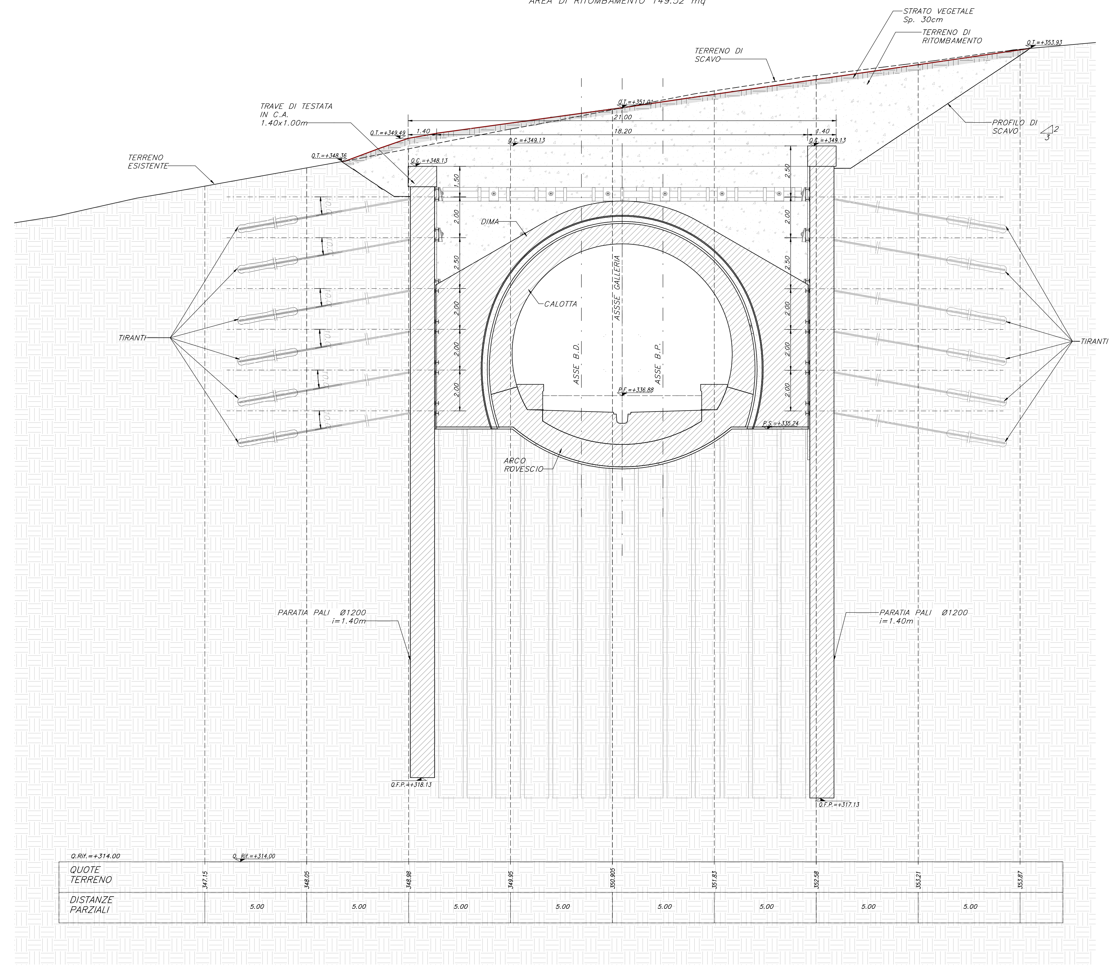
SEZIONE A-A SCALA 1:100 PK 68+534.10 AREA DI RITOMBAMENTO 149.52 mq
