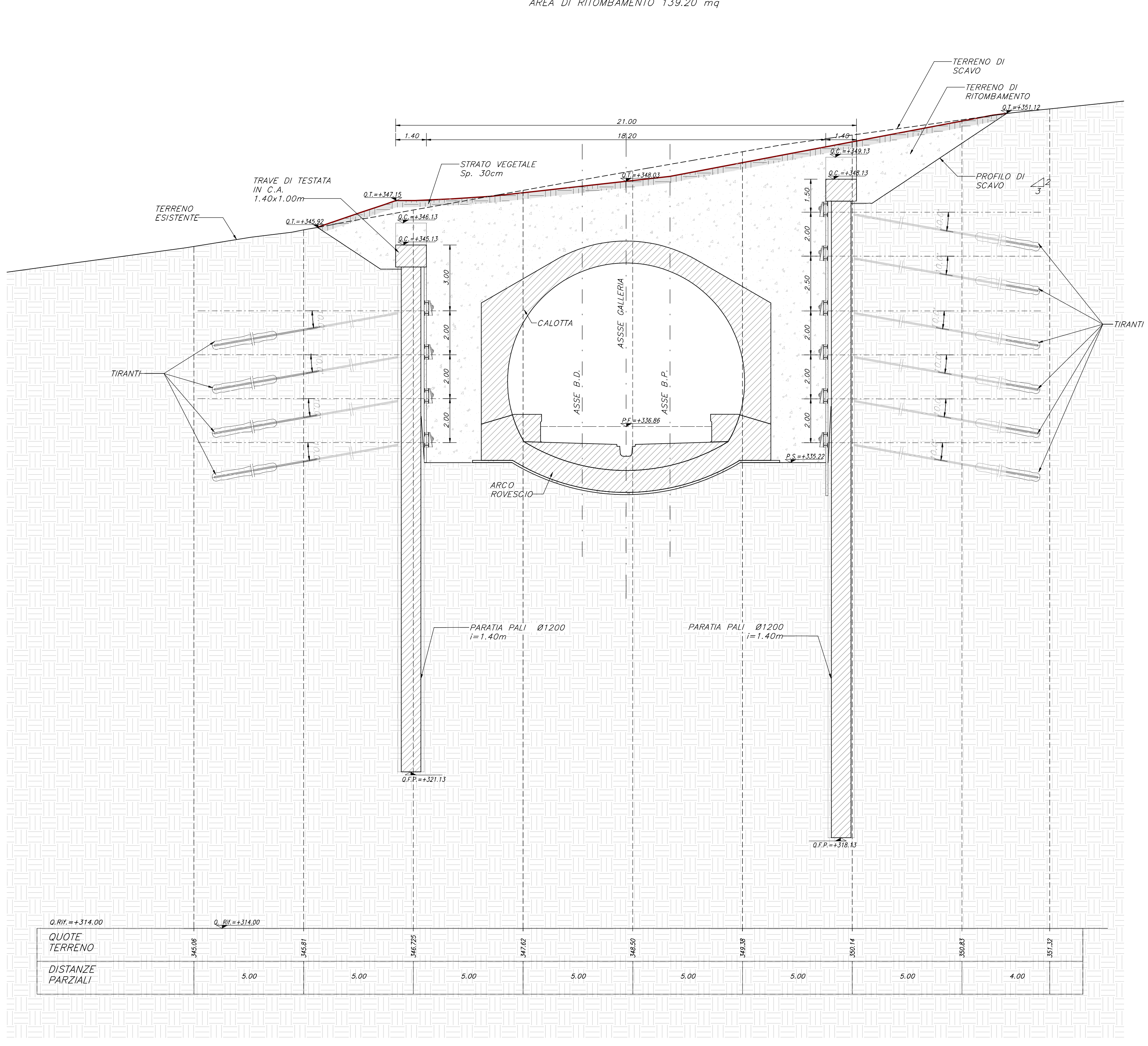
SEZIONE B-B SCALA 1:100 PK 68+545.10 AREA DI RITOMBAMENTO 139.20 mq
