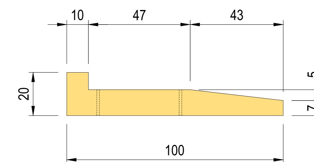
(*) dettaglio elementi prefabbricati modulari
