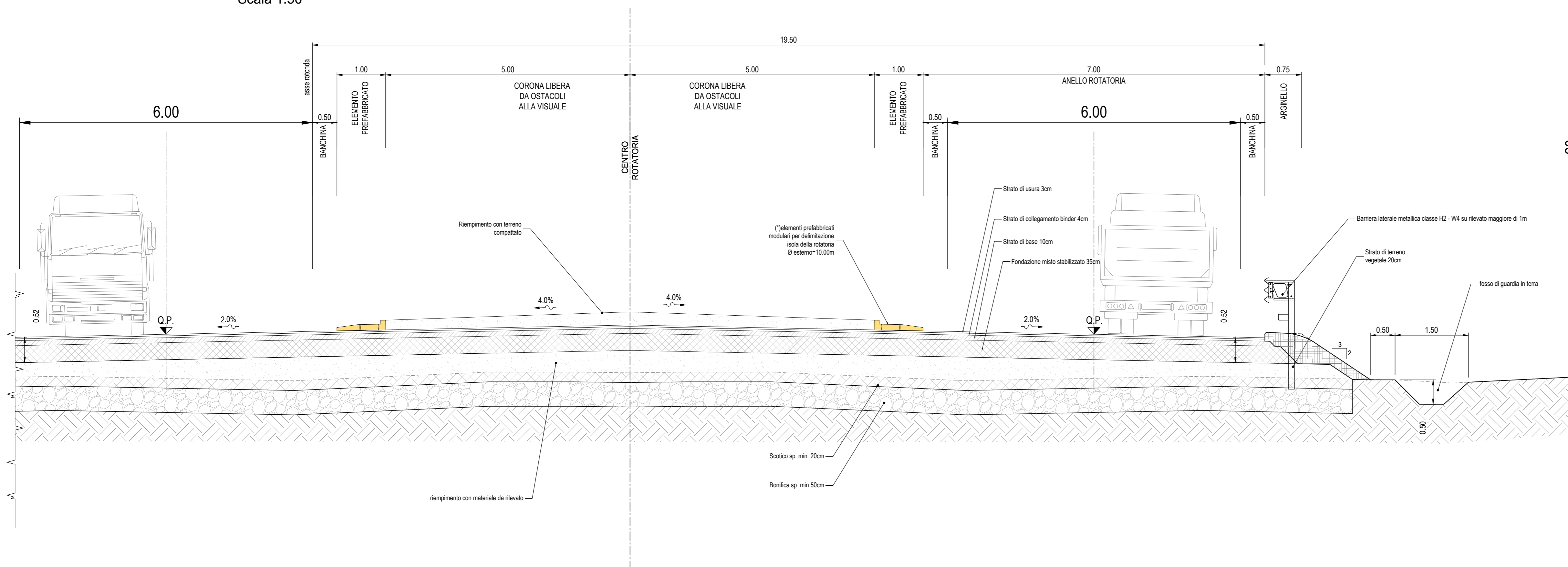
SEZIONE TIPO ROTATORIA SU S.S.90 Scala 1:50
