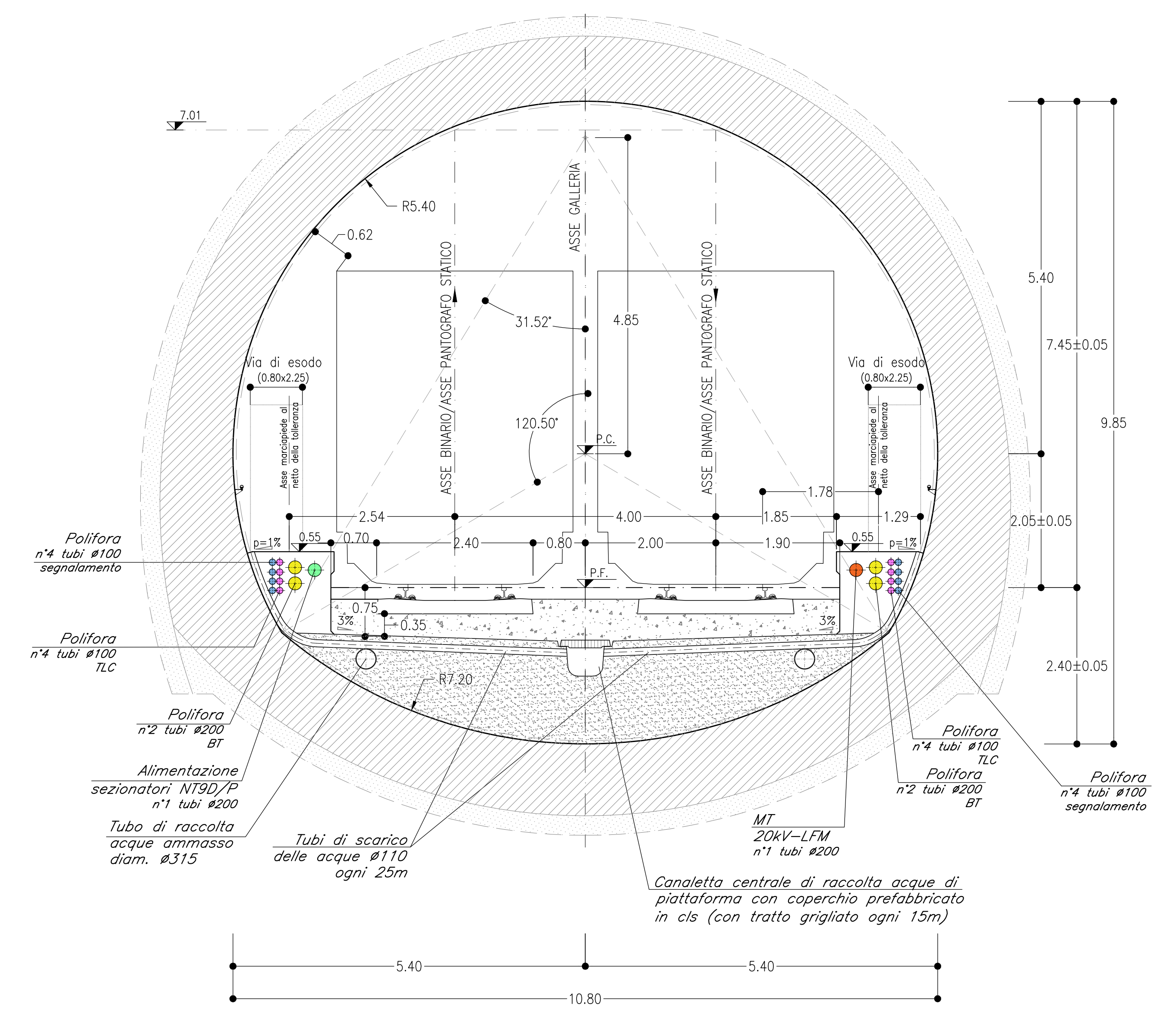
GALLERIA NATURALE DOPPIO BINARIO SCAVO IN TRADIZIONALE - SEZIONE CORRENTE 160 km/h <math>V \le 200 \text{ km/h}</math> SCALA 1:50
