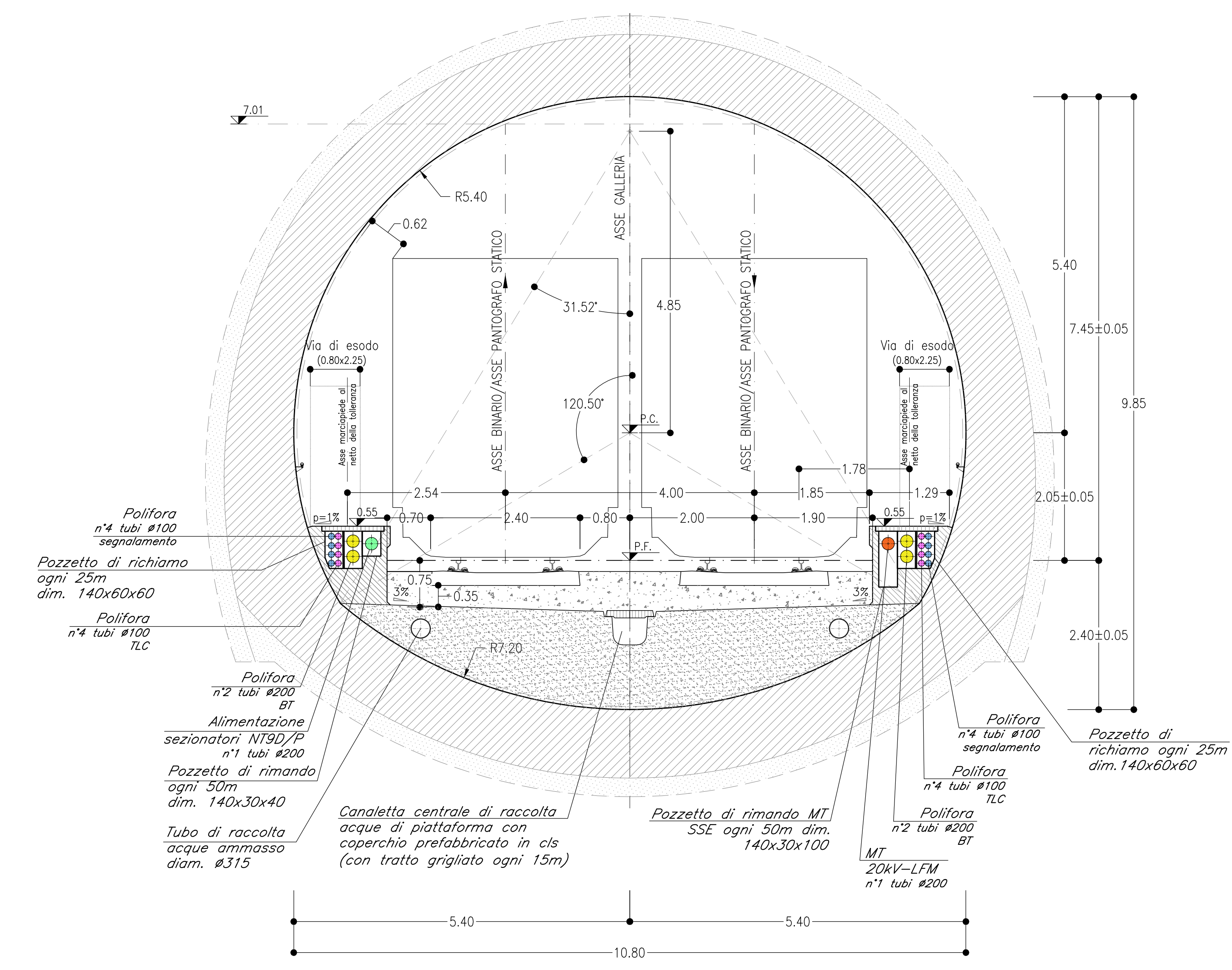
GALLERIA NATURALE DOPPIO BINARIO SCAVO IN TRADIZIONALE - SEZIONE IN CORRISPONDENZA DEI POZZETTI DI RIMANDO 160 km/h <math>V \le 200 \text{ km/h}</math> SCALA 1:50
