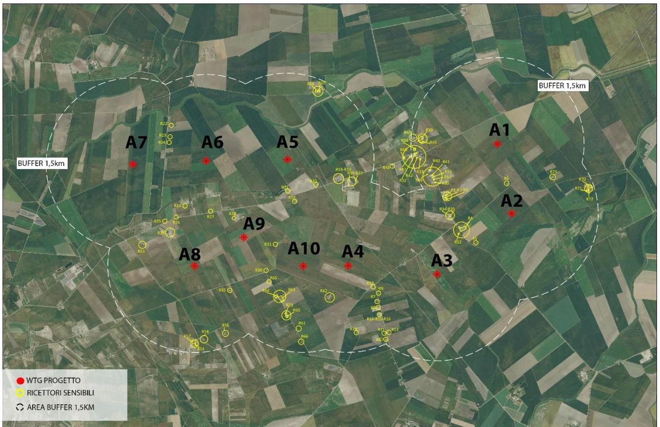
figura 13: Vista generale dell'area di studio su ortofoto estratta da Google Earth, con evidenza delle turbine di progetto e dei ricettori sensibili rientranti nel buffer di 1,5 km dalle torri.
