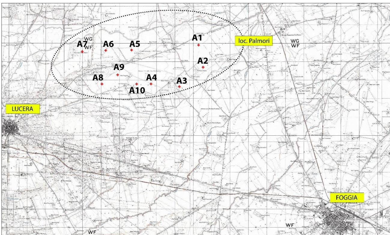
figura 10: inquadramento impianto di Progetto su IGM 1.25000
