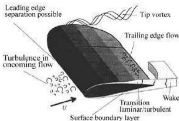
figura 2: Flussi di aria intorno al profilo alare di una turbina eolica.
