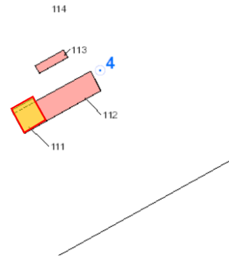
figura 20: Inquadramento geografico della postazione fonometrica PF 01 ed inquadramento catastale del ricettore R28.
