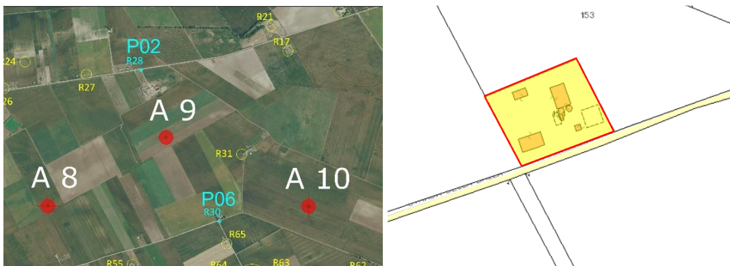
figura 28: Inquadramento geografico della postazione fonometrica PF 01 ed inquadramento catastale del ricettore R30.
