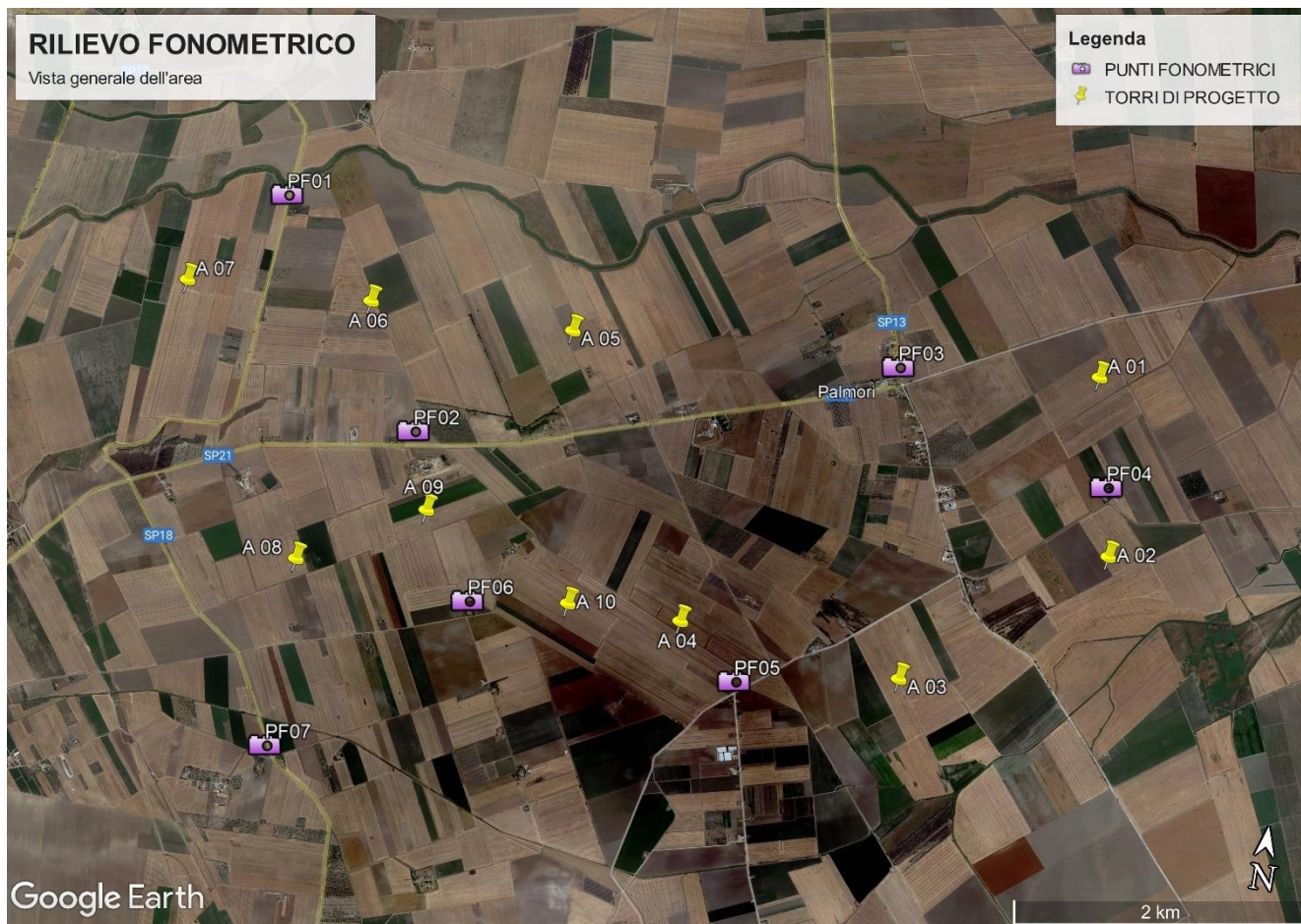
Figura 17: Inquadramento geografico dell'area di progetto e delle postazioni fonometriche scelte.
