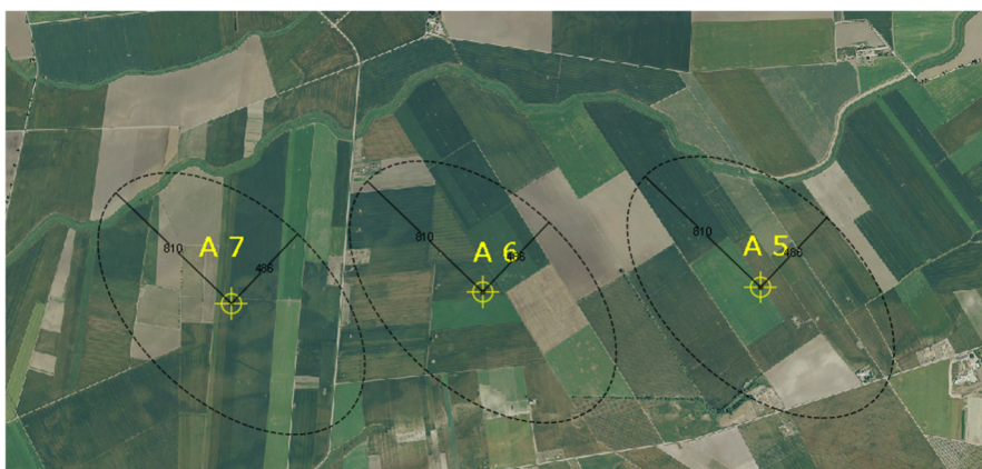
figura 16: schema del layout di progetto con indicazione delle interdistanze tra gli aerogeneratori.
