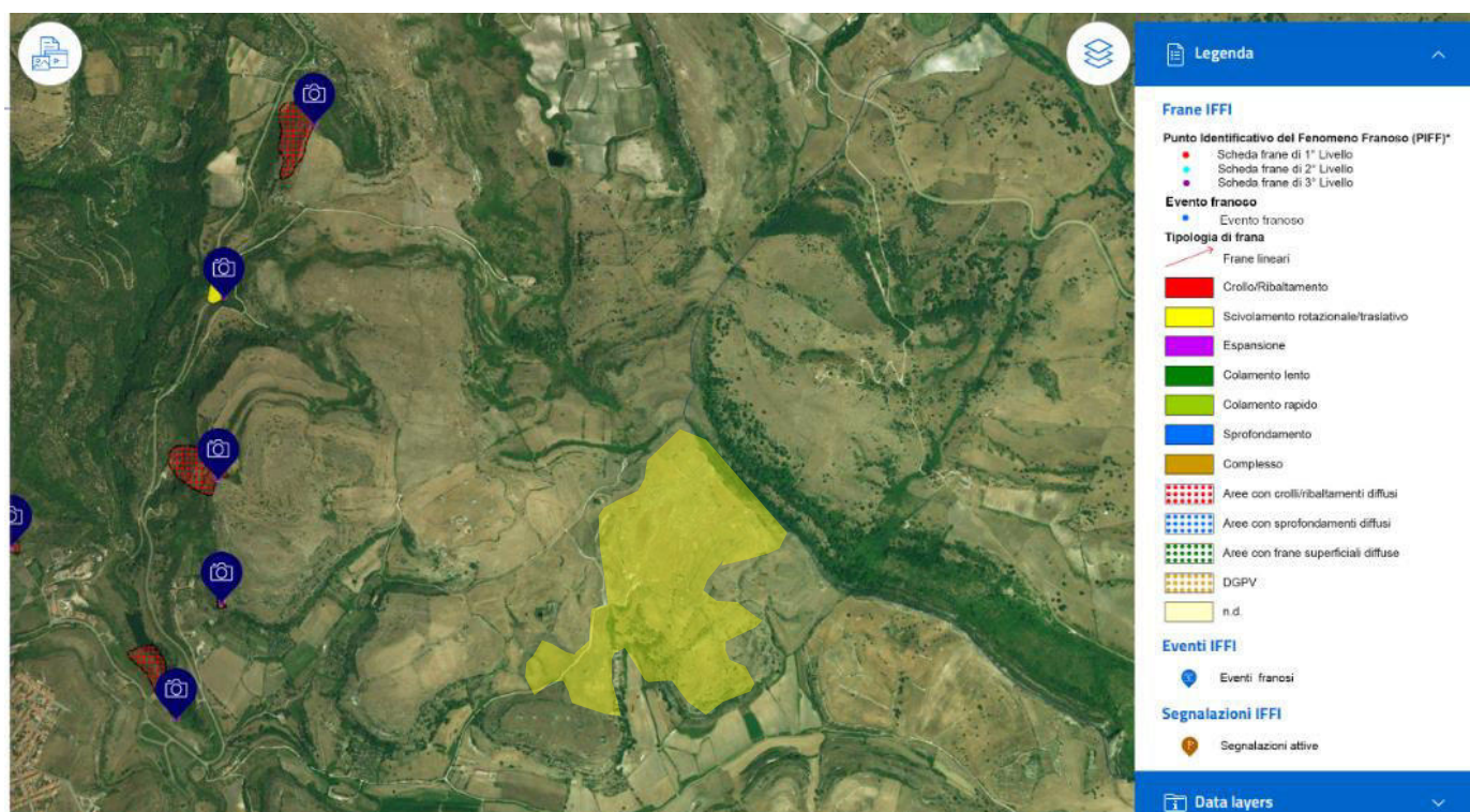
Figura 4-2 Censimento frane_Progetto IFFI (ISPRA)
