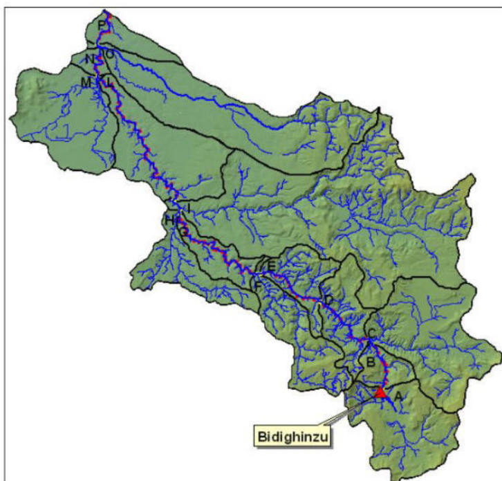
Figura 4-5 Suddivisione in sottobacini del bacino idrografico del Flumini Mannu di Porto Torres; in rosso è
