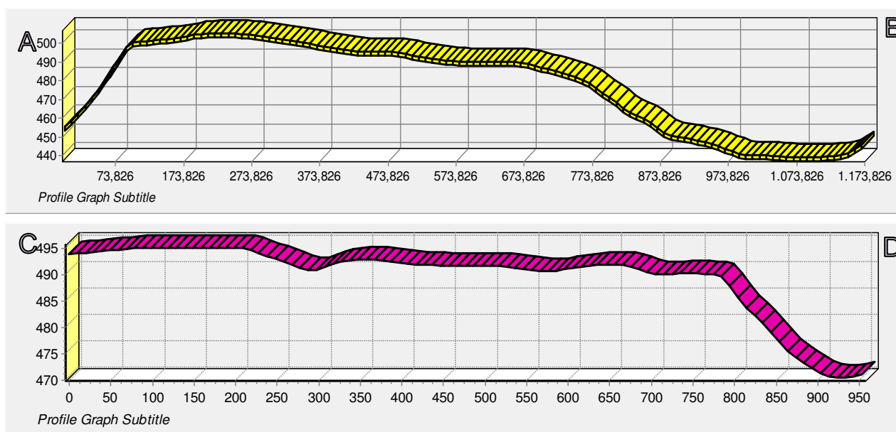
Figura 4-1 Profili altimetrici dell'area di interesse
