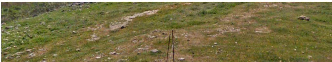
Figura 4-4 Dettaglio roccia affiorante
