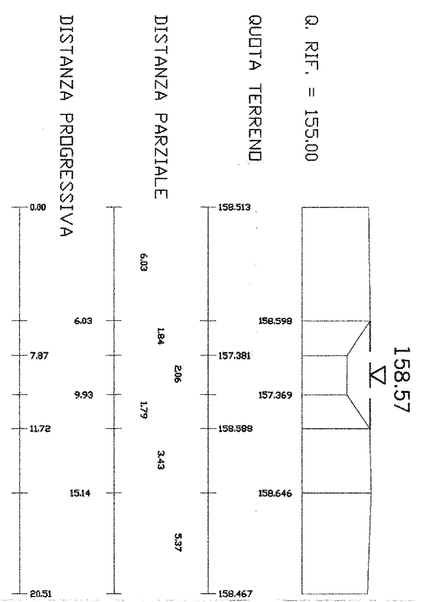
SEZIONE R12 B Scala 1:200/200
