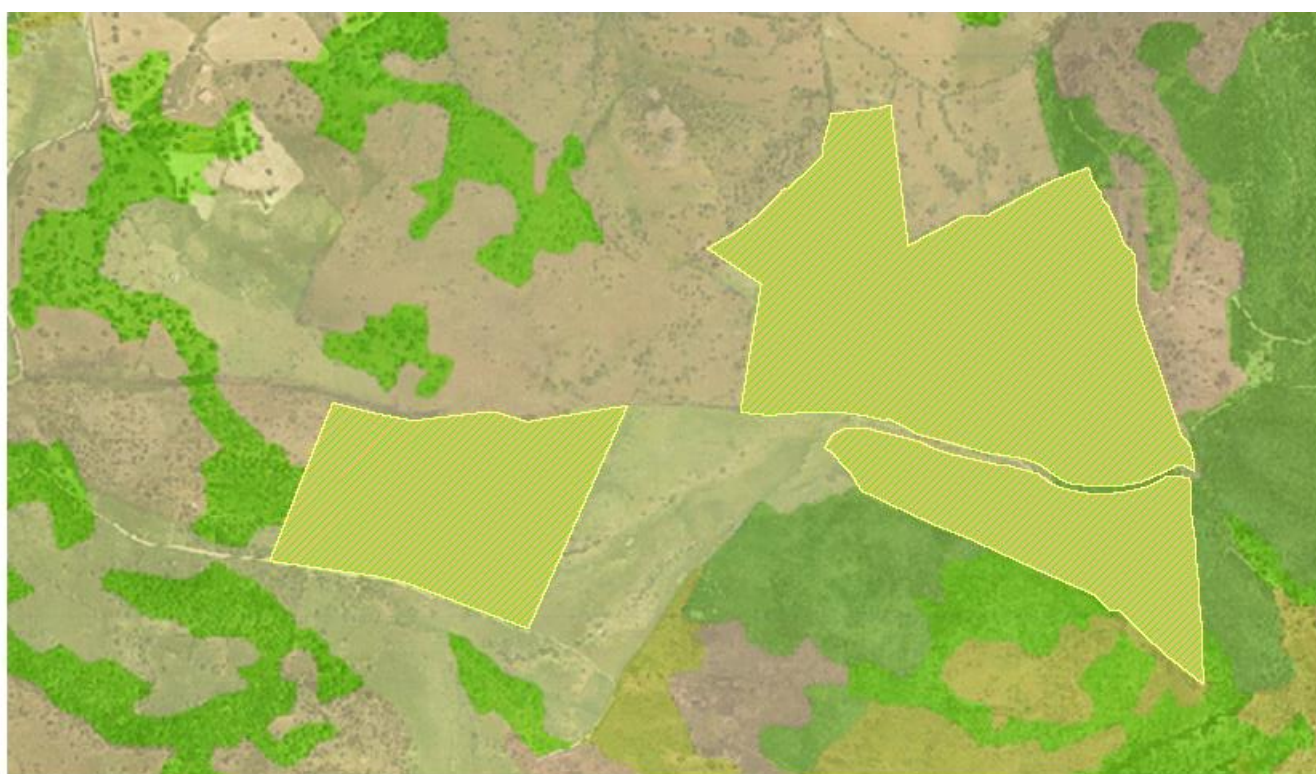
Area di intervento Paesaggi su rocce effusive acide, (andesiti, rioliti, rioladati, etc.) e intermedie (fanaliti) del Cenozoico e loro depositi di versante, colluvi (Fonte: Osservatorio Regionale Suoli Sardegna)
