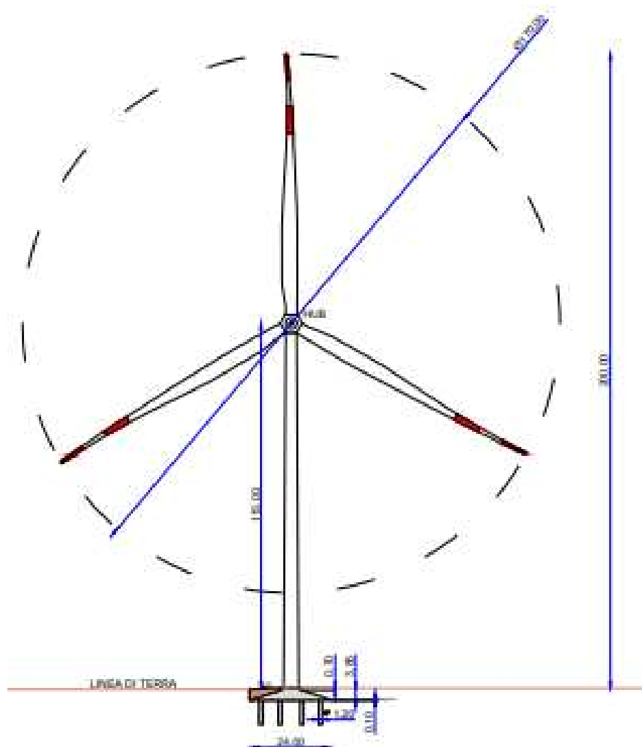
Fig. 1- Tipico Aerogeneratore
