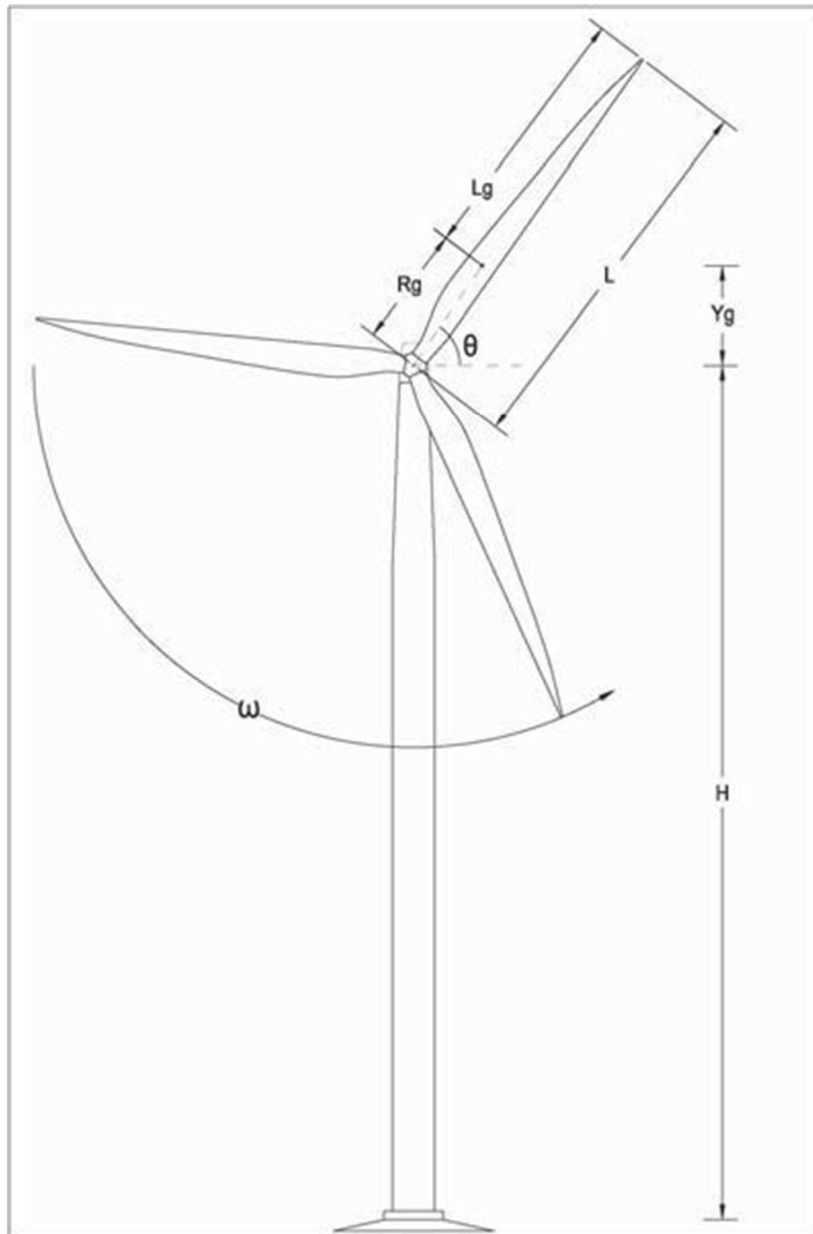
Fig.4: Grandezze di calcolo della gittata massima
