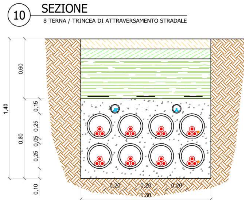
Fig. 2 Sezione tipo cavidotto su strada asfaltata
