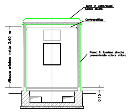
SEZIONE W-W
