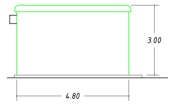
VISTA LATERALE
