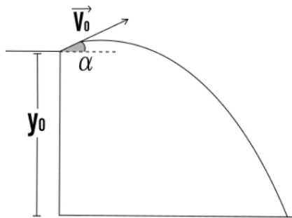
Figura 7 – Metodo di calcolo teorico della gittata massima
