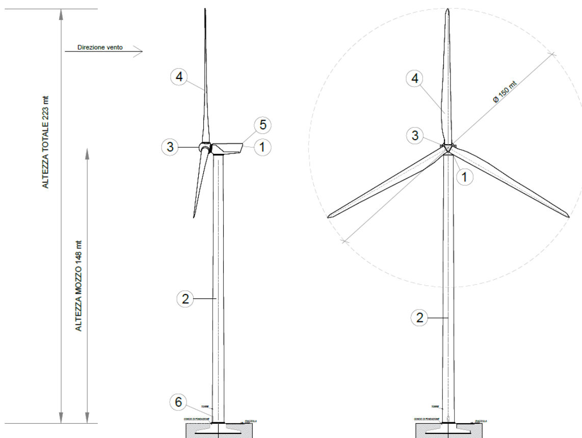
Figura 3 – Tipico dell'aerogeneratore in progetto con dimensioni di ingombro
