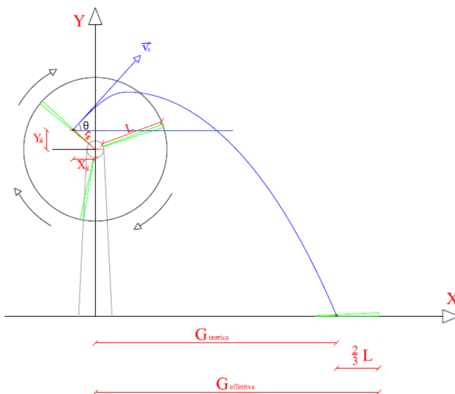
Figura 9 – Rappresentazione della legge di caduta di un grave, lanciato nello spazio con velocità iniziale v_0 e con una inclinazione rispetto all'orizzontale di \theta
