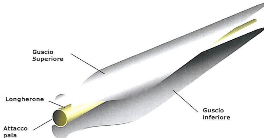
Figura 6 - Componenti di un'ala
