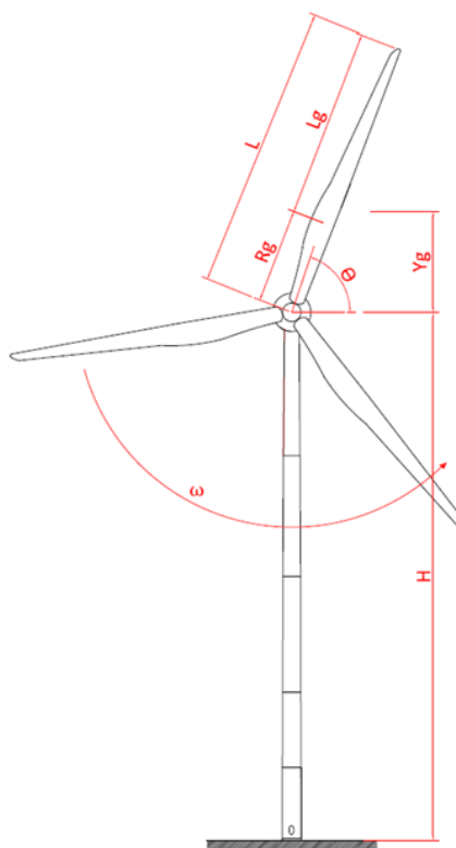
Figura 8 – Parametri geometrici assunti per il calcolo del moto parabolico
