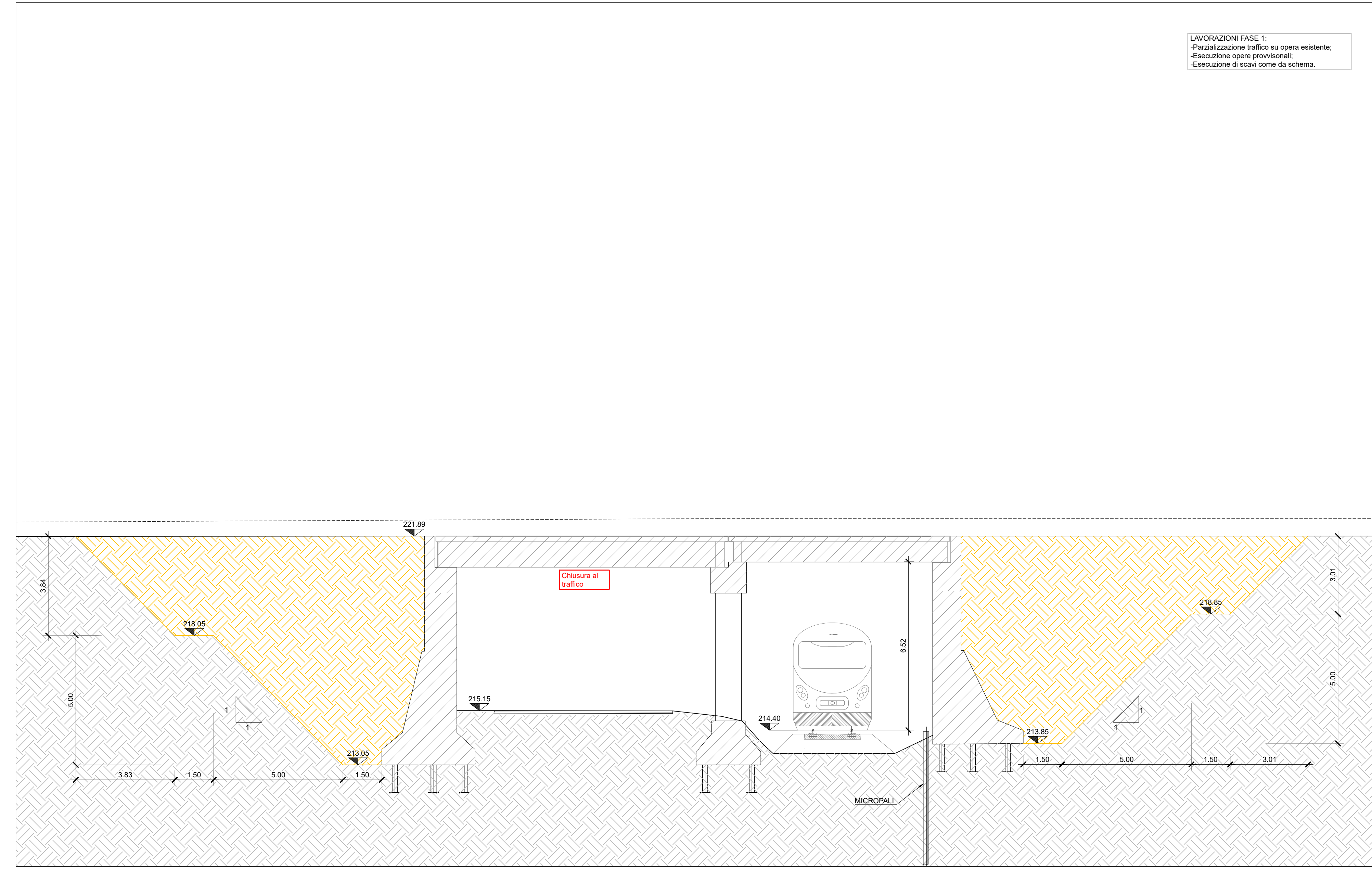
SEZIONE LONGITUDINALE FASE 1 1:100
