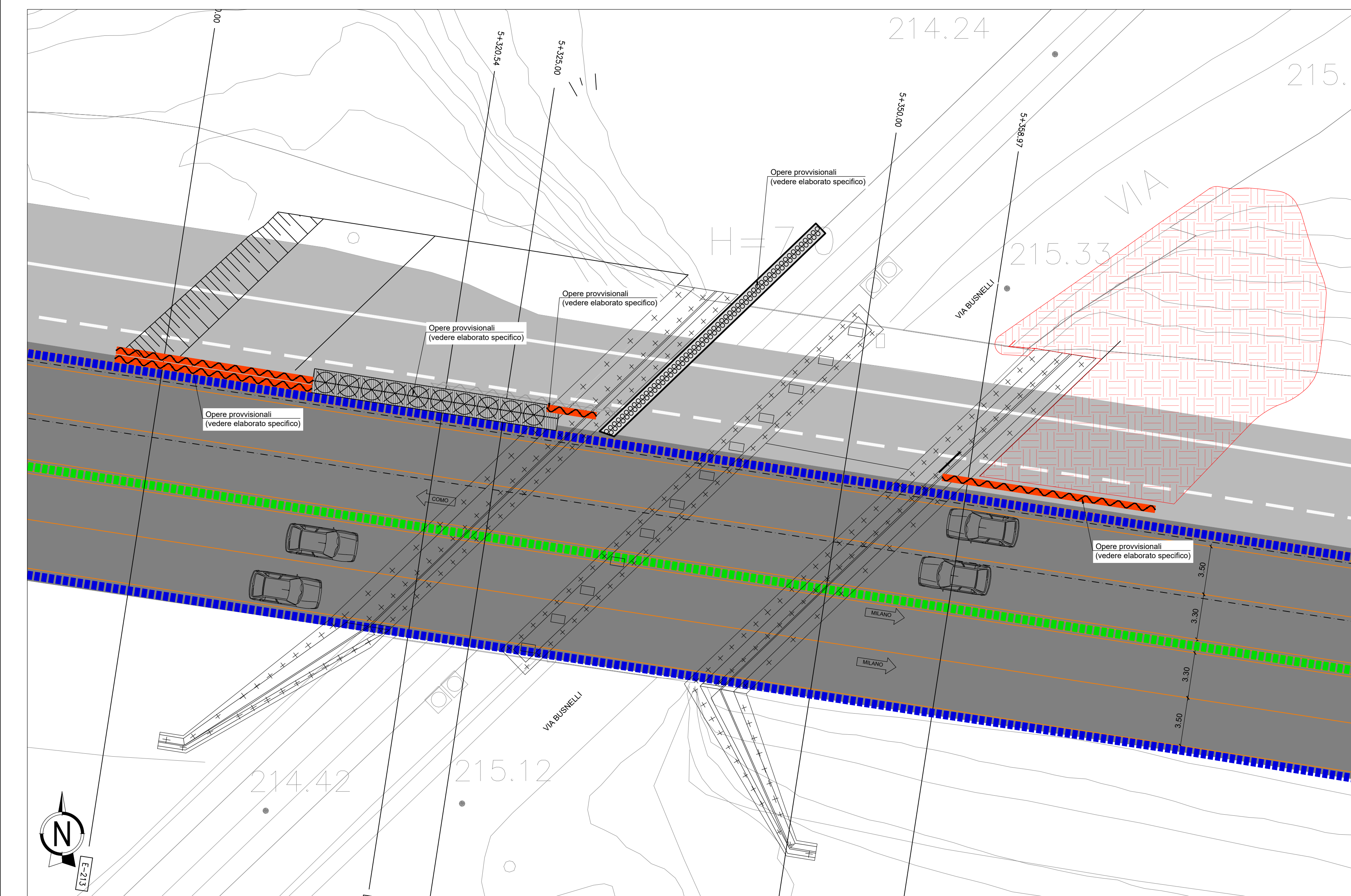
PLANIMETRIA FASE 2 1:200
