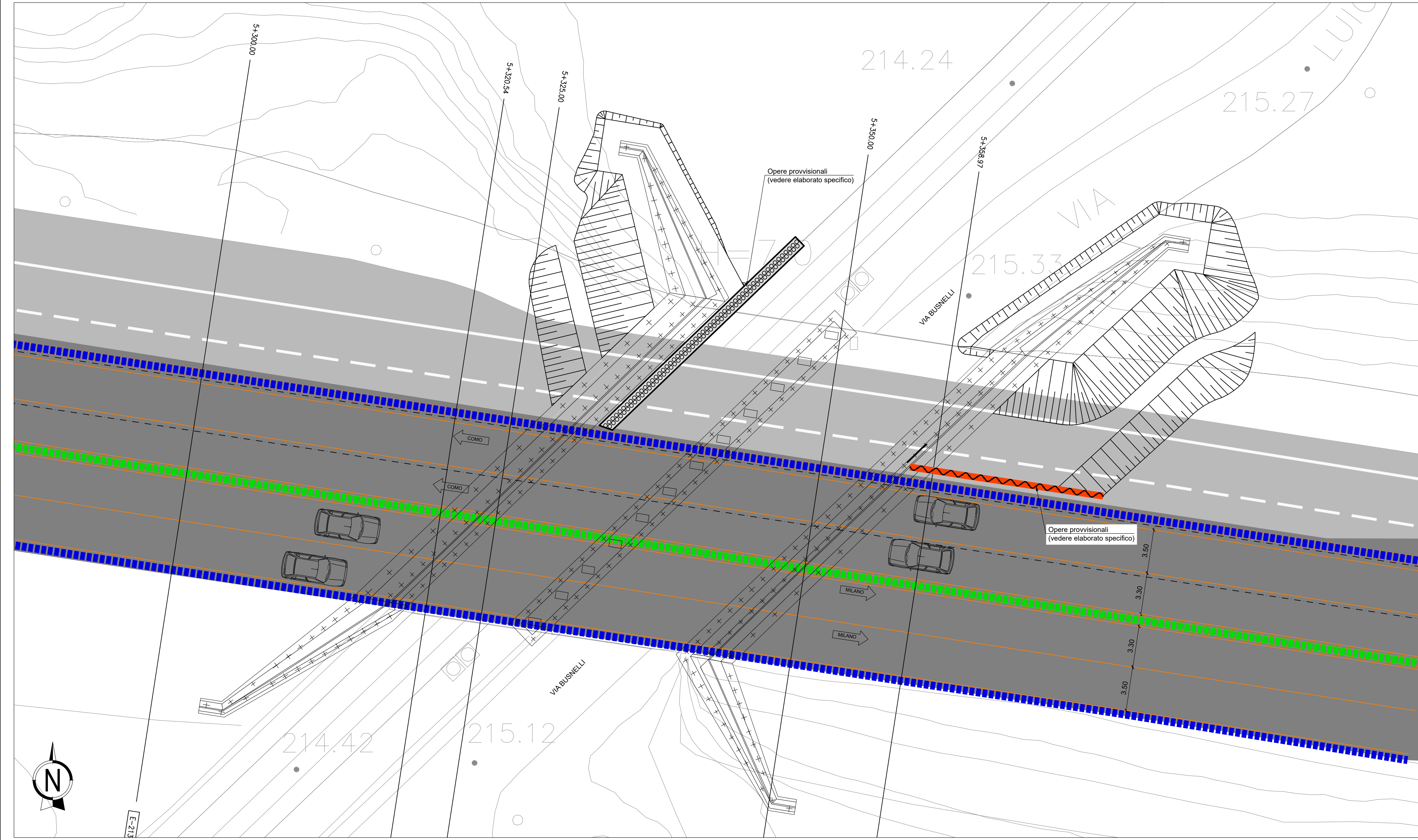
PLANIMETRIA FASE 1 1:200
