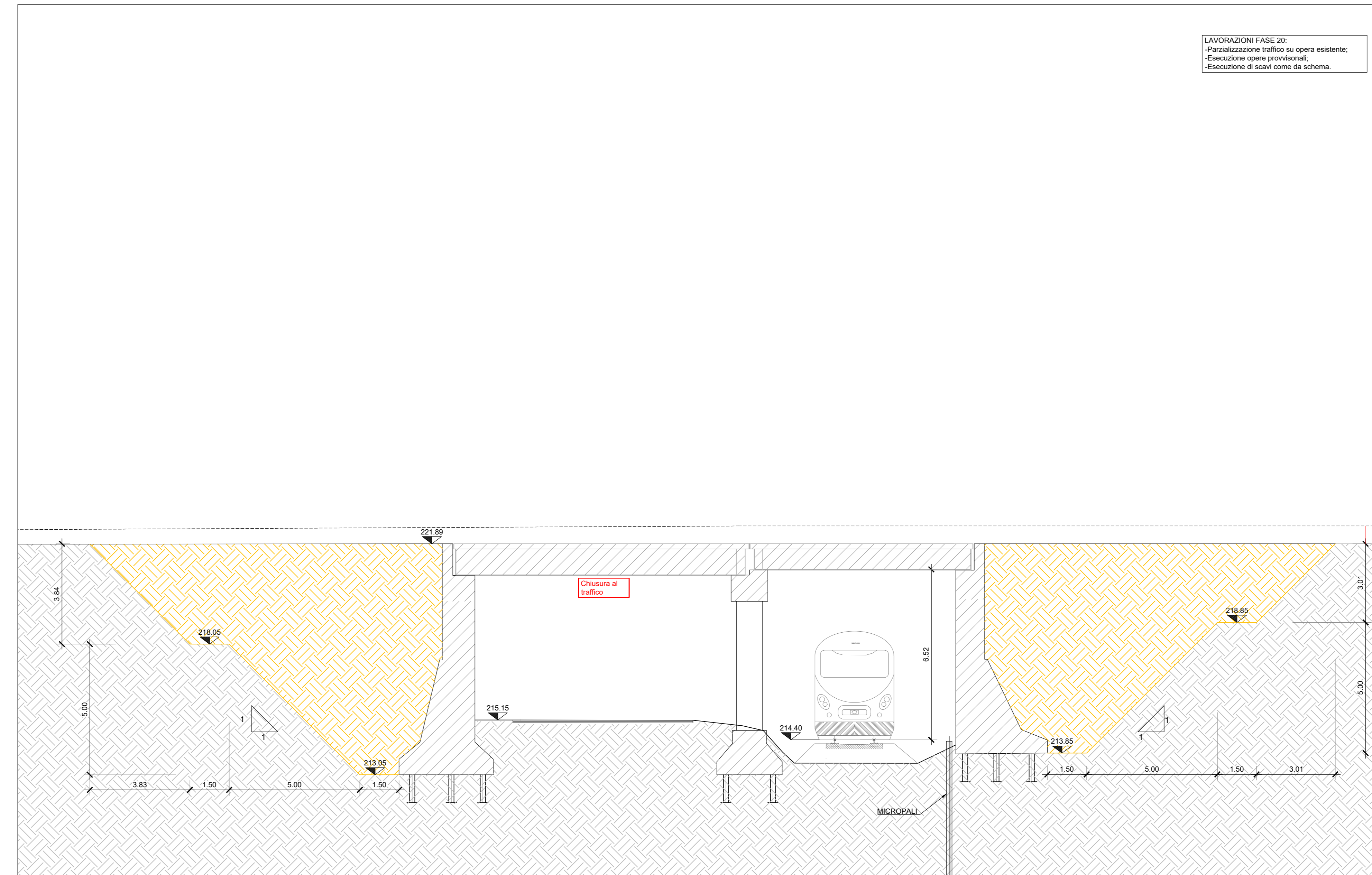
SEZIONE LONGITUDINALE FASE 20 1:100
