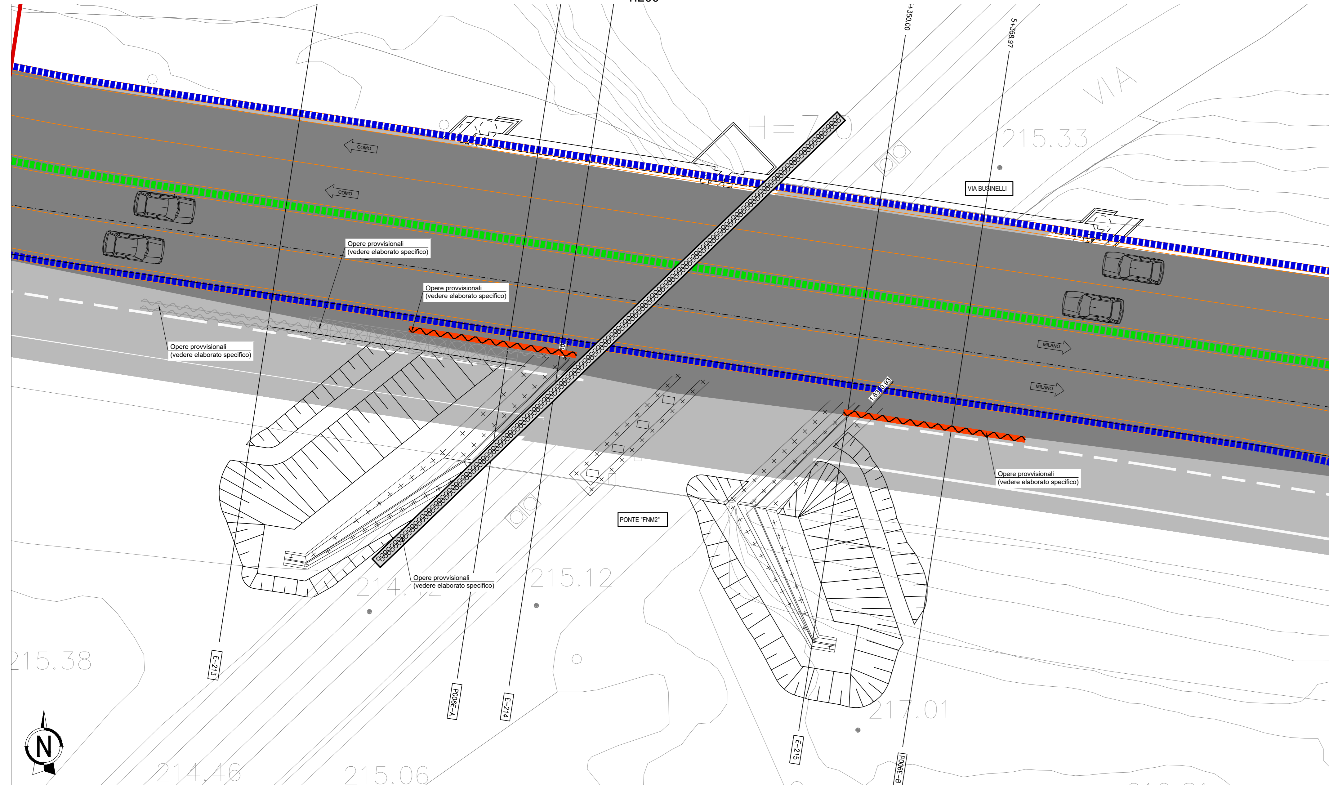
PLANIMETRIA FASE 20 1:200
