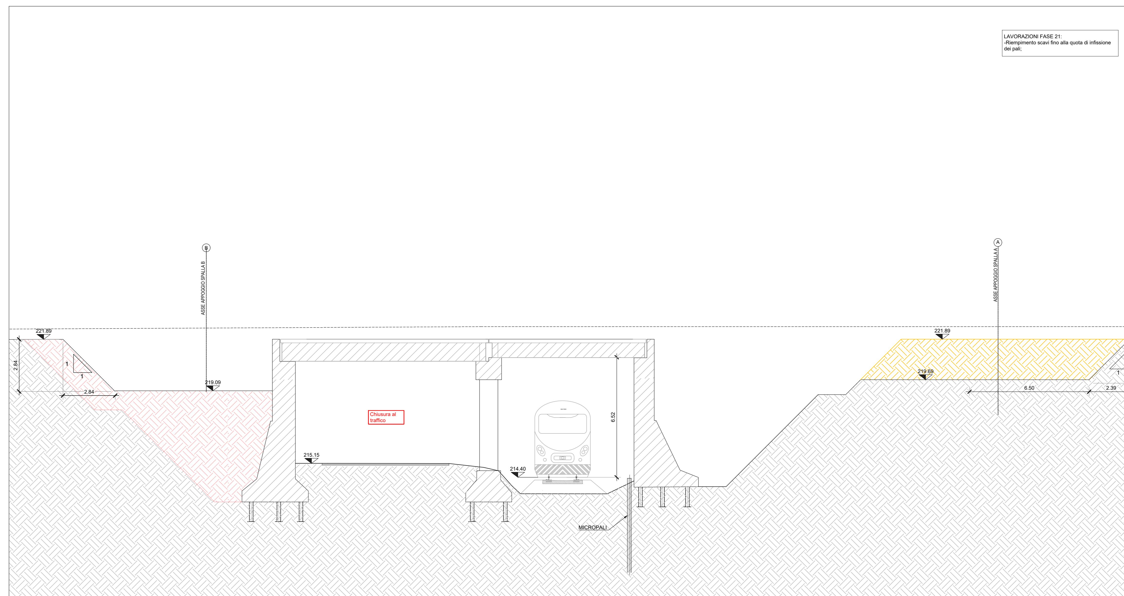
SEZIONE LONGITUDINALE FASE 21 1:100
