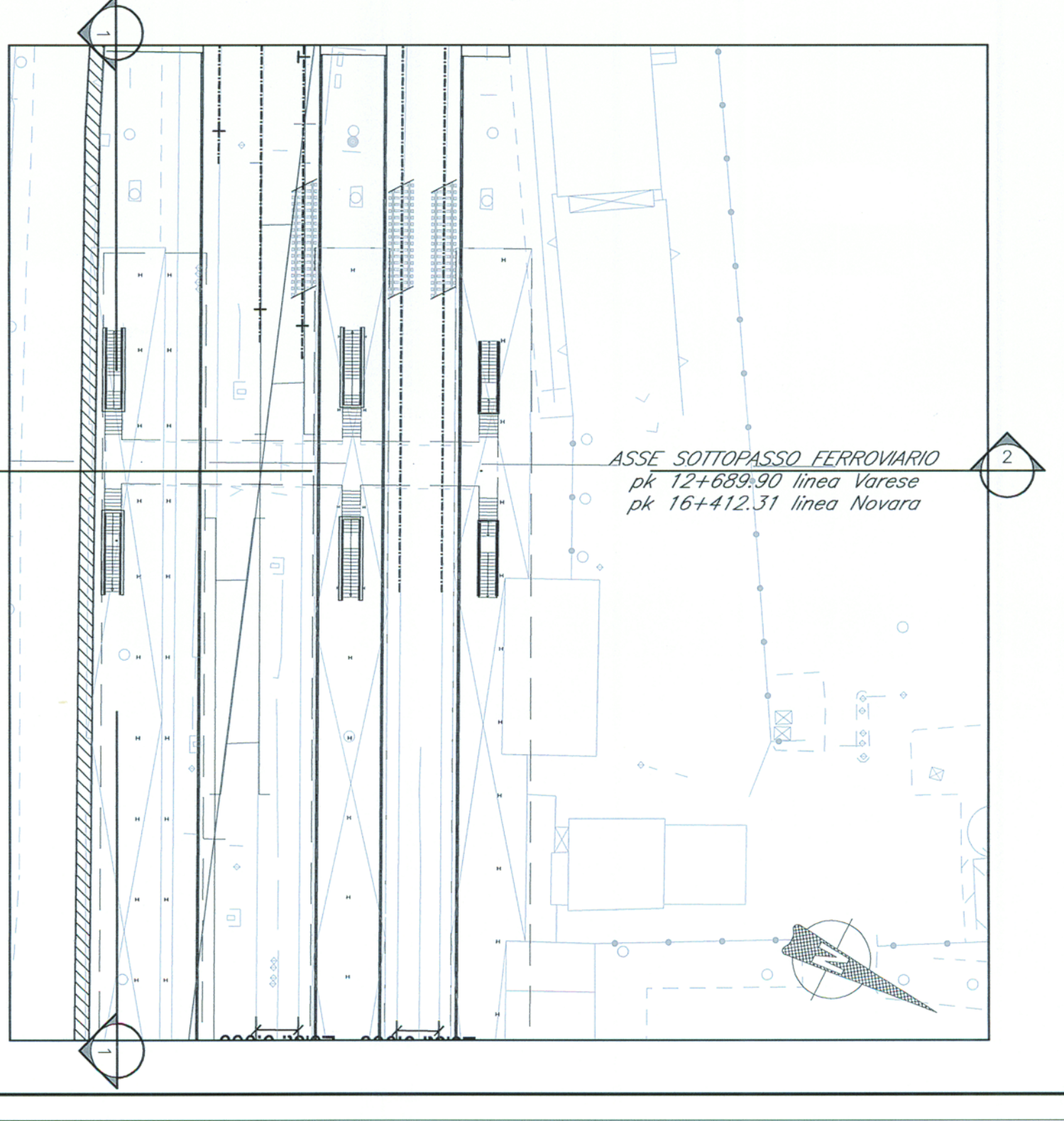
3 PIANI POST OPERAM scala 1:500
