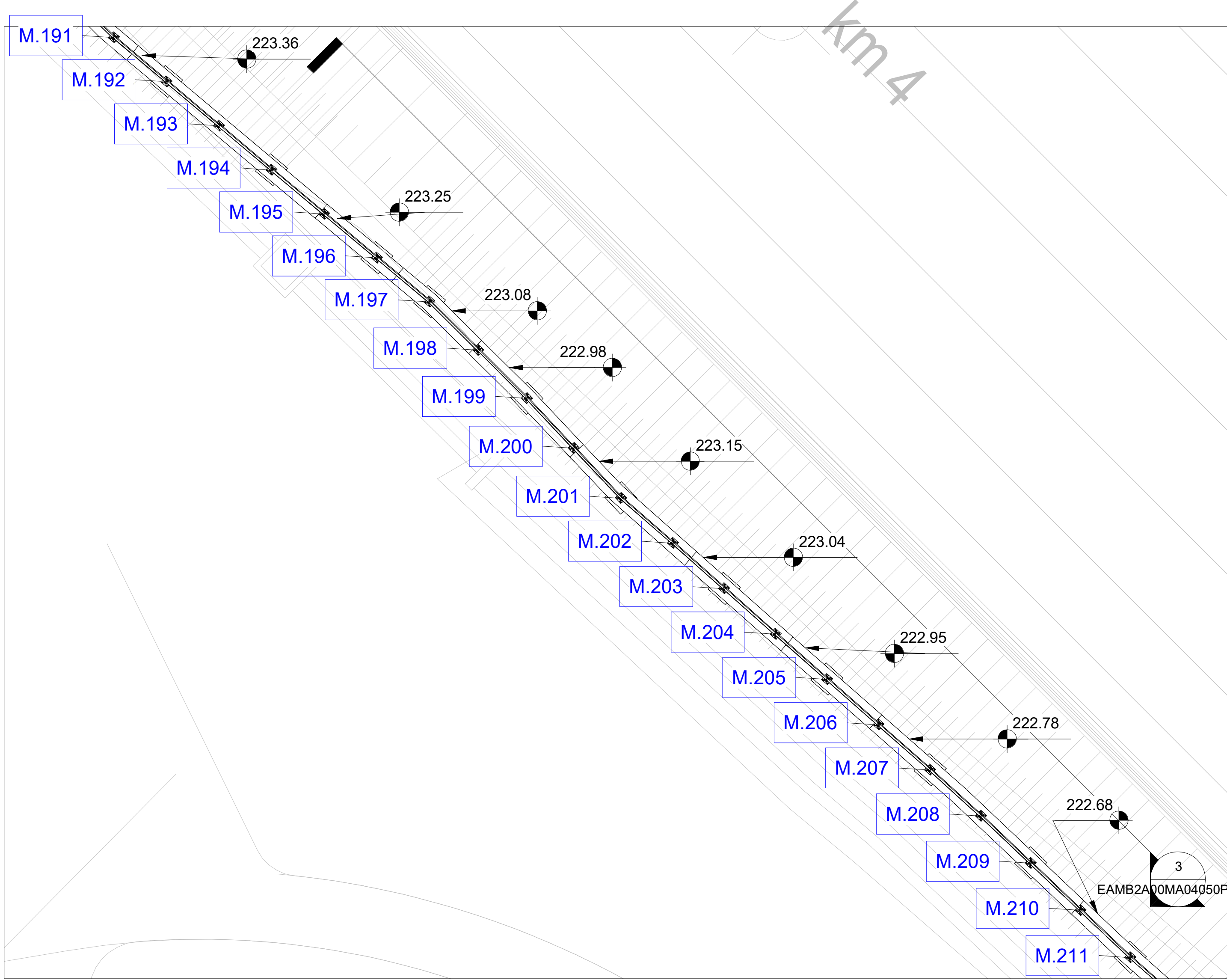
Stralcio Planimetrico 28a pt4
