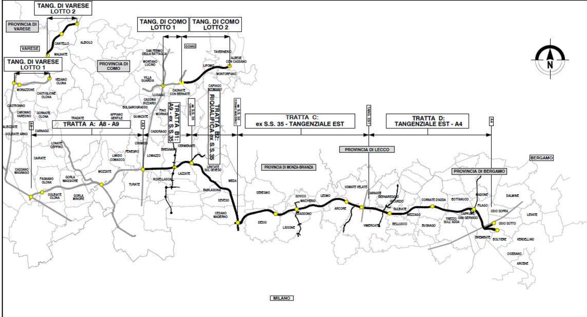
QUADRO DI UNIONE GENERALE
