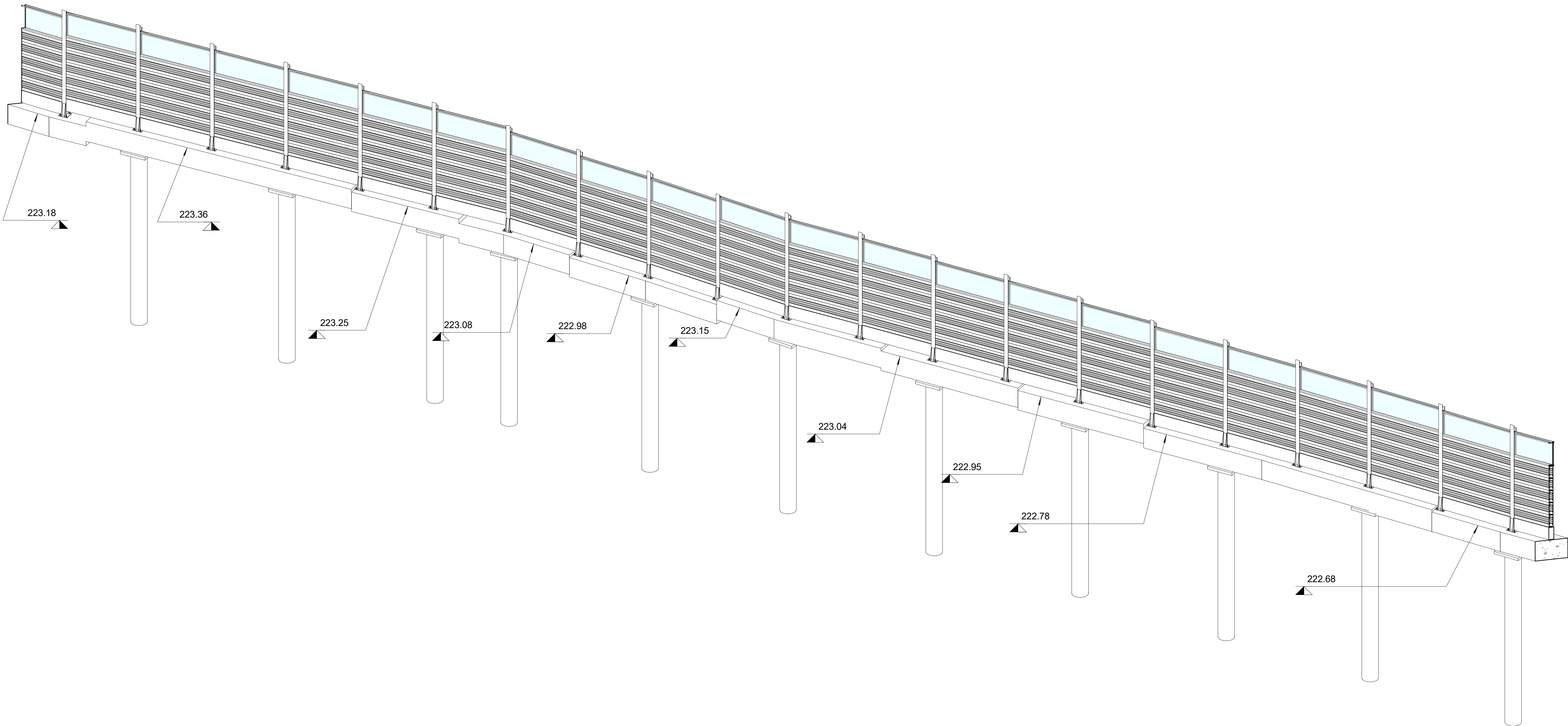
Assonometria WBS 28a pt4
