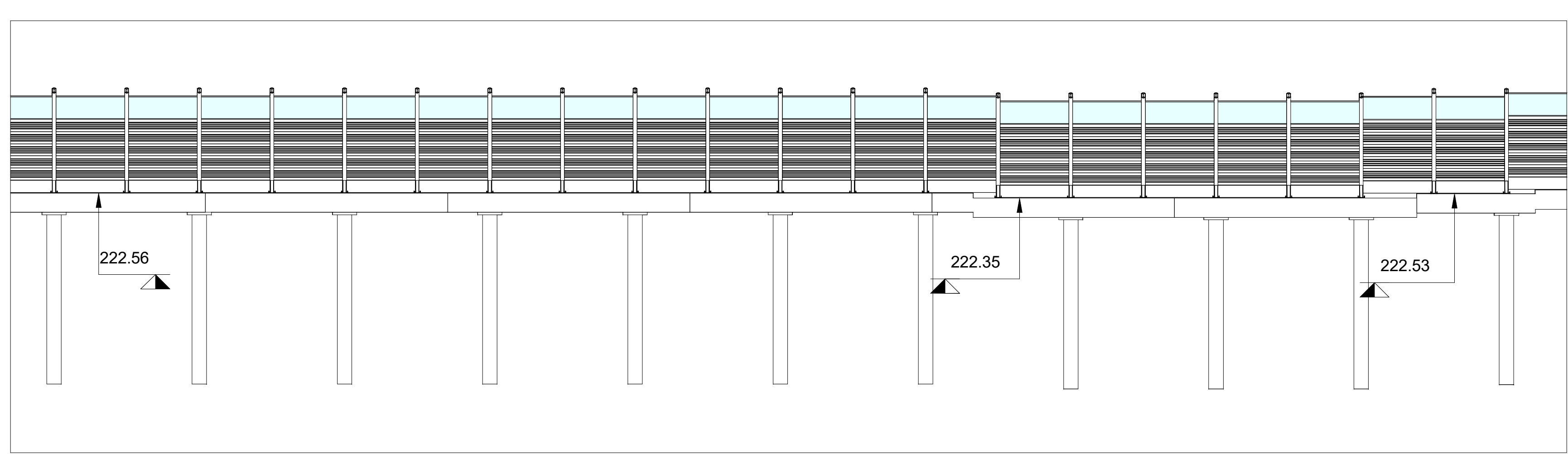
3 Sezione WBS 28 pt5 1 : 200
