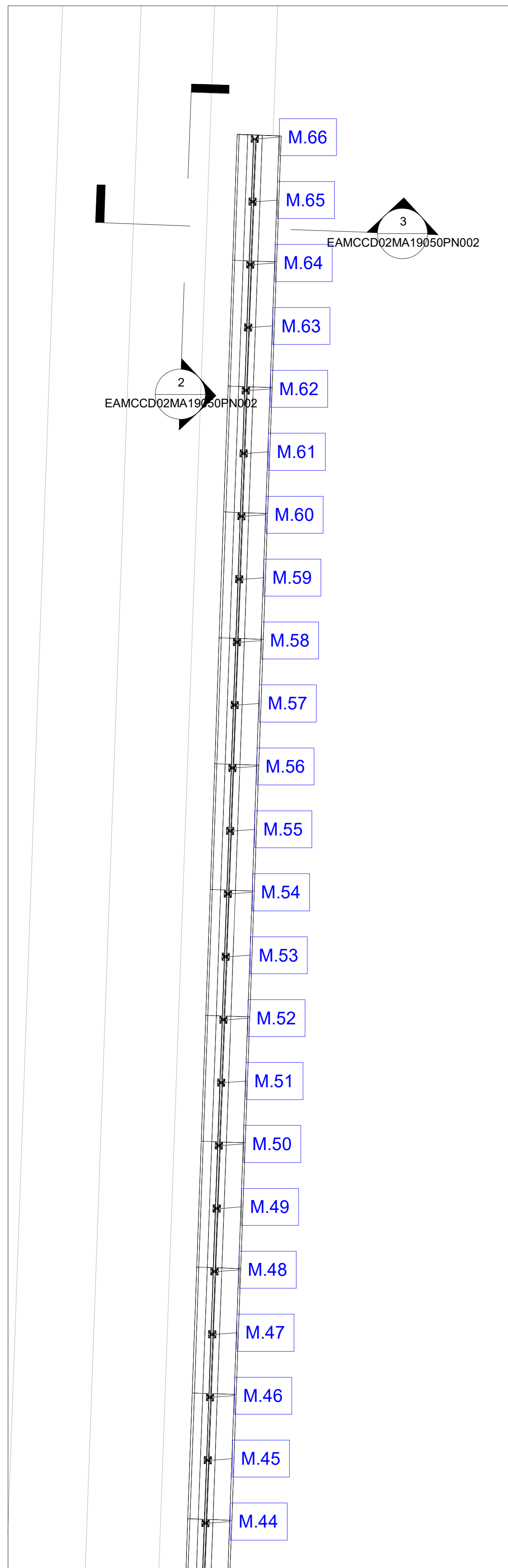
1 Stalcio Planimetrico WBS C.BA.19 pt.1 1 : 200
