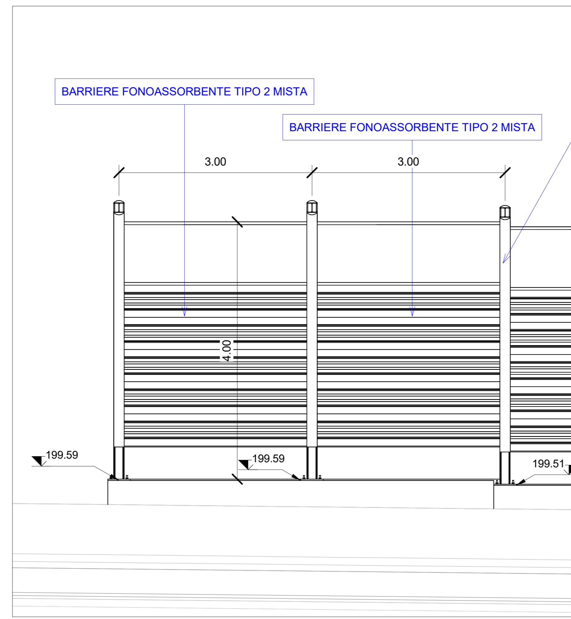
2 Sezione tipologica 1 : 50
