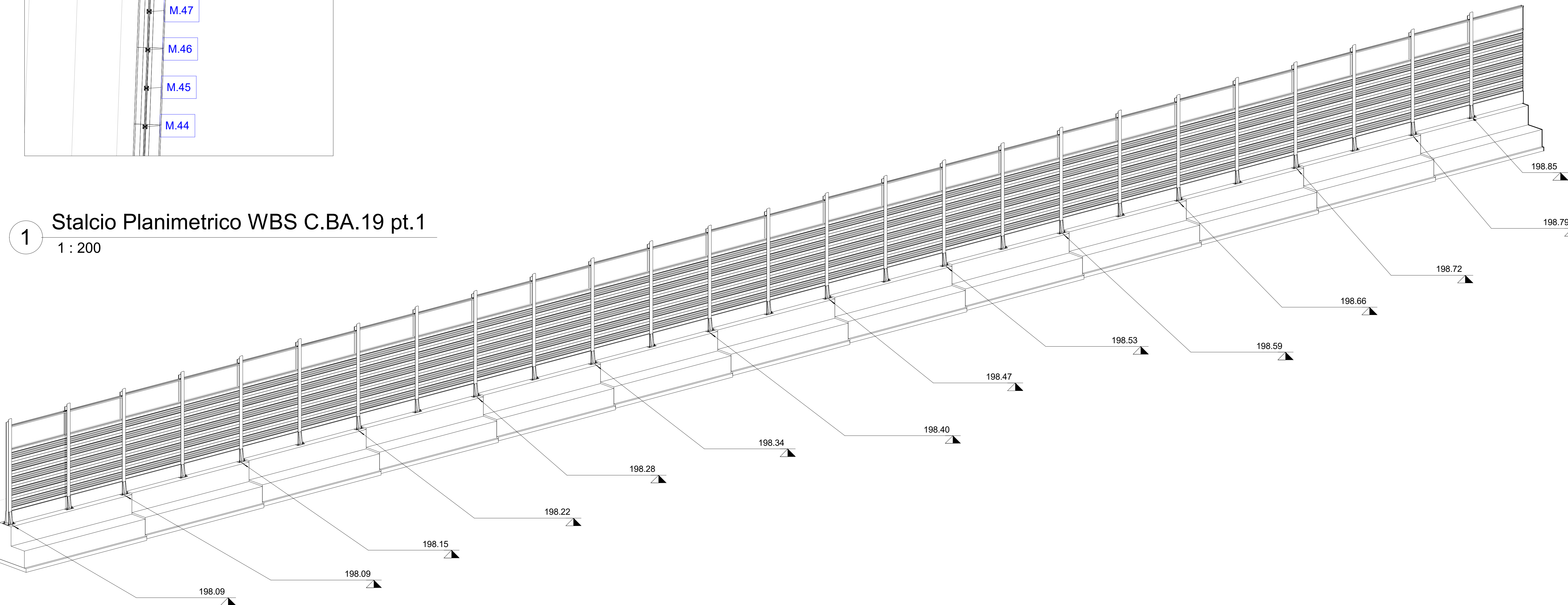
4 Assonometria WBS C.BA.19 pt.1
