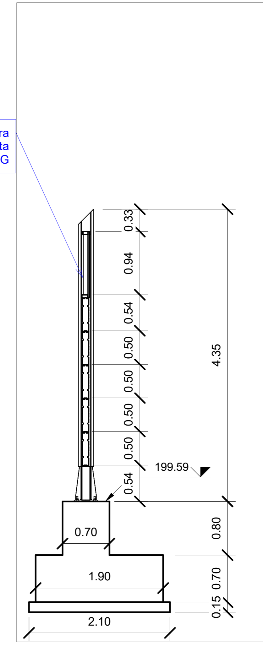
3 Sezione tipologica 1 : 50
