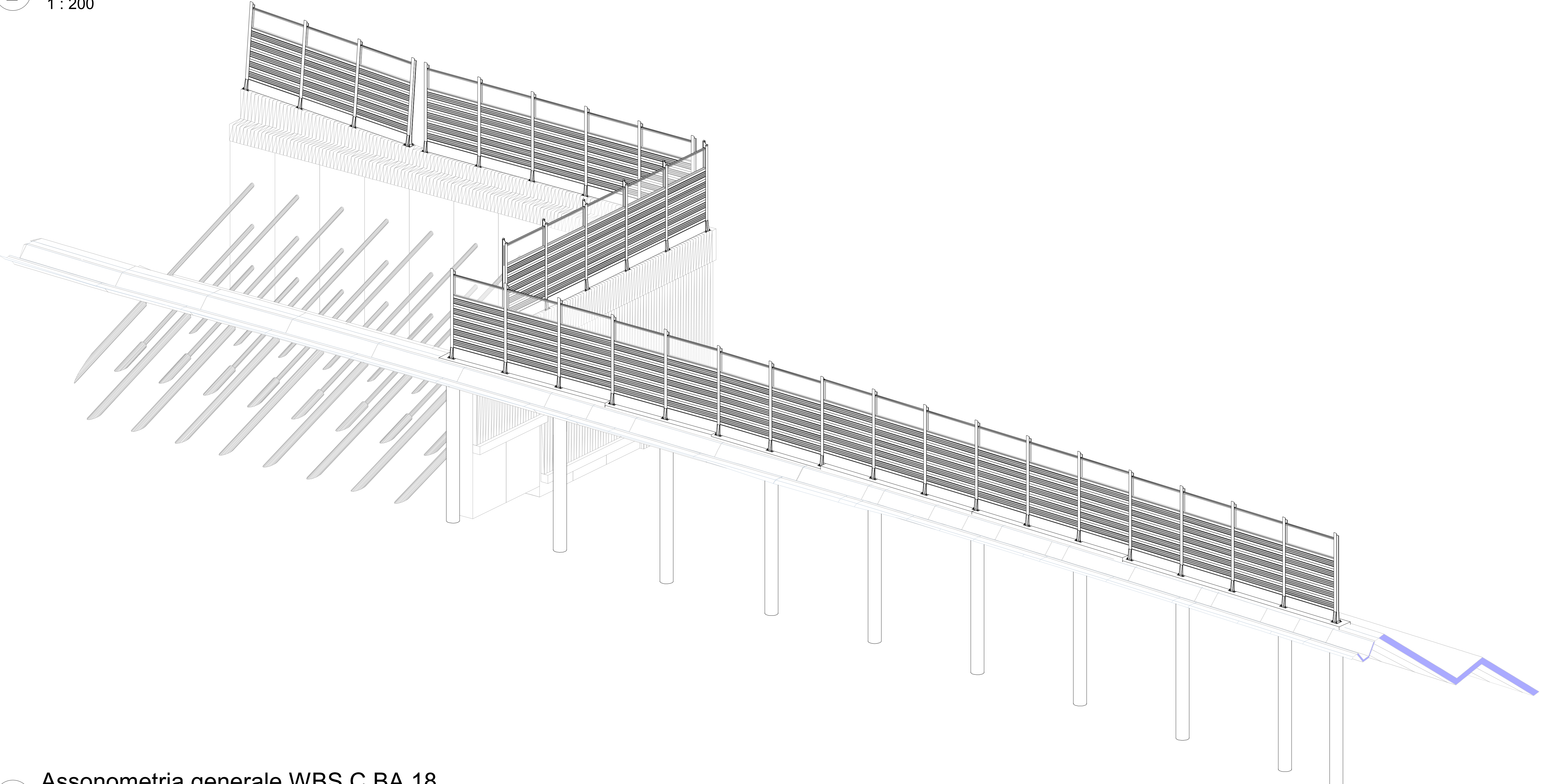
3 Assonometria generale WBS C.BA.18
