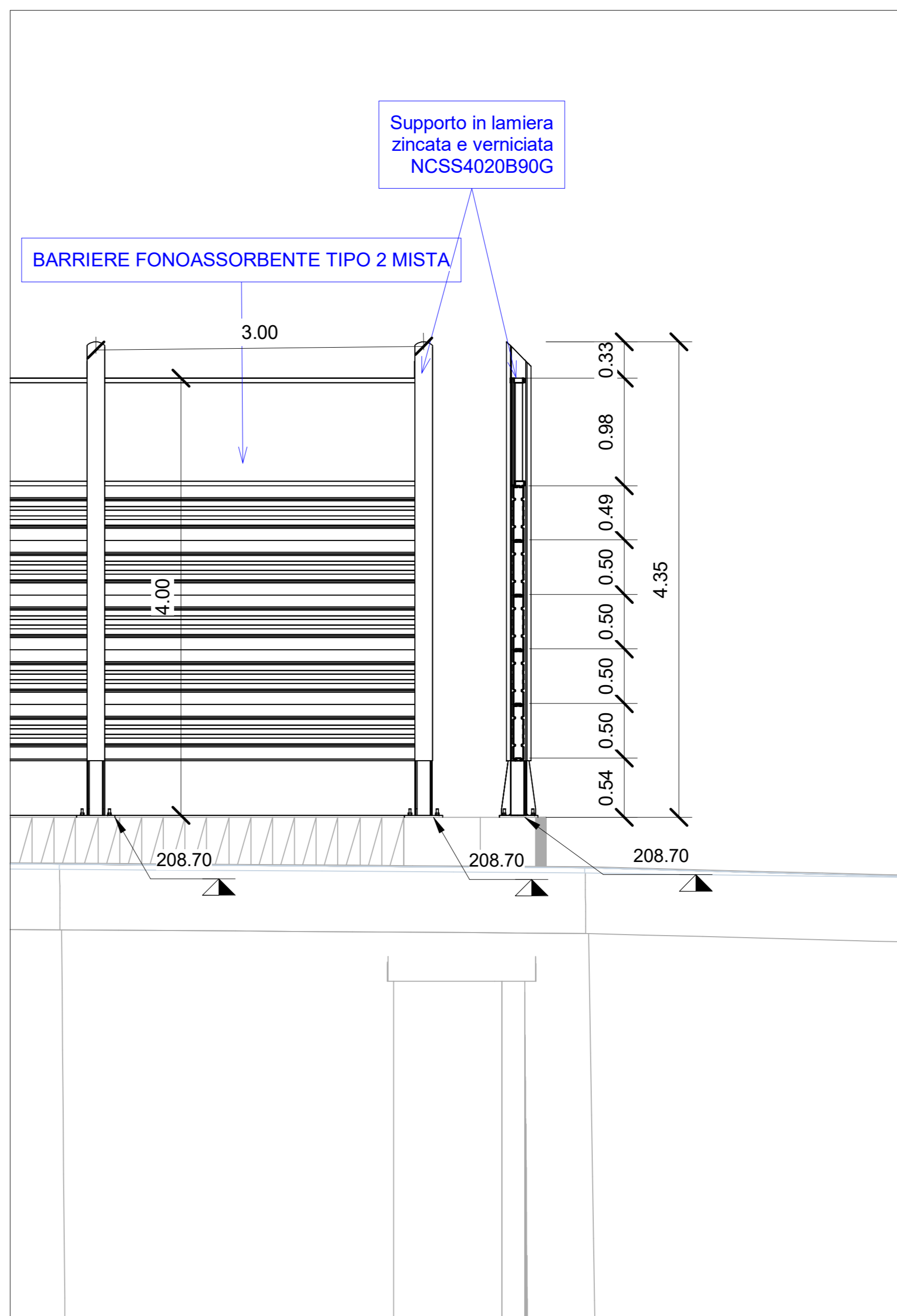
2 Sezione tipologica 1 : 50
