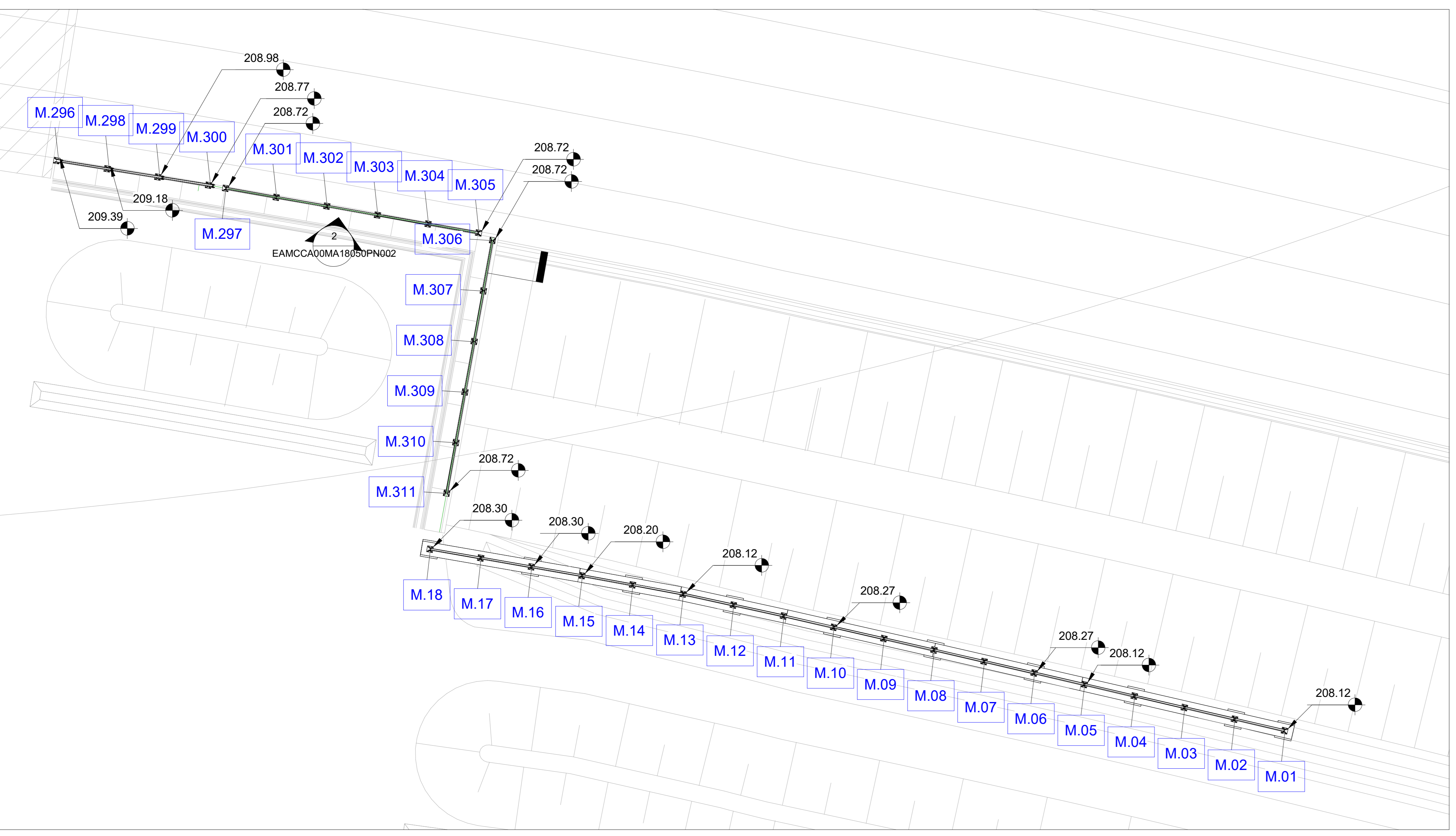
1 Stalcio Planimetrico WBS C.BA.18 1 : 200
