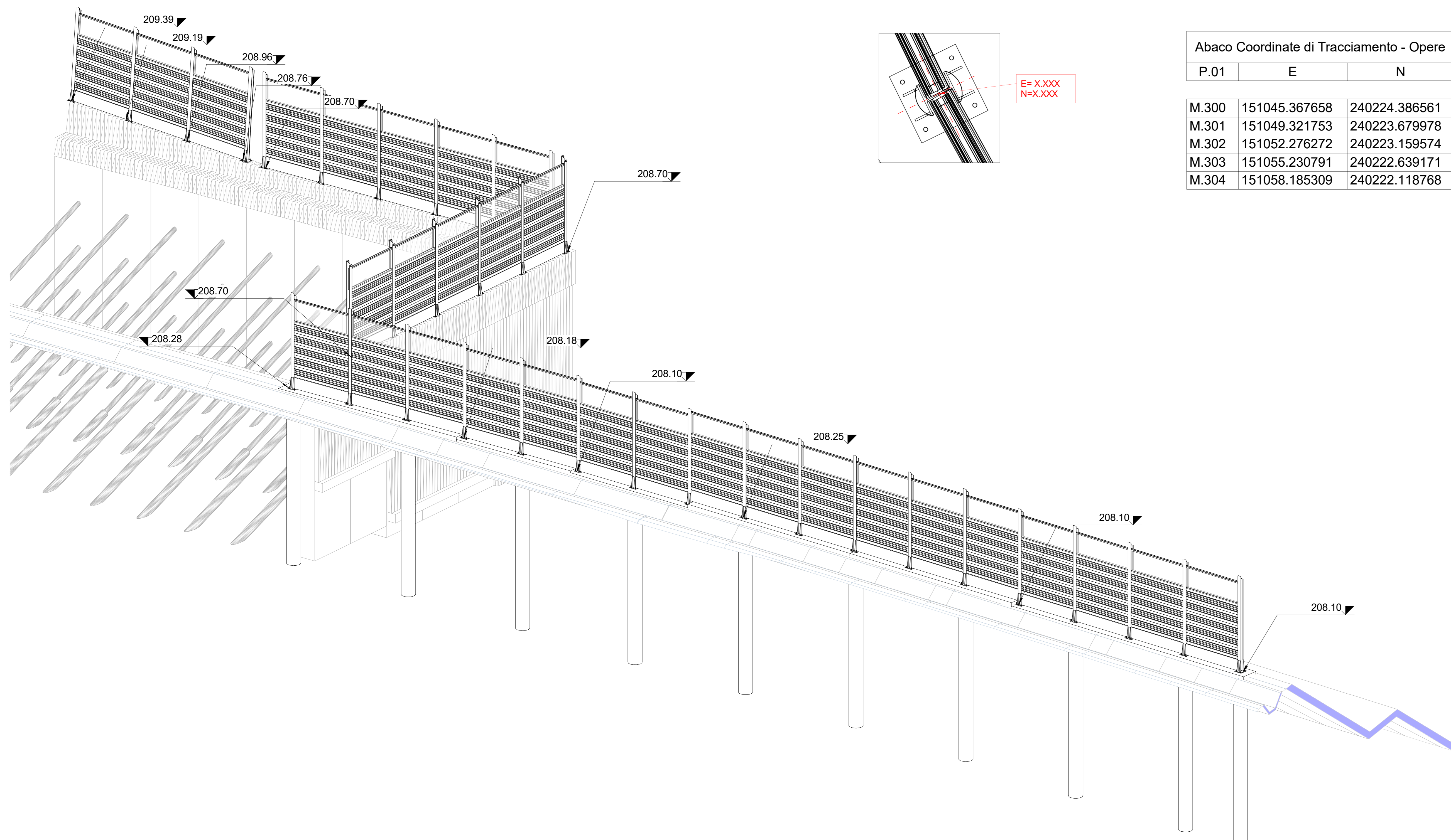
3 Assonometria WBS C.BA.18 pt.1
