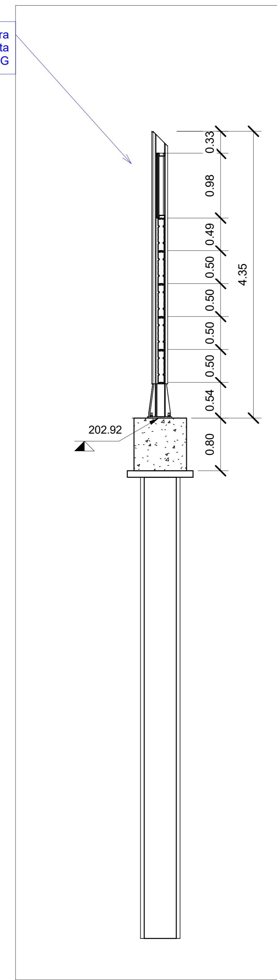
3 Sezione tipologica 1 : 50
