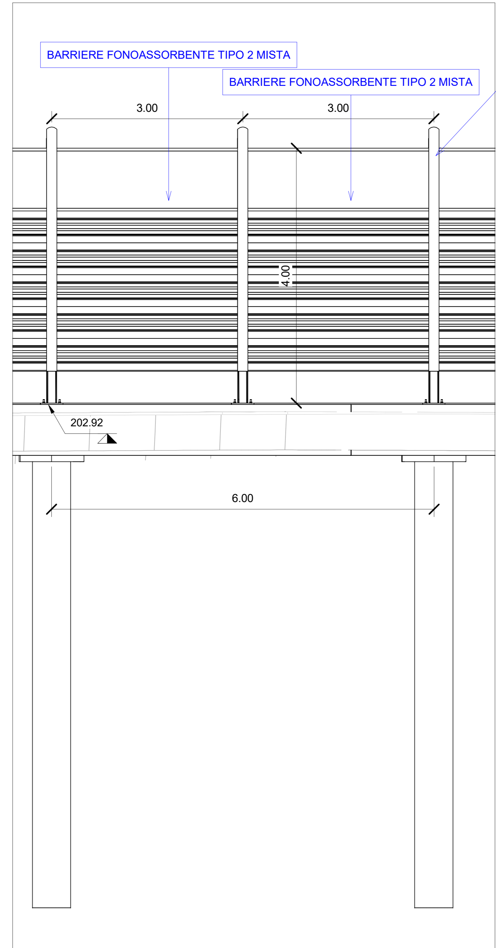
2 Sezione tipologica 1 : 50
