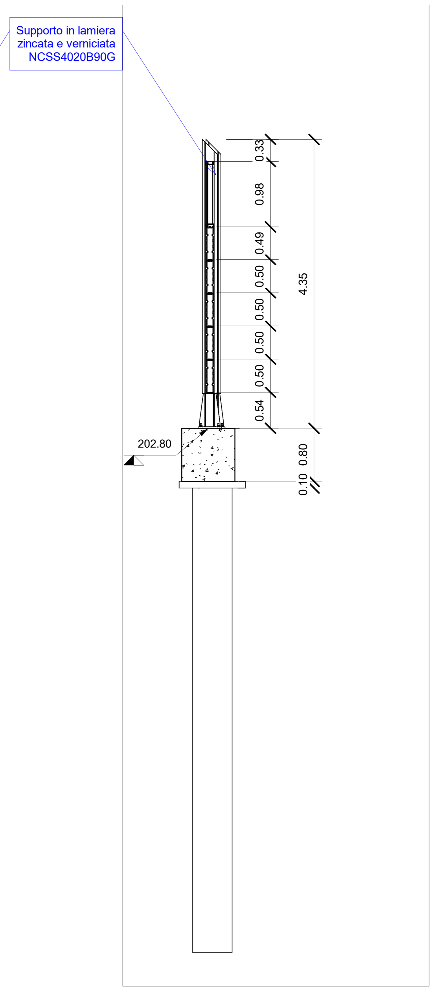
3 Sezione tipologica 1 : 50
