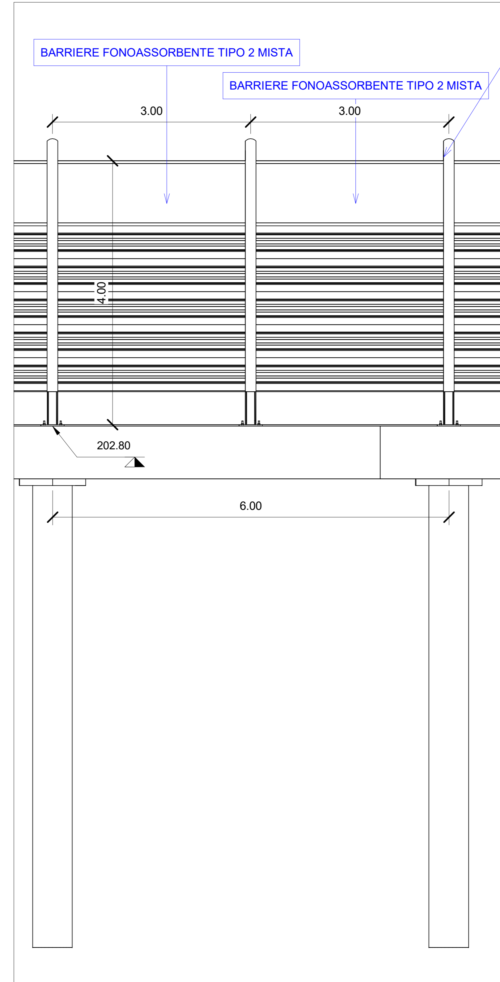
4 Sezione tipologica 1 : 50
