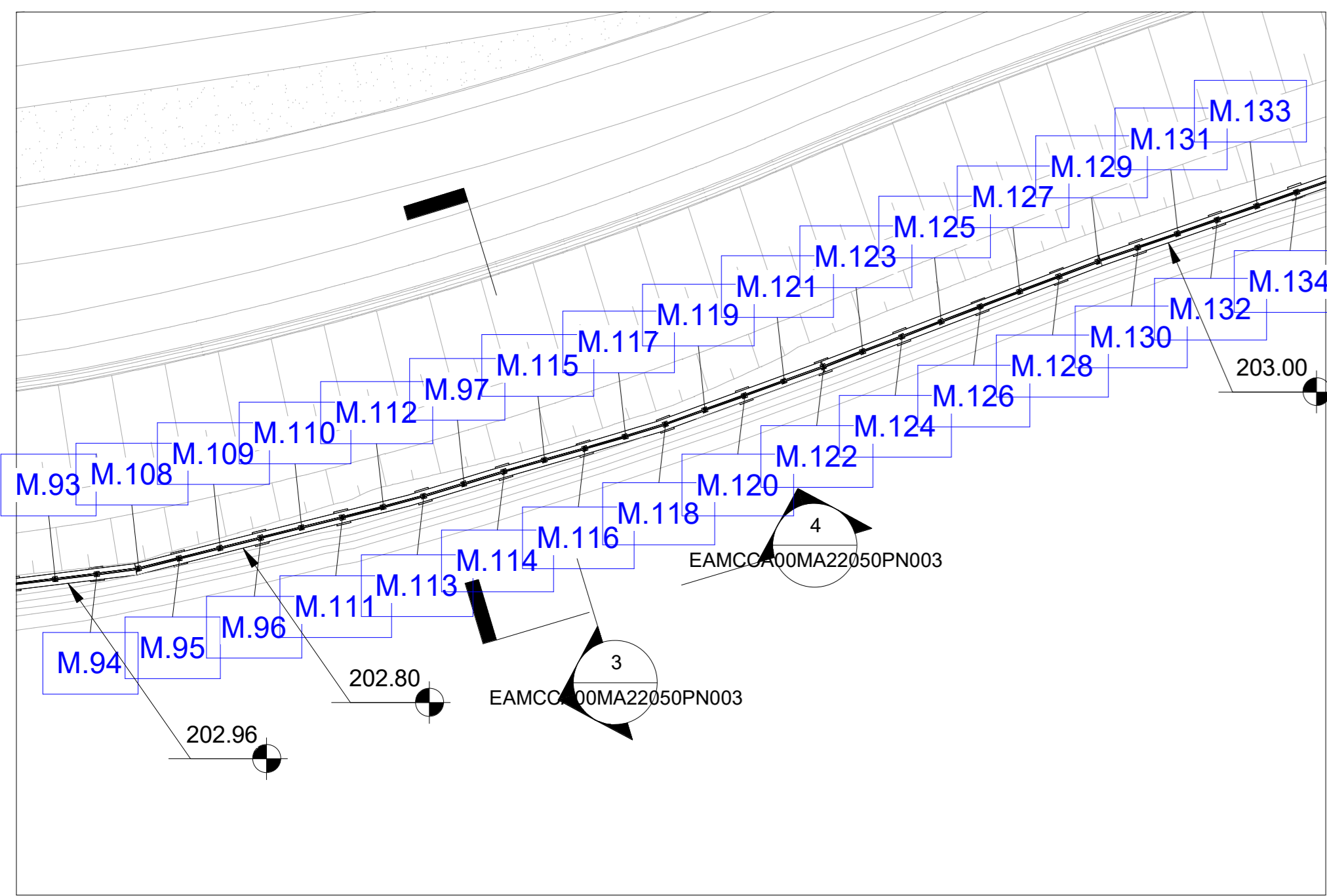
1 Stalcio Planimetrico WBS C.BA.22 pt.2 1 : 500
