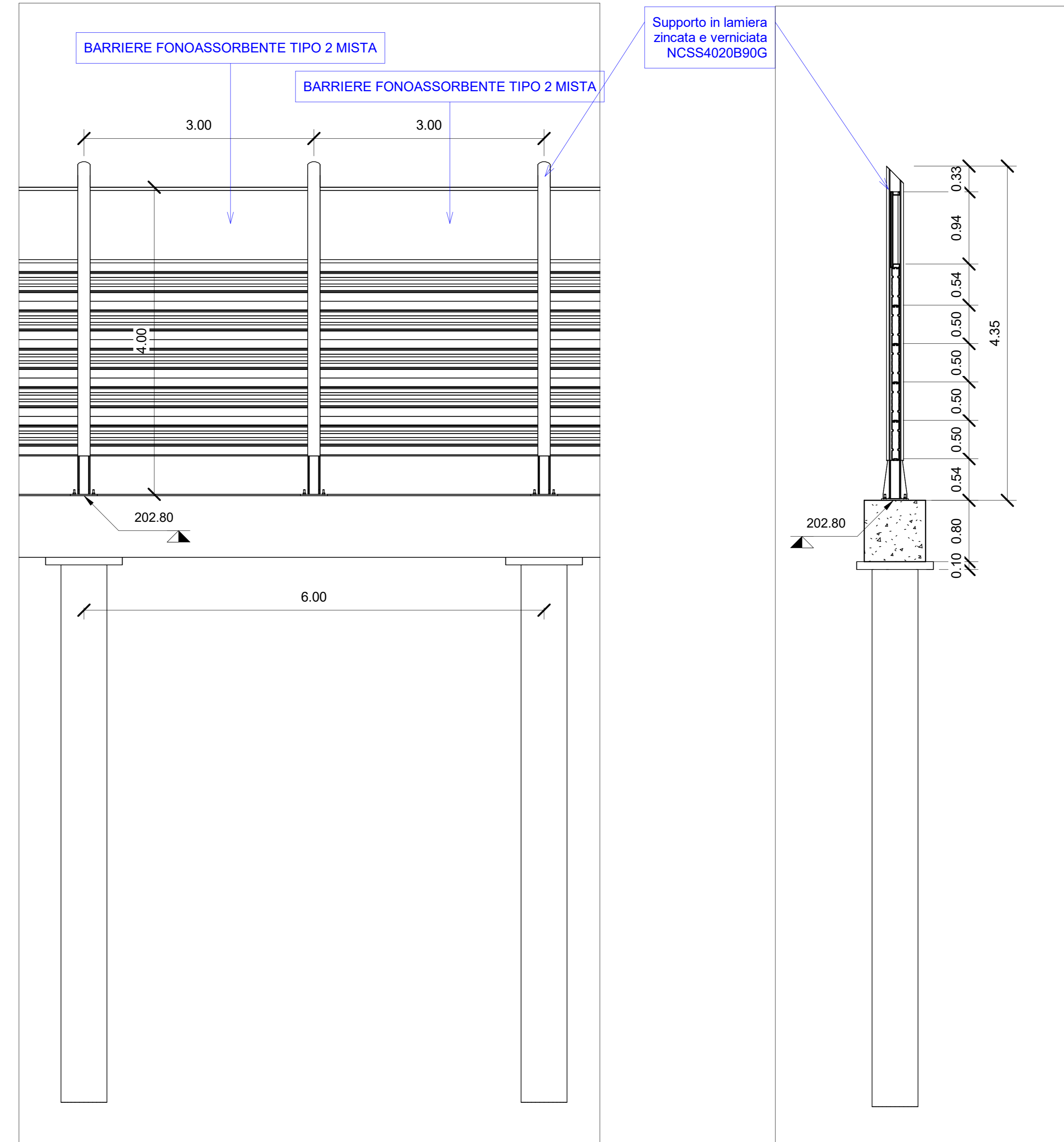
2 Sezione tipologica 1 : 50
