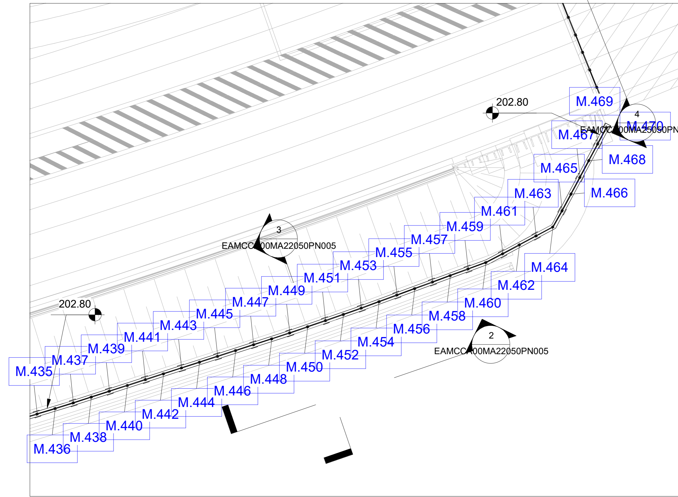
1 Stalcio Planimetrico WBS C.BA.22 pt.4 1 : 50
