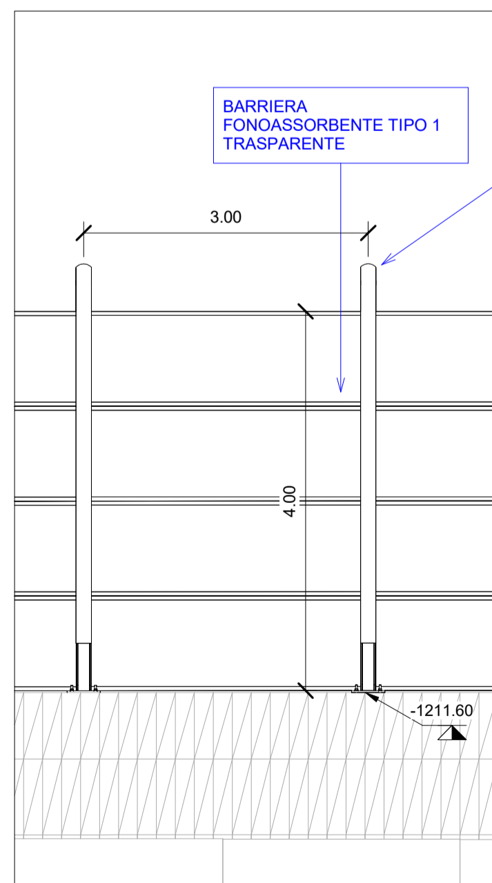
2 Sezione tipologica 1 : 50
