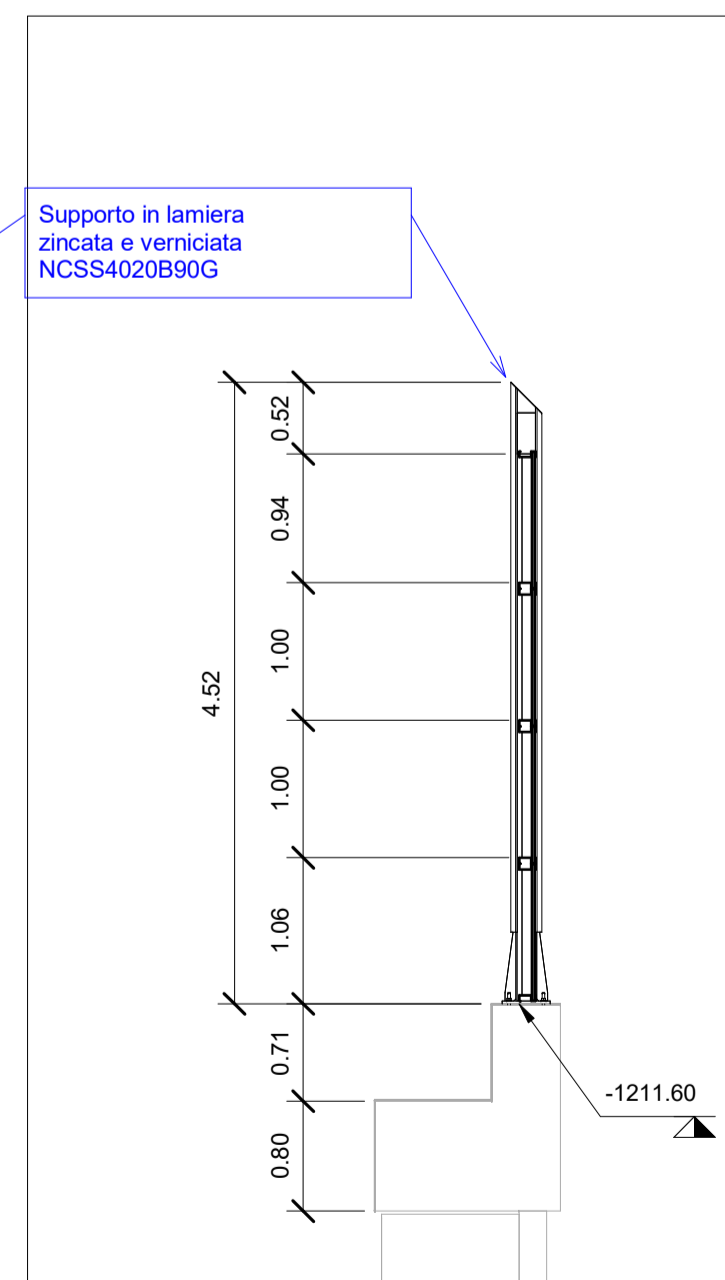
3 Sezione tipologica 1 : 50
