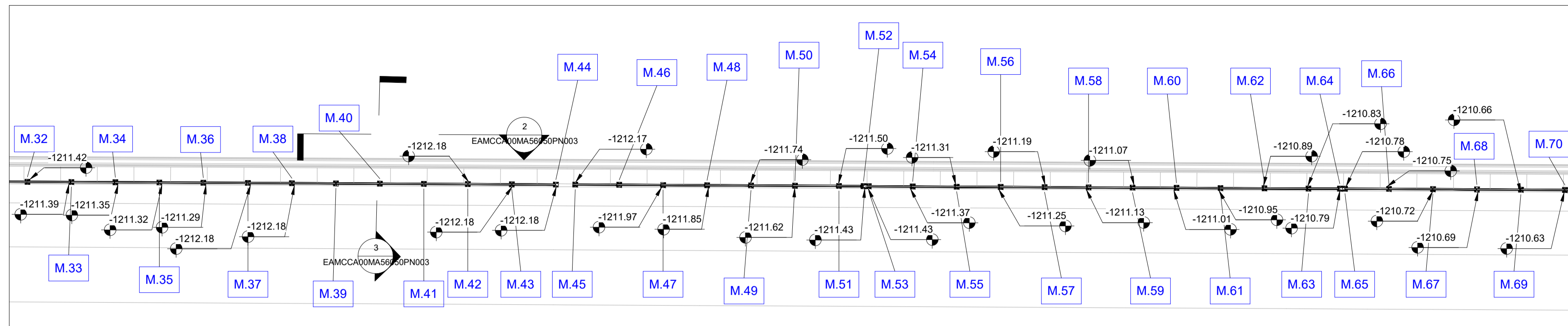
1 Stalcio Planimetrico WBS C.BA.56 pt.2 1 : 200
