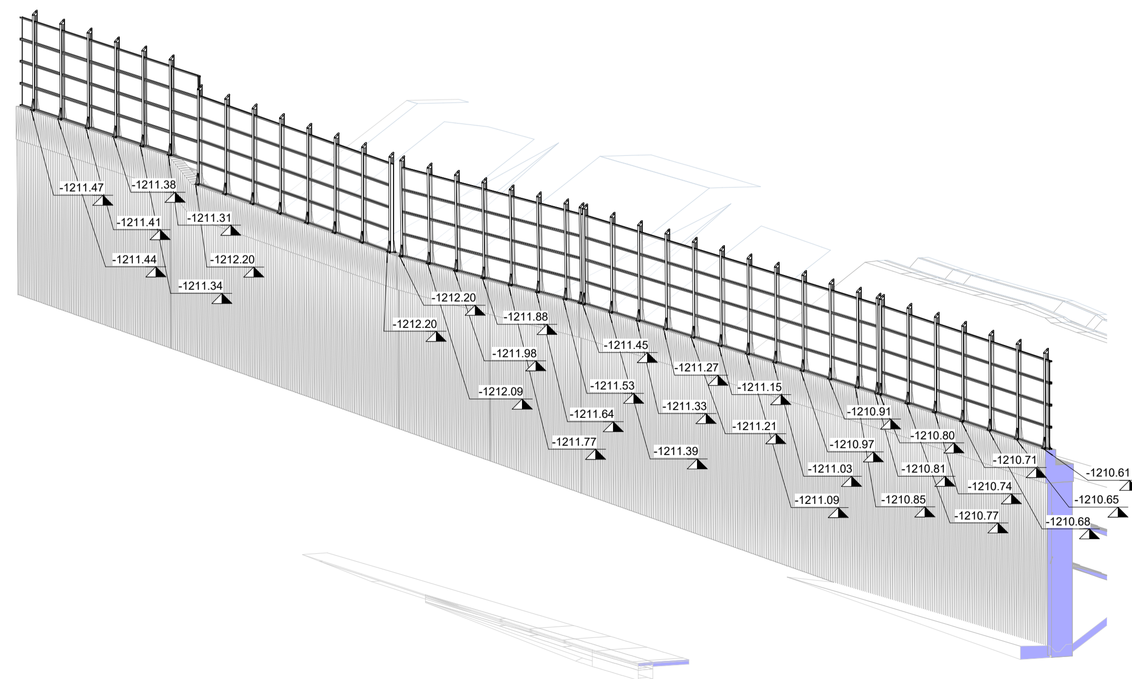
3 Assonometria WBS C.BA.56 pt.2
