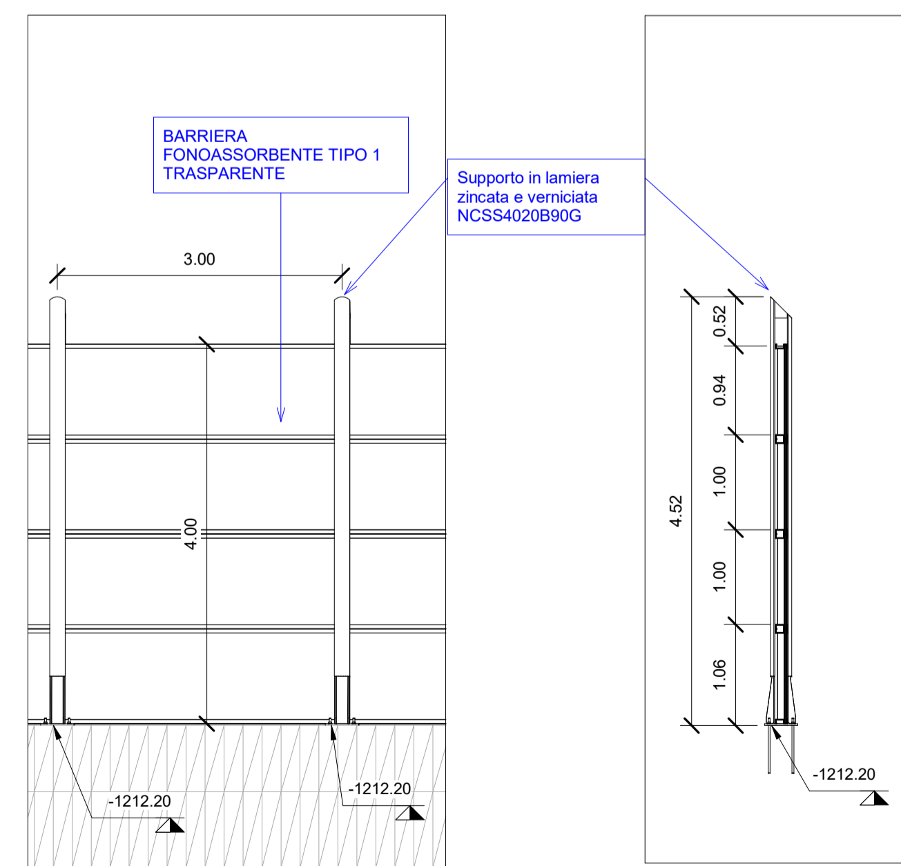
2 Sezione tipologica 1 : 50
