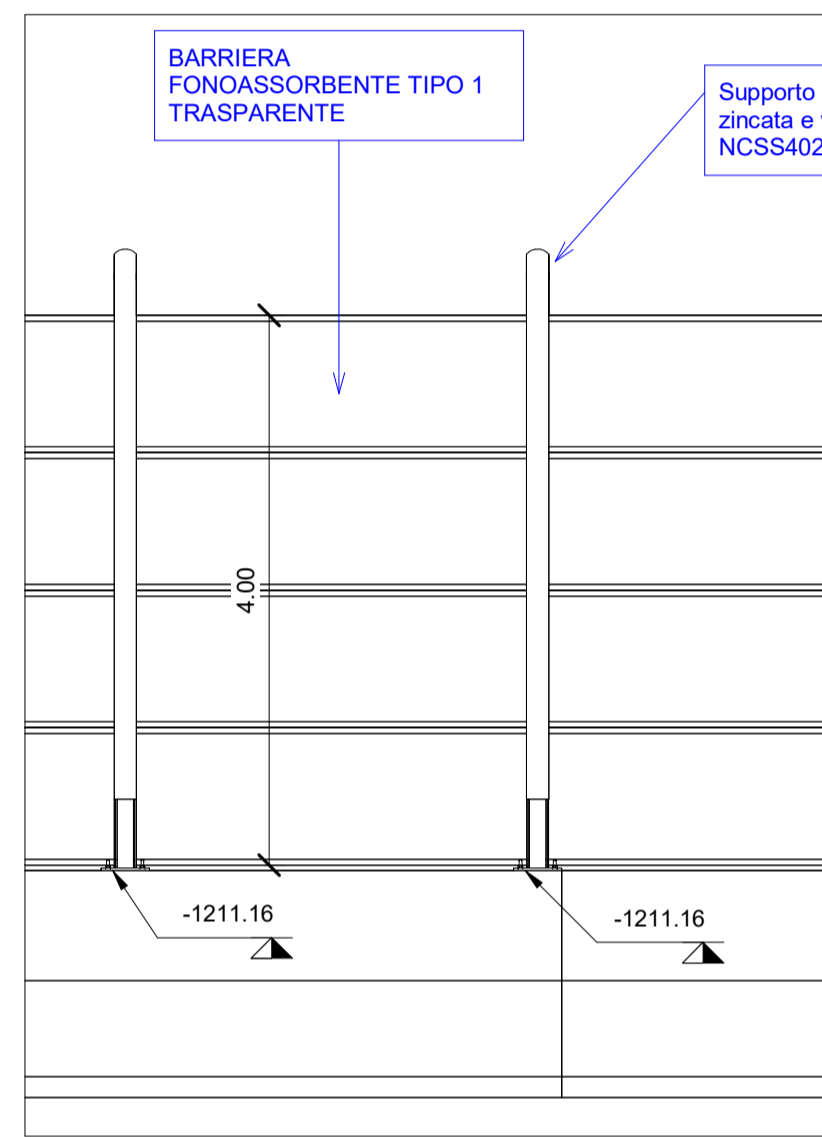
2 Sezione tipologica 1 : 50
