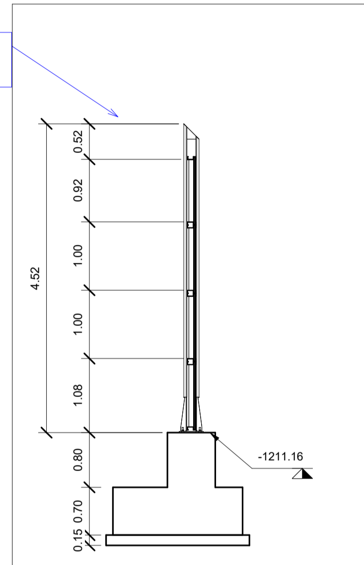
3 Sezione tipologica 1 : 50
