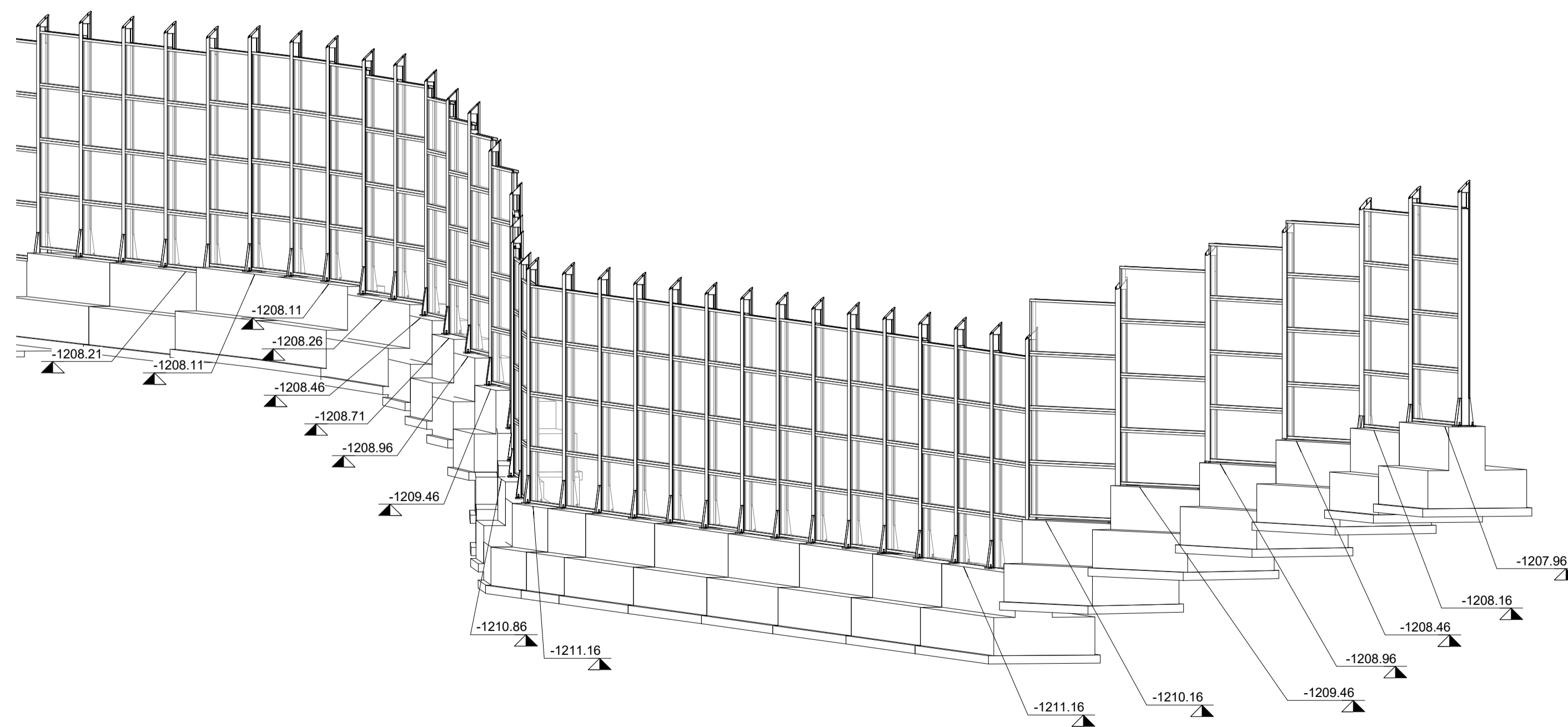
4 Assonometria WBS C.BA.57 pt.6
