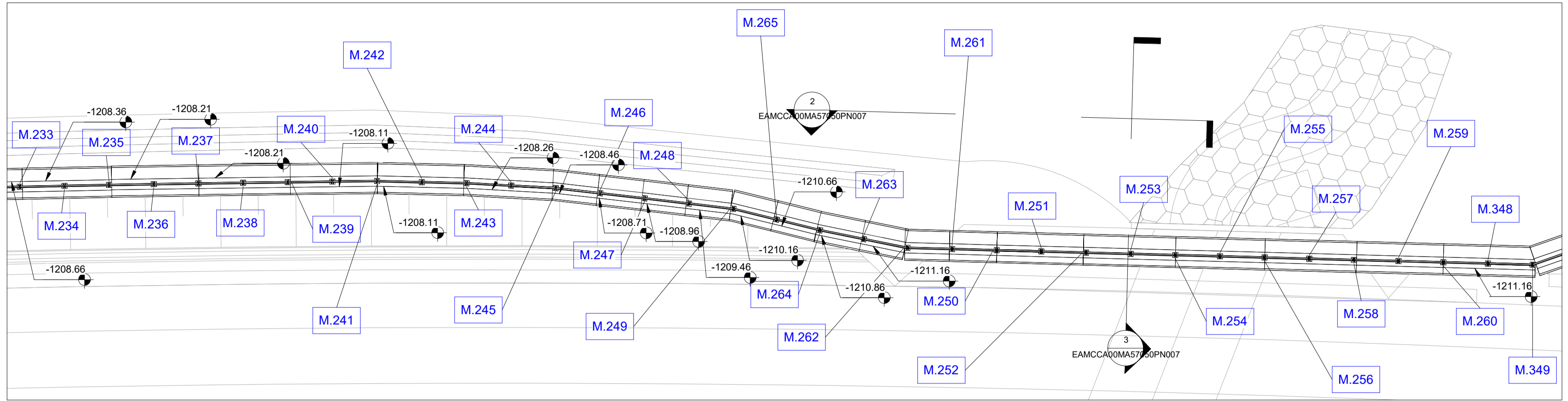
1 Stalcio Planimetrico WBS C.BA.57 pt.6 1 : 200
