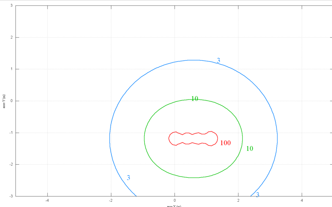
Figura 5.2: Curve isolivello d'induzione magnetica calcolate su un piano XY
