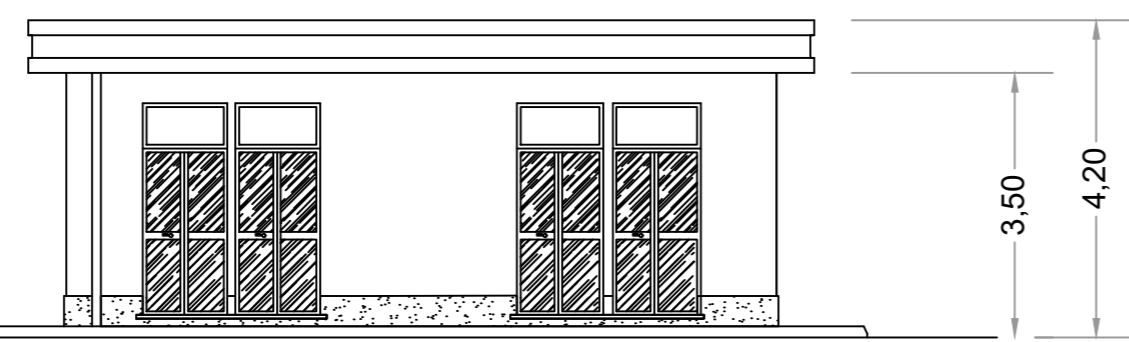
Prospetto C - C
