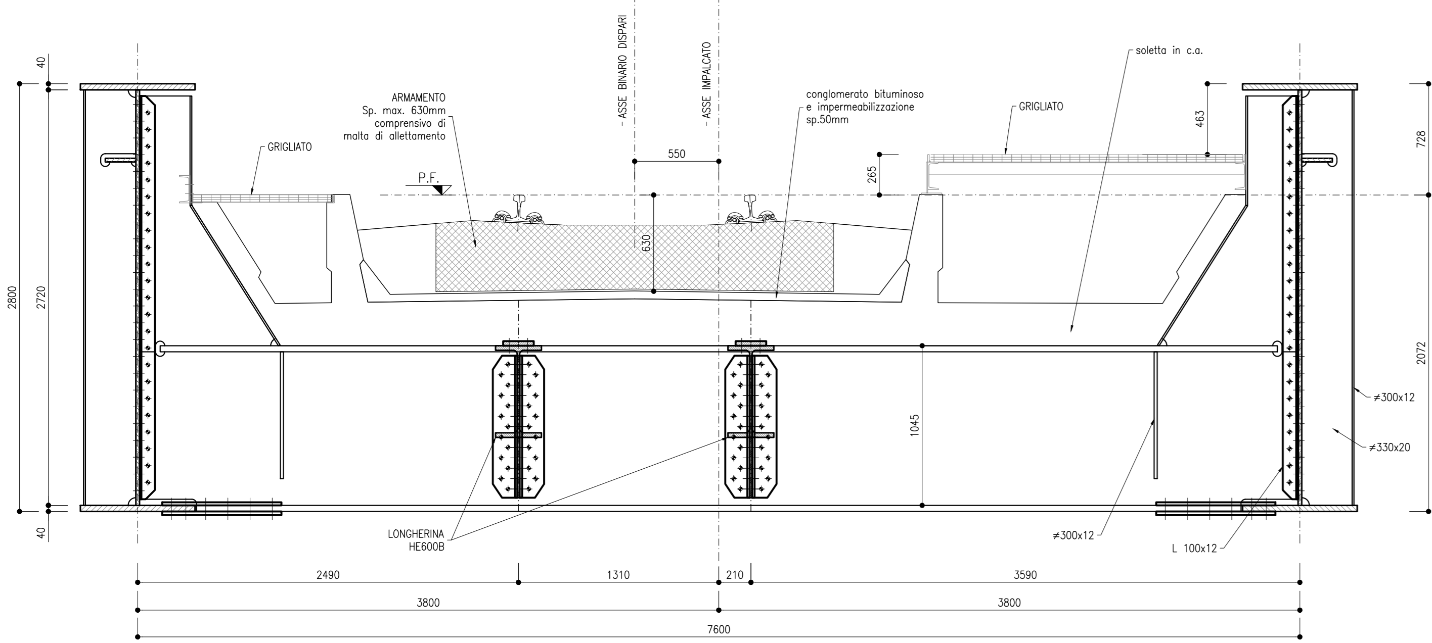
SEZIONE TIPICA TRAVE TIPO 2 SCALA 1:25
