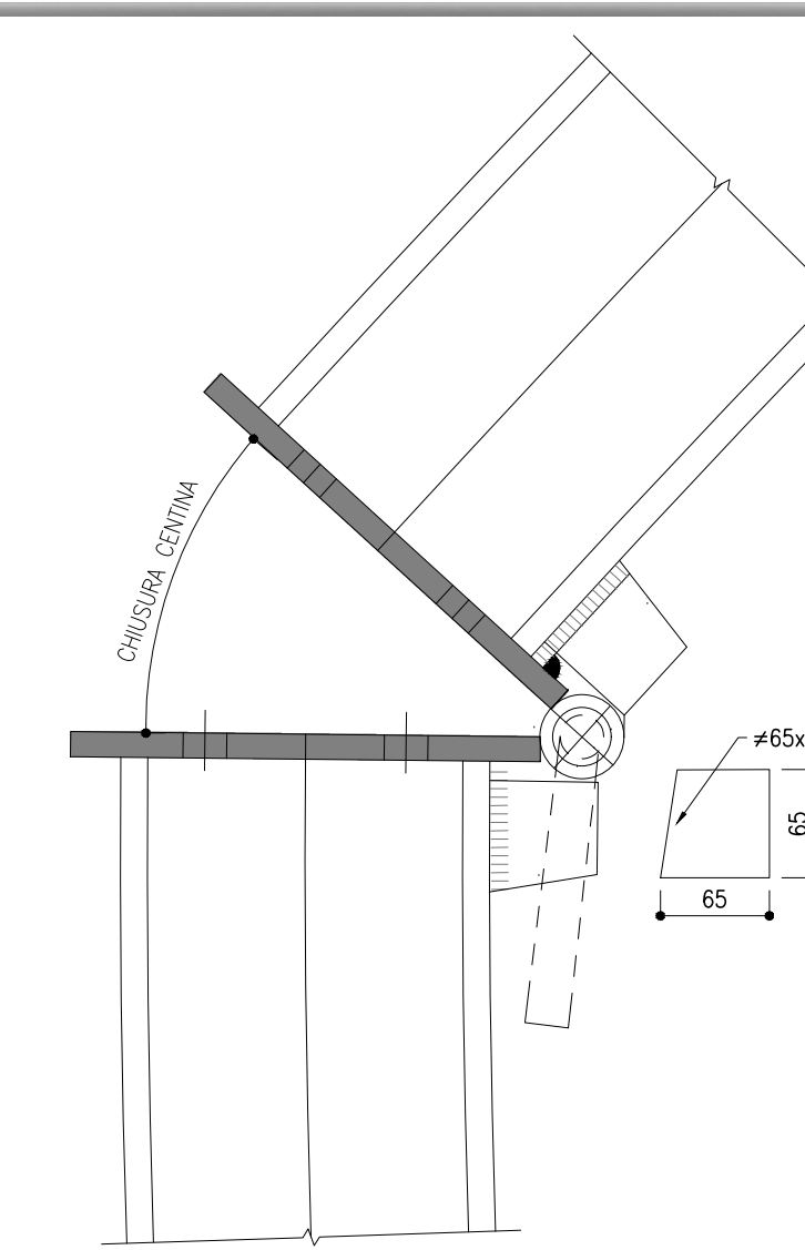
DETTAGLIO CERNIERA (Posizione iniziale) SCALA 1:5
