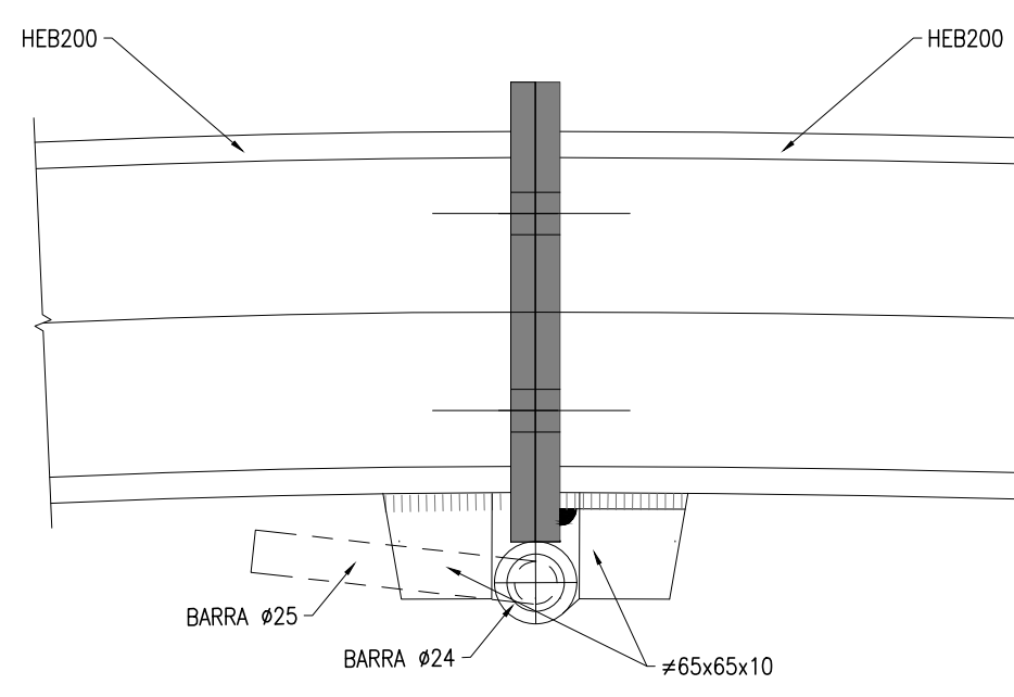
DETTAGLIO CERNIERA (Posizione finale) SCALA 1:5
