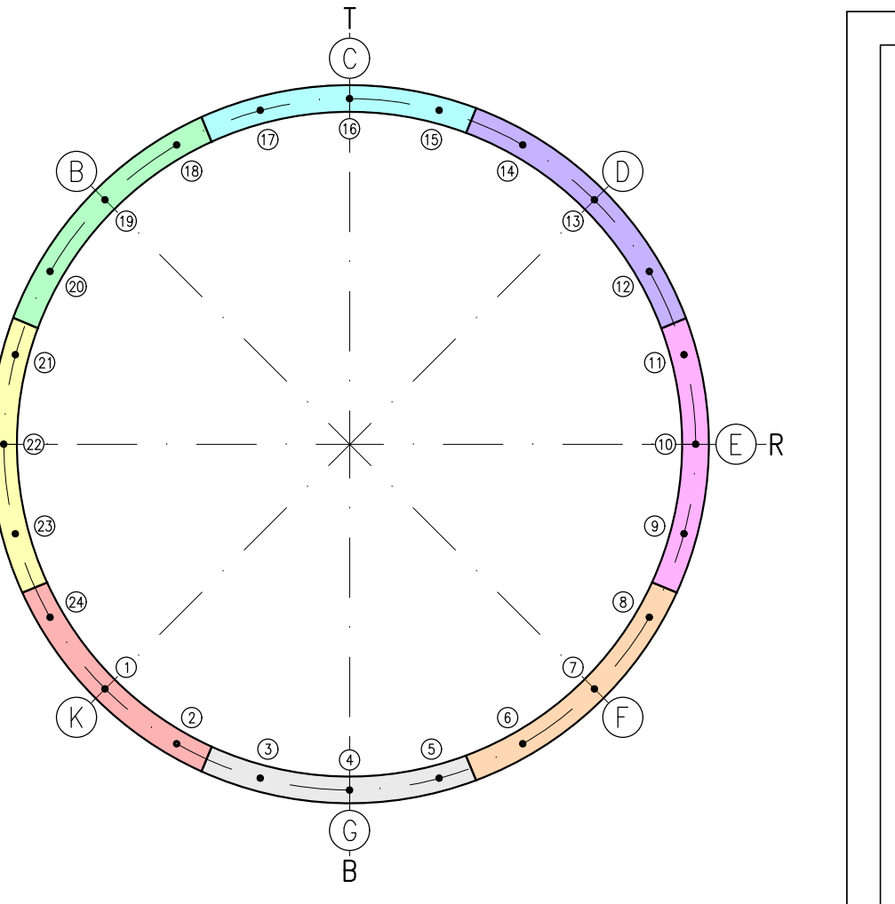
POSIZIONE 24 SCALA 1:100
