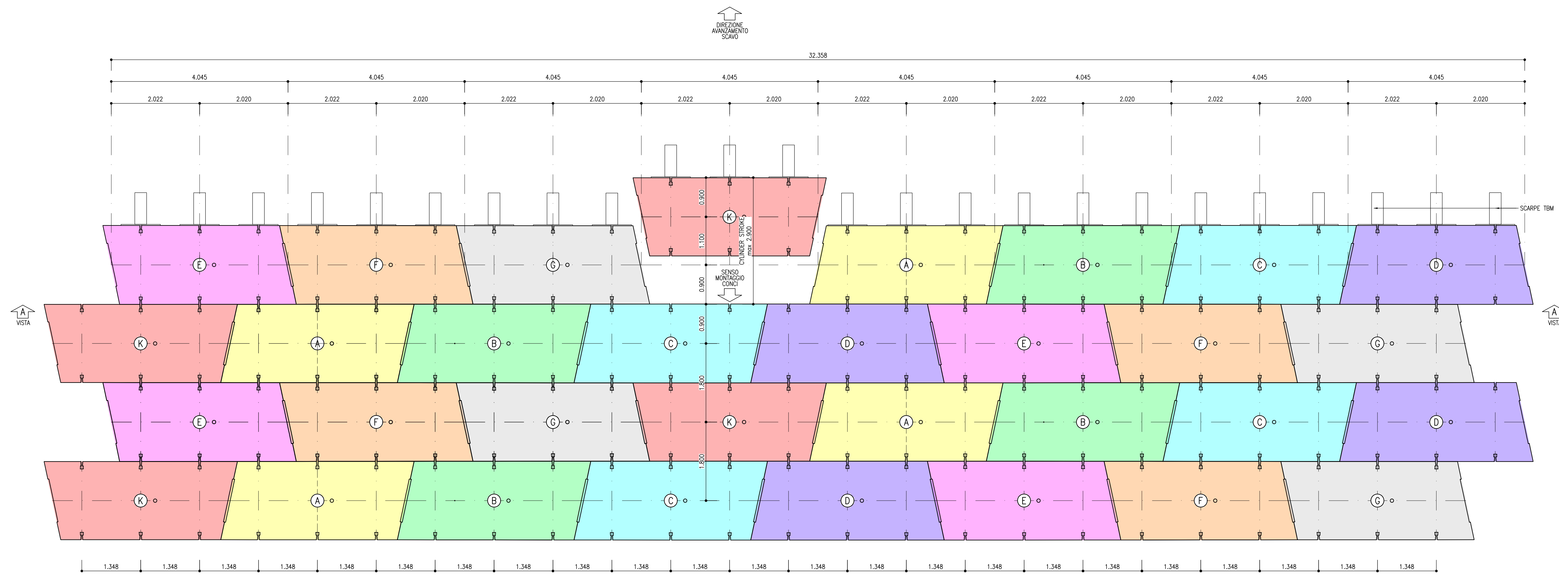
SCHEMA SVILUPPATA CONCI SCALA 1:50 (RAPPRESENTAZIONE TIPOLOGICA DI COMBINAZIONI CONSENTITE)
