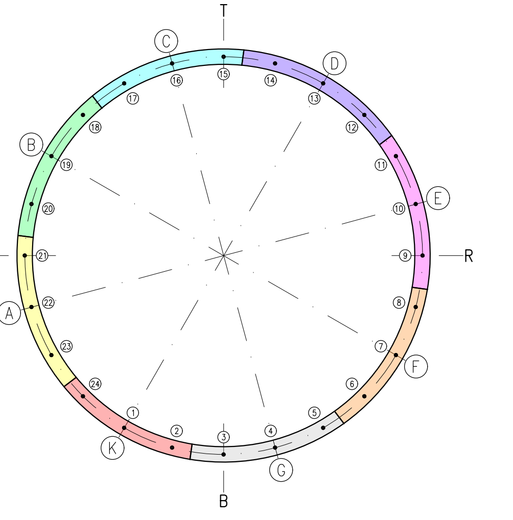
POSIZIONE 23 SCALA 1:100
