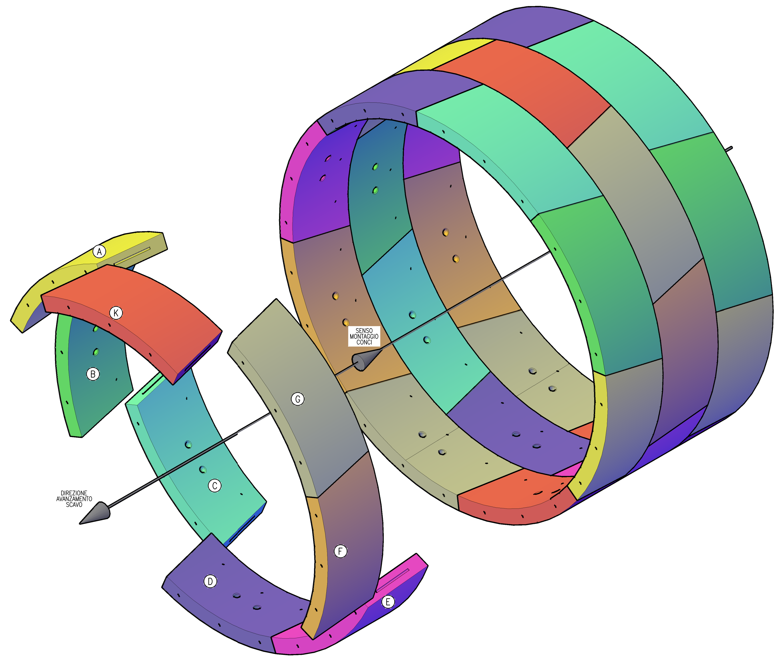
VISTA ASSONOMETRICA SCALA 1:50
