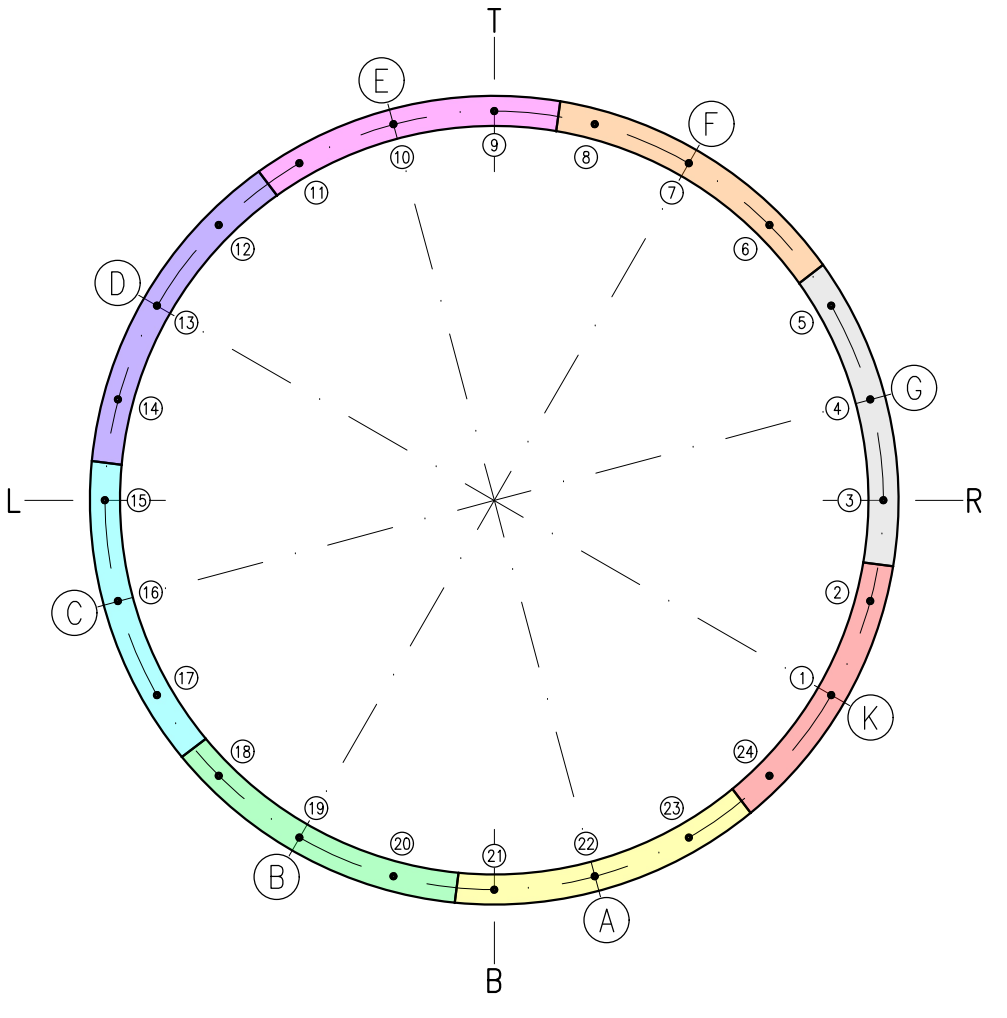
POSIZIONE 17 SCALA 1:100
