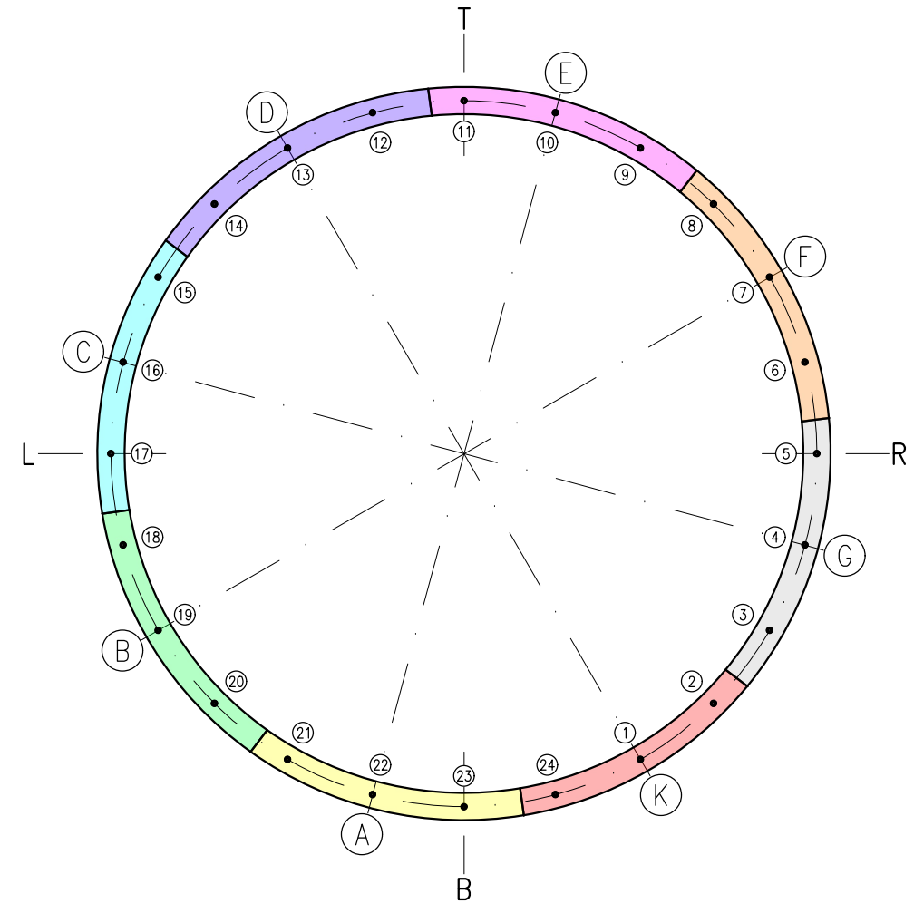
POSIZIONE 19 SCALA 1:100
