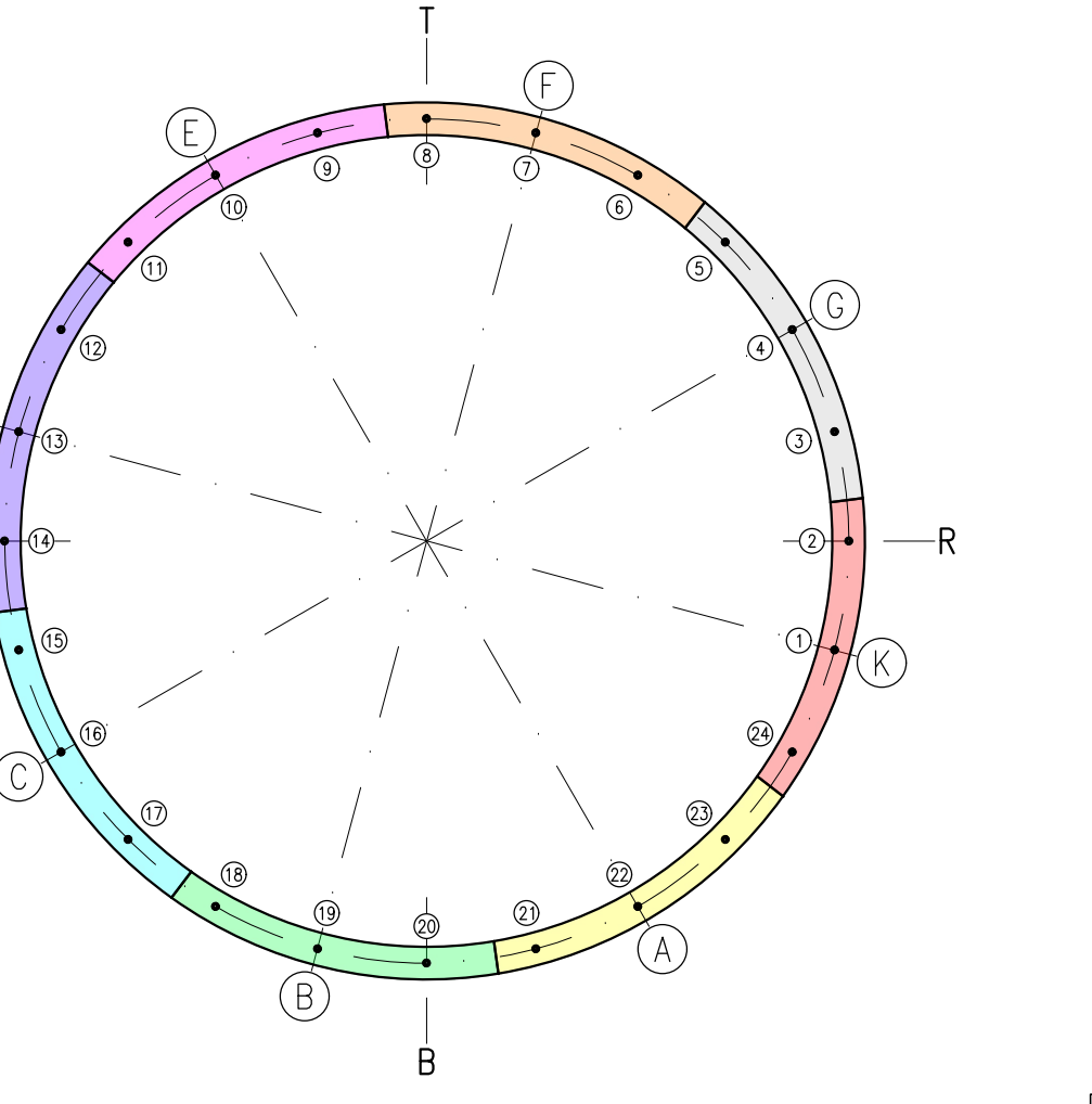
POSIZIONE 16 SCALA 1:100
