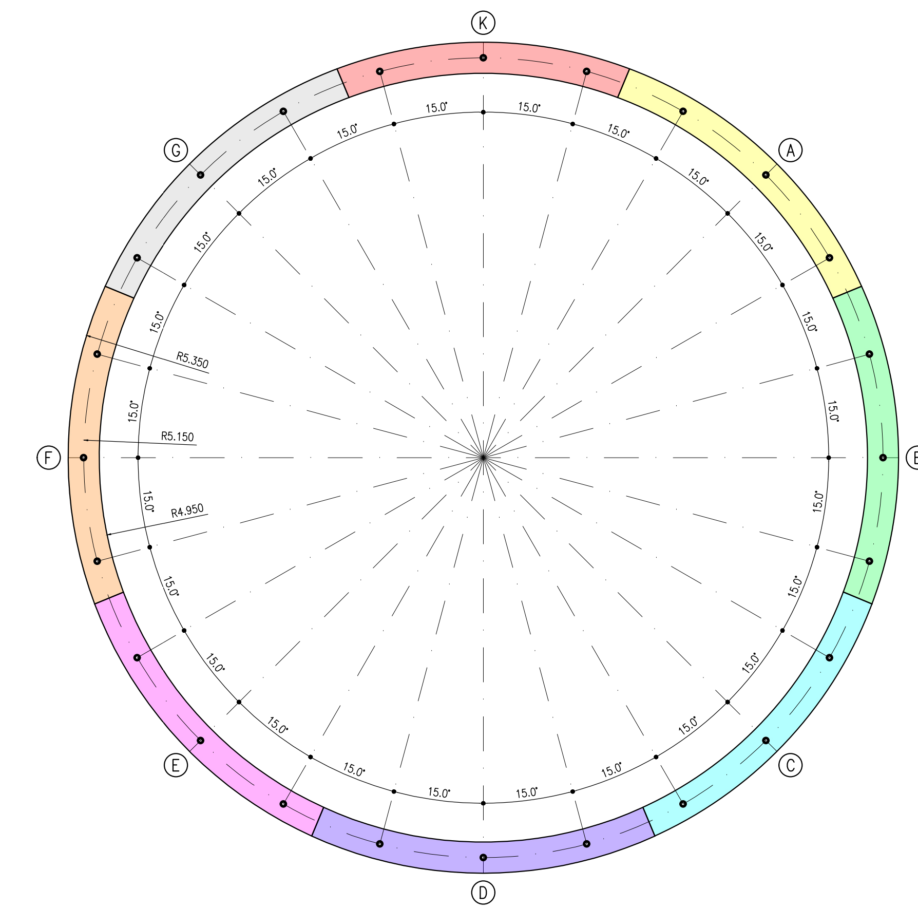
VISTA "A" SCALA 1:50
