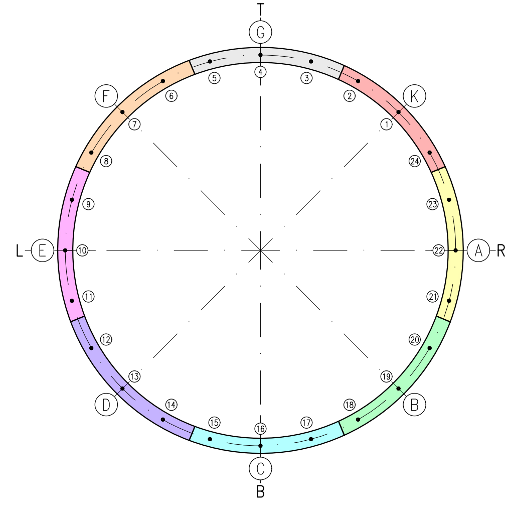
POSIZIONE 12 SCALA 1:100
