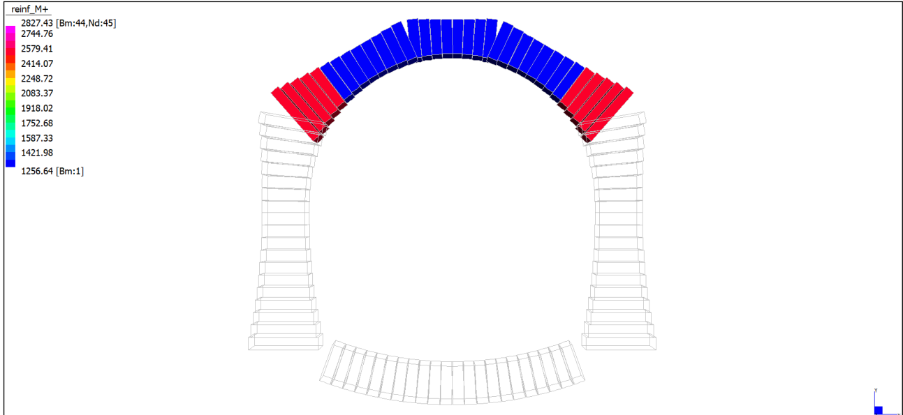
Figura 2: Armatura calotta – Strato Esterno (Lato Contro Terra)
