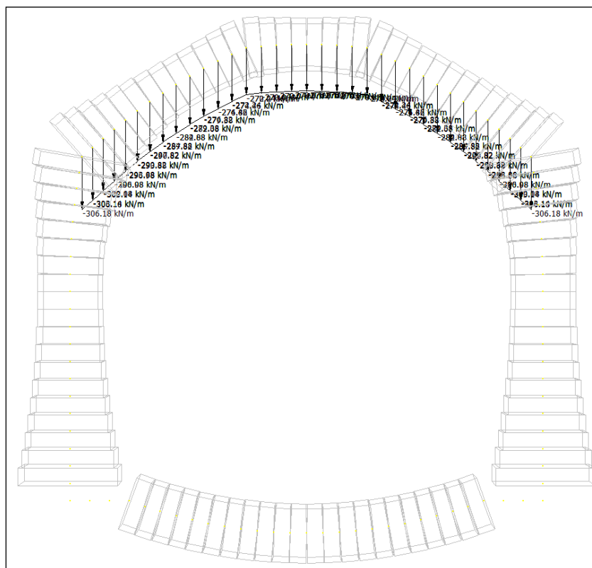
Figura 44: G01 – Peso Terreno Ricoprimento.
