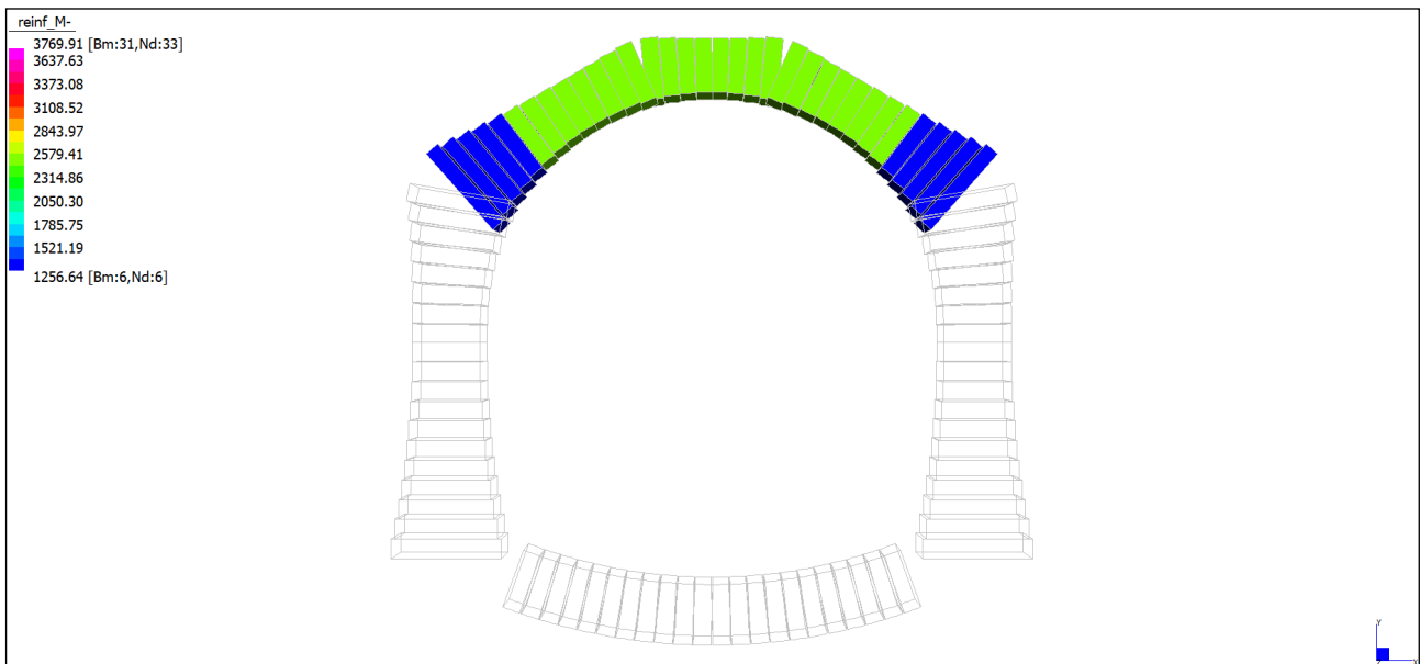
Figura 3: Armatura calotta – Strato Interno
