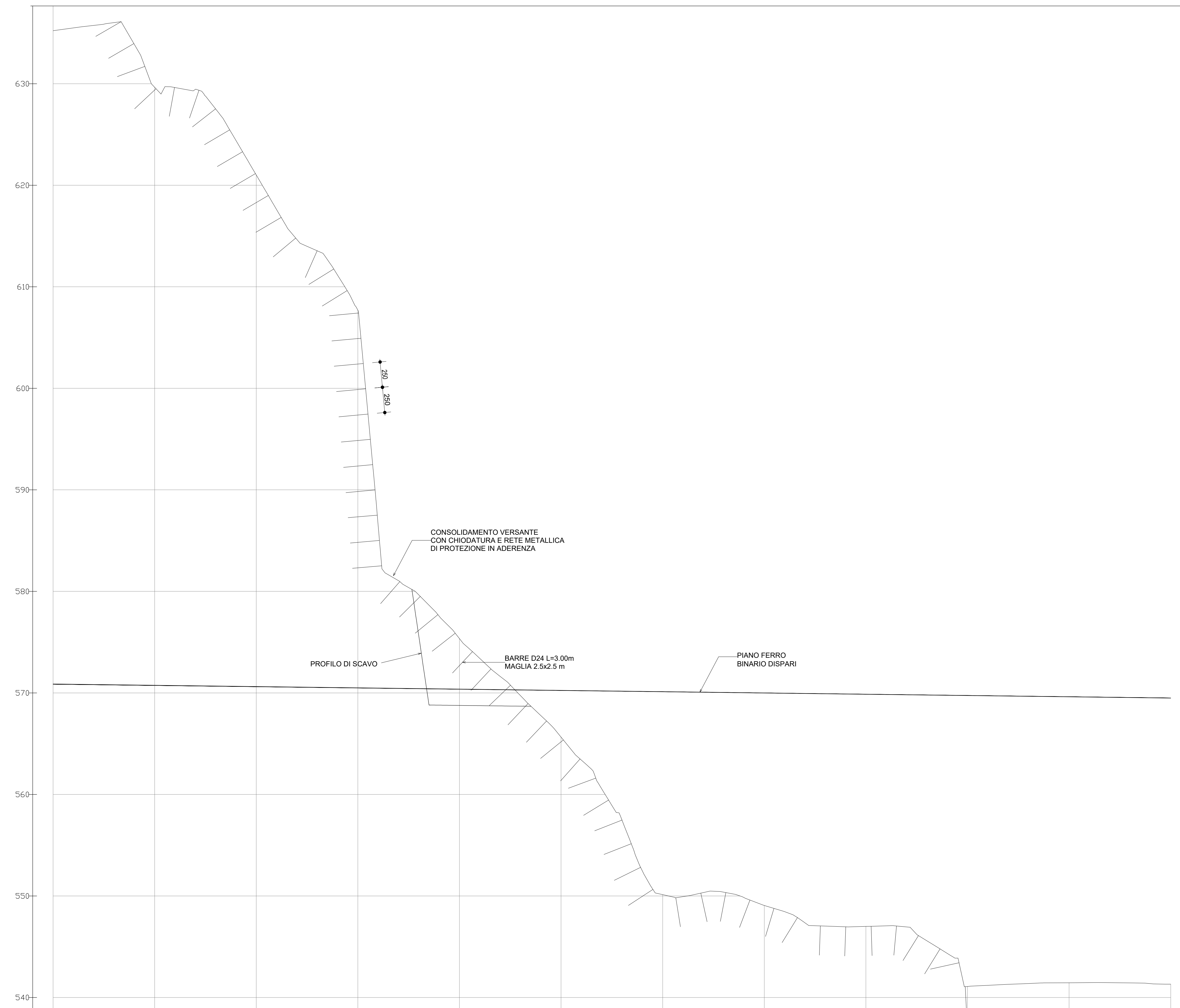
PROFILO BD SCALA 1 : 200
