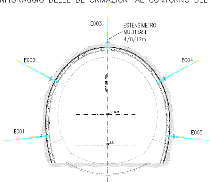
Figura 2. Ubicazione stensimetri multibase al contorno
