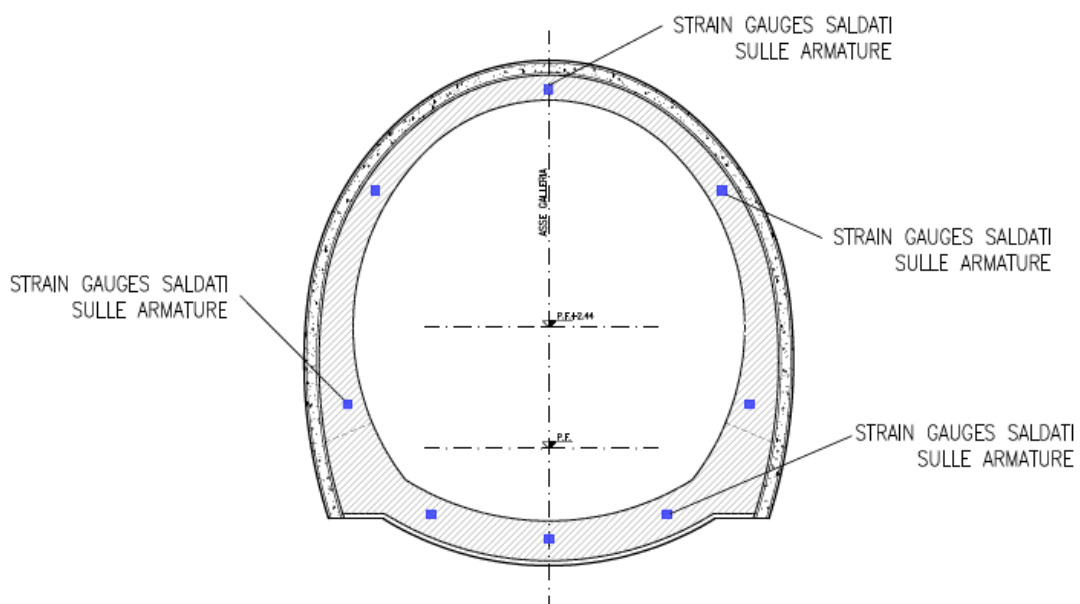
Figura 5. Ubicazione strain gauges: Rivestimento definitivo
