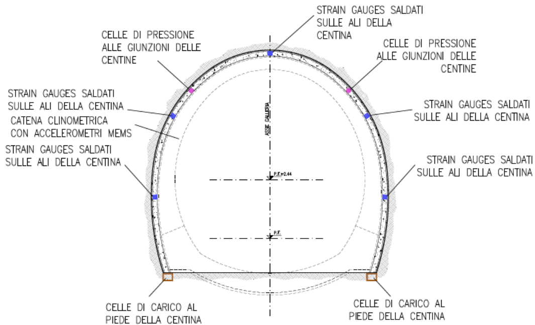
Figura 4. Ubicazione strain gauges: Rivestimento di prima fase
