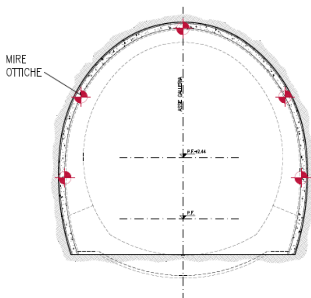
Figura 1. Ubicazione mire ottiche
